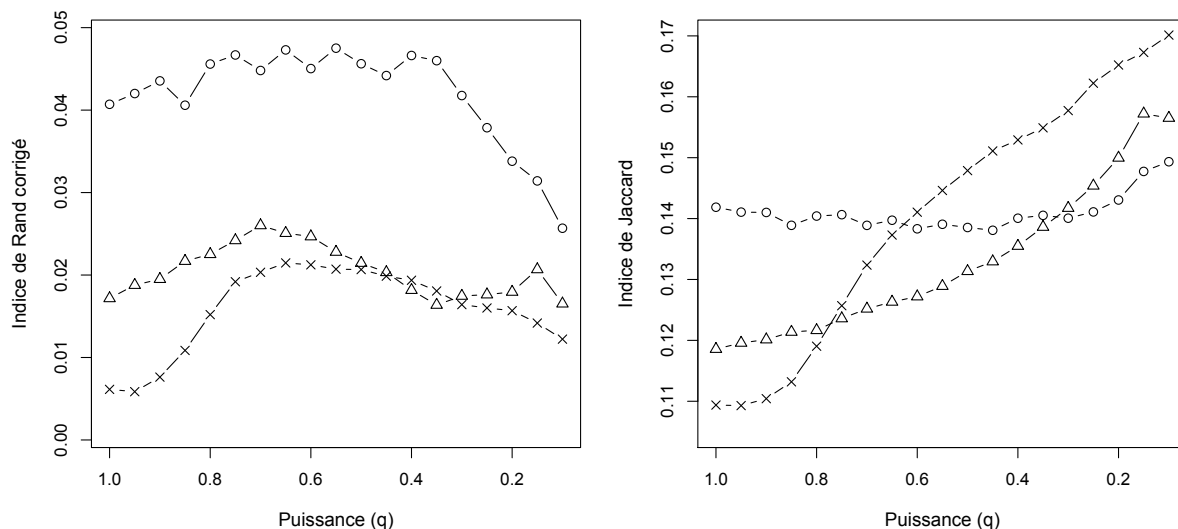
FIGURE 4.11 – « L'Orient » avec l'algorithme K-means. Indice de Rand corrigé (gauche) et de Jaccard (droite) en fonction de la puissance q . ( \circ = unigrammes, \triangle = bigrammes et \times = trigrammes). Pour rappel, q = 1 est équivalent à ne pas effectuer de transformation.
