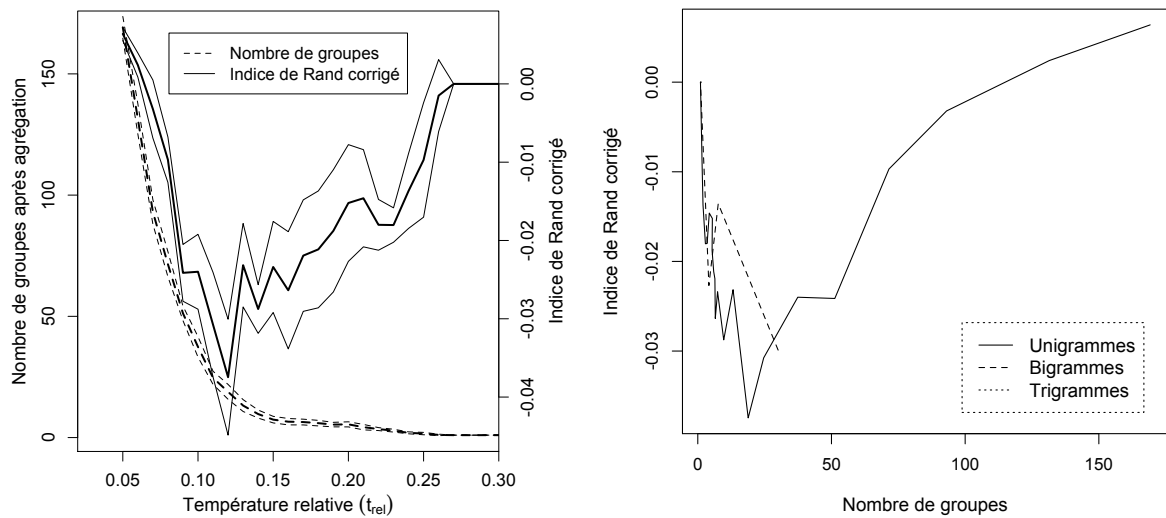
FIGURE 4.21 – « Un Fou ? » avec l’algorithme K-means flou. Moyenne (ligne épaisse) et écart-types (ligne fine) de RC et de M en fonction de t_{rel} , pour les unigrammes de CMS (gauche) et moyenne de RC en fonction de la moyenne de M pour les uni-, bi- et trigrammes de CMS (droite).
