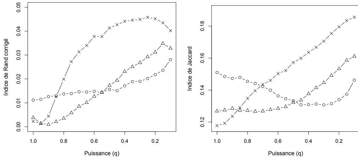
FIGURE 4.14 – « Un Fou » avec l'algorithme K-means. Indice de Rand corrigé (gauche) et de Jaccard (droite) en fonction de la puissance q . (○ = unigrammes, △ = bigrammes et × = trigrammes).
