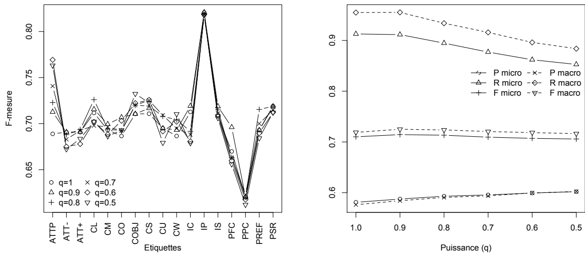
FIGURE 5.3 – Classification avec les lemmes et le critère du plus proche centroïde. F-mesure pour chaque étiquette selon la puissance q (gauche). Macro- et micro-moyennes pour la précision, le rappel et la F-mesure (droite).
