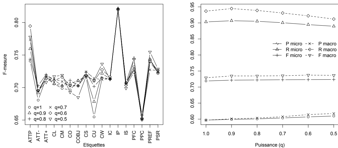
FIGURE 5.5 – Classification avec les CMS et le critère du plus proche centroïde. F-mesure pour chaque étiquette selon la puissance q (gauche). Macro- et micro-moyennes pour la précision, le rappel et la F-mesure (droite).
