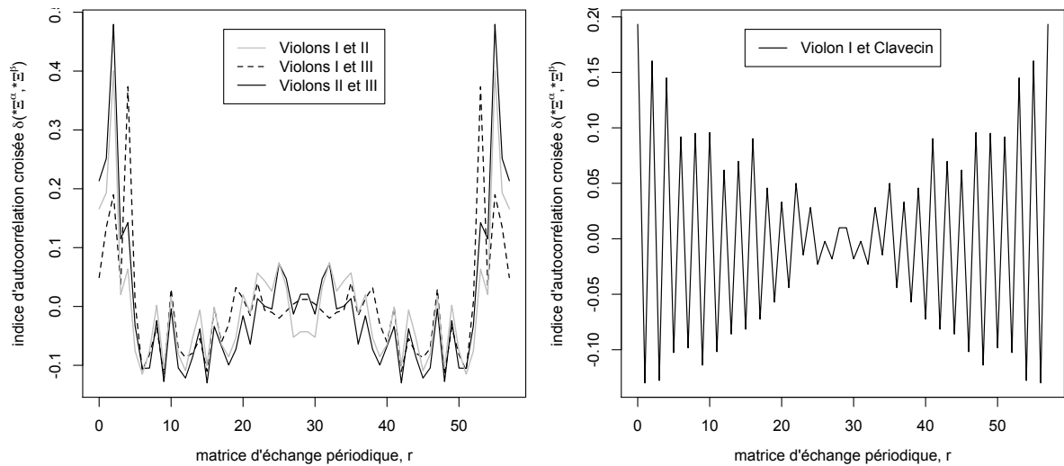
FIGURE 8.17 – Indice d'autocorrélation croisée en fonction de la distance r variant entre 0 et n pour le « Canon en ré majeur » de Pachelbel, avec \tau égal à une mesure.
