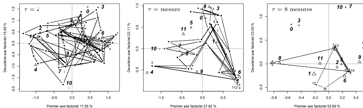
FIGURE 8.7 – AFC sur la « Mazurka en fa \sharp mineur, Op. 6, N°1 » de Chopin. Biplots avec \tau égal à une noire (gauche), à une mesure (centre) et à huit mesures (droite).
