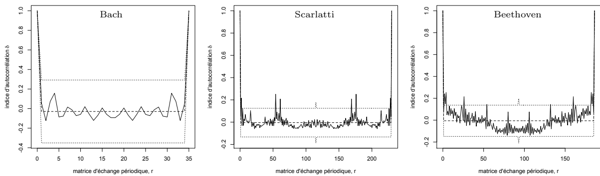
FIGURE 8.13 – Indice d'autocorrélation en fonction du décalage r variant entre 0 et n , avec \tau égal à une mesure, pour le « Prélude N°1 en do majeur, BWV 846 » de J. S. Bach (gauche), pour la « Sonate en ré majeur, Andante cantabile, L. 12 (K. 478) » de Scarlatti (centre) et pour le 3 e mouvement, « Minuetto e Trio », de la « Sonate pour piano N°1 en fa mineur, Op. 2, N°1 » de Beethoven (droite).
