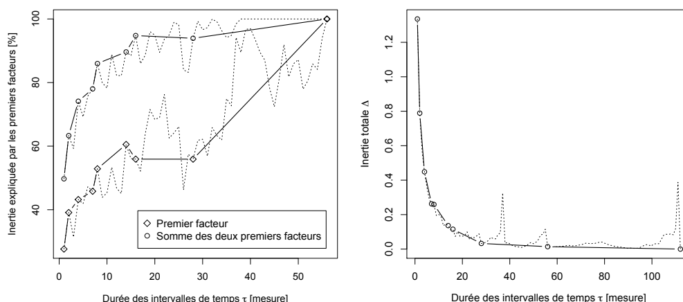
FIGURE 8.8 – AFC sur la « Mazurka en fa \sharp mineur, Op. 6, N°1 » de Chopin. Proportion d'inertie expliquée par les premiers facteurs (gauche) et inertie totale (droite) en fonction de la valeur de \tau .
