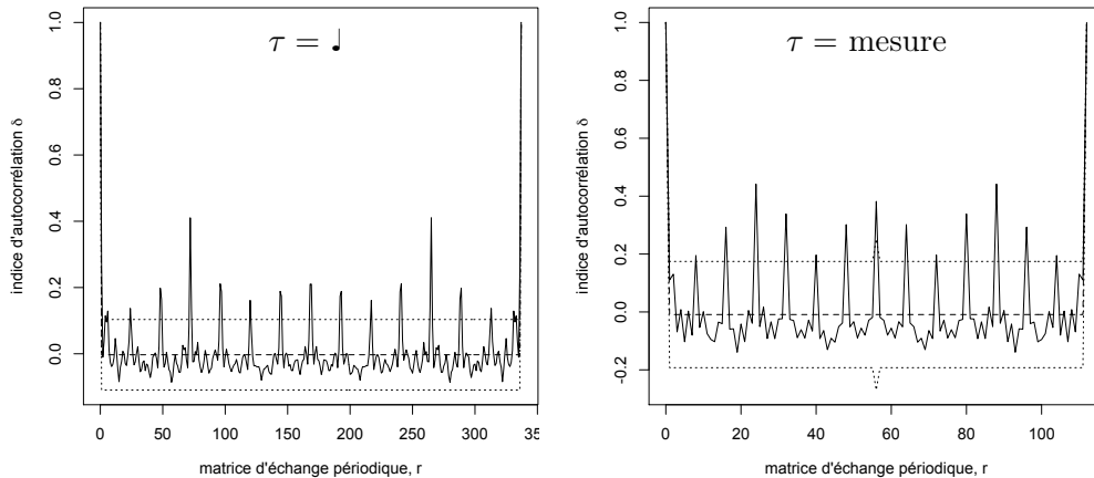
FIGURE 8.9 – Indice d'autocorrélation en fonction du décalage r variant entre 0 et n pour la « Mazurka en fa♯ mineur, Op. 6, N°1 » de Chopin, avec \tau égal à une noire (gauche) et à une mesure (droite).
