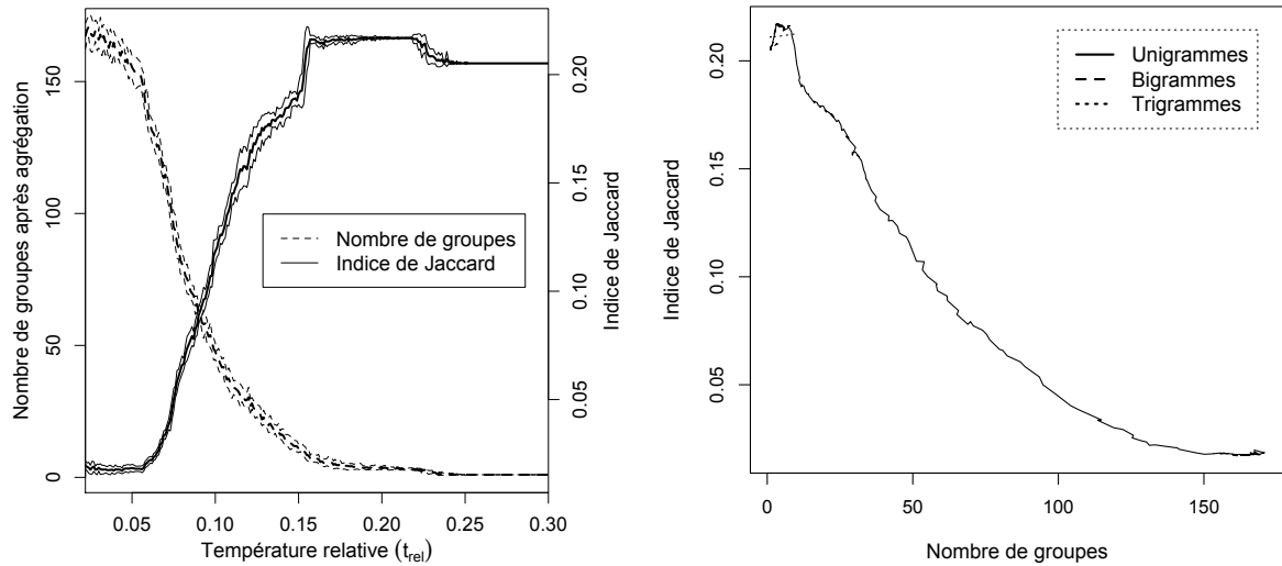
FIGURE 4.20 – « Un Fou ? » avec l’algorithme K-means flou. Moyenne (ligne épaisse) et écart-types (ligne fine) de J et de M en fonction de t_{rel} , pour les unigrammes de CMS (gauche) et moyenne de J en fonction de la moyenne de M pour les uni-, bi- et trigrammes de CMS (droite).
