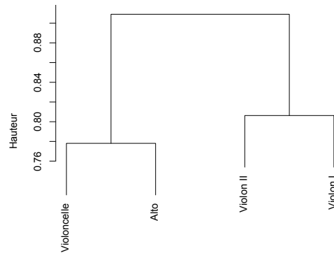
FIGURE 8.20 – Classification ascendante hiérarchique des quatre voix du 1 er mouvement du « Quatuor à cordes N°1 en fa majeur, Op. 18 N°1 » de Beethoven selon \delta(*\Xi^\alpha, *\Xi^\beta)^{(r=0)} , avec \tau égal à une mesure.
