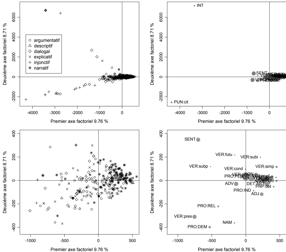
FIGURE 4.5 – AFC sur « Un Fou ? ». Coordonnées factorielles des propositions (en haut à gauche) et des unigrammes de CMS (en haut à droite). En bas : zoom sur le centre des figures du haut.
