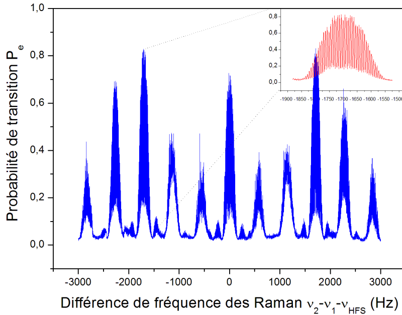
Figure 3.16 : Franges d'interférences lors d'un interféromètre de Ramsey-Raman. Paramètres : U_{\text{reseau}} = 3,9E_R , P_{IR} = 0,5 W, \tau_{\pi/2 \text{ Ram}} = 6 ms, T_{\text{Ramsey}} = 150 ms, désaccord Raman 300 GHz.
