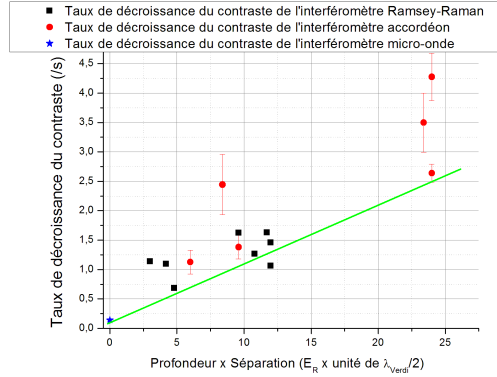
Figure 4.9 : Étude du taux de décroissance du contraste des interféromètres Ramsey-Raman (carrés noirs), accordéon (ronds rouges) et Ramsey-micro-onde (étoile bleue) en fonction de la profondeur du réseau multipliée par la séparation des paquets d'ondes atomiques (en unité de \lambda_{Verde}/2 ). Mesures réalisées pour une puissance infrarouge P_{IR} = 0,5 W et avec le faisceau CDL optimisé.
