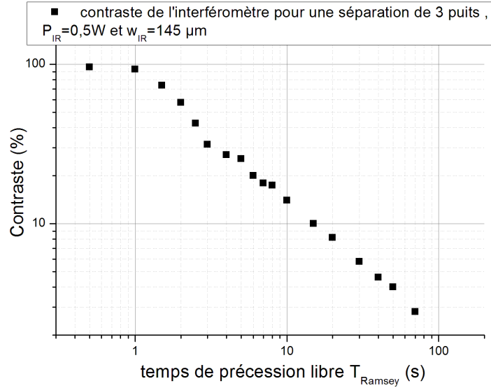
Figure 4.21 : Calcul du contraste de l'interféromètre en fonction du temps de précession libre T_{Ramsey} tracé en échelle log/log. Calcul réalisé pour P_{IR} = 0,5 W et w_{IR} = 145 \mu m, les atomes à z = 2 cm du col du laser infrarouge et \Delta m = 3 .
