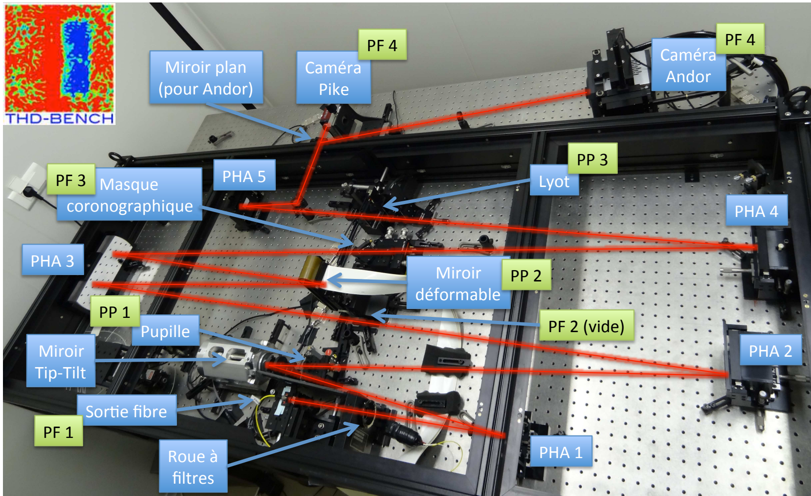
FIGURE II.1.1 – Une photo légendée du banc THD en février 2013 dans la configuration utilisée pour les analyses présentées dans Mazoyer et al. (2014a). En rouge, j’ai indiqué le chemin parcouru par le faisceau depuis la sortie de la fibre (en bas) jusqu’aux caméras (en haut), en passant par plusieurs composants, en bleu (qui seront décrits plus précisément dans cette partie) et miroirs paraboliques hors-axe (PHA). En vert enfin, j’ai indiqué la position des plans pupilles (PP) et plans focaux (PF).
