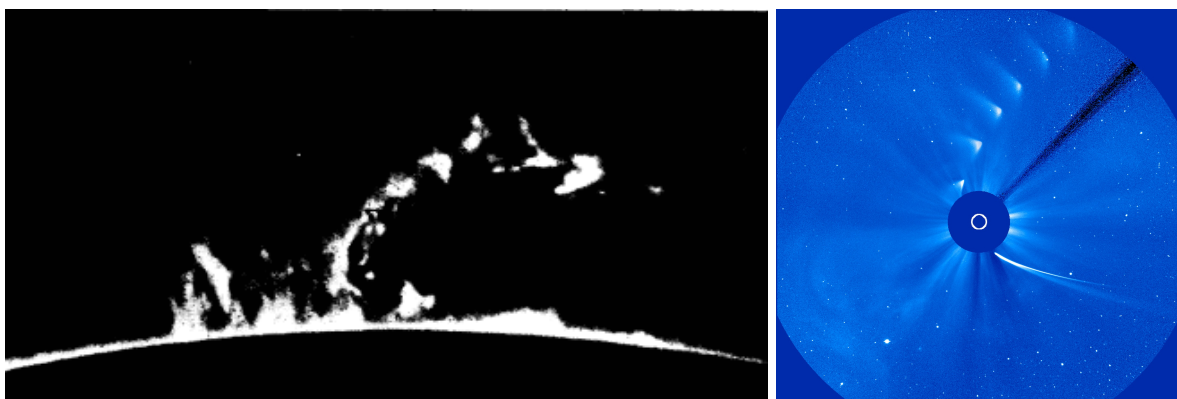
FIGURE I.3.7 – 80 ans de coronographie solaire. A gauche : observations de la couronne solaire effectuées en 1935 à l’observatoire du MIDI, tirée de Lyot (1937) . Droite : superposition de 3 jours de données du satellite SOHO montrant la désintégration de la comète ISON lors de son passage près du soleil en novembre 2013 : la trace continue en bas à droite montre son passage avant désintégration, tandis que les taches en haut sont les marqueurs de sa désintégration (crédit : ESA / NASA).
