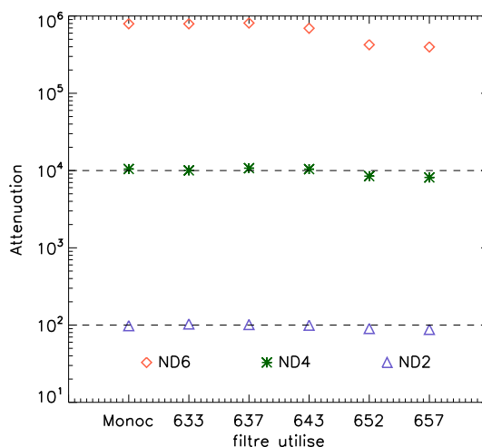
FIGURE II.1.3 – Évaluation de l'atténuation des différents filtres ND pour les bandes accessibles sur le banc
