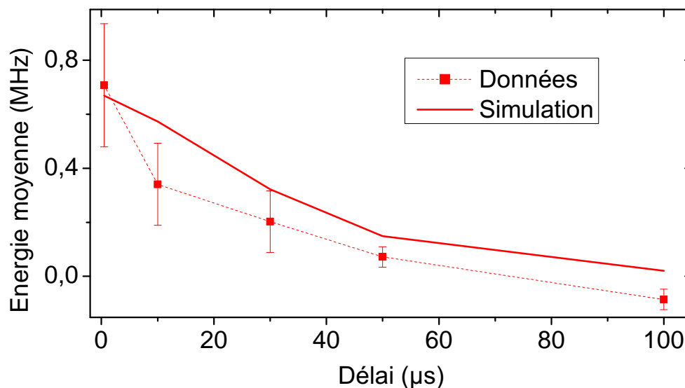
FIGURE IV.16 – Évolution de l'énergie moyenne des spectres micro-onde d'un ensemble d'atomes 60\text{S} excités à résonance, comme fonction du temps (carrés rouges), mesurée à partir des spectres de la figure IV.15. L'évolution calculée par simulation Monte Carlo est montrée en traits pleins. Le mouvement d'expansion mécanique du nuage explique bien l'évolution temporelle observée.
