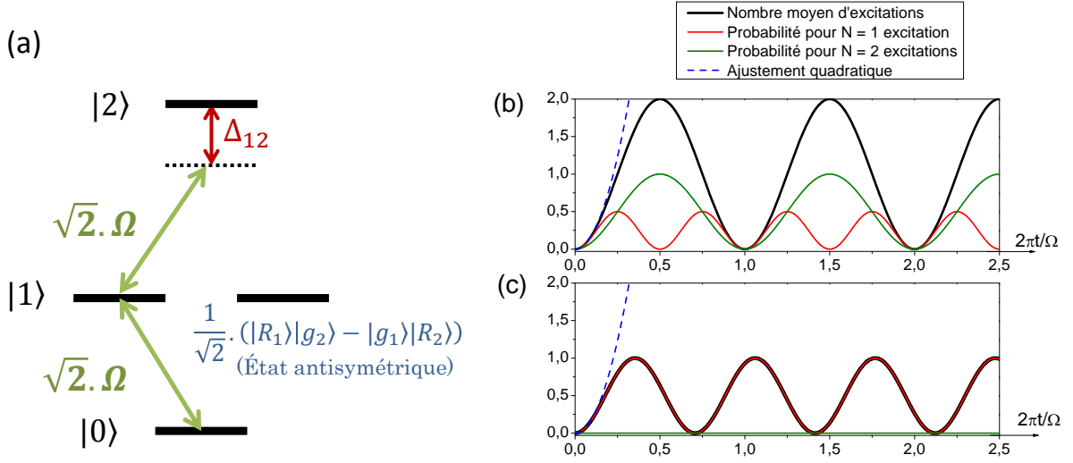
FIGURE I.8 – Solution analytique pour une paire d’atomes dans deux cas limites, le cas sans interaction et le cas à double excitation bloquée \Delta_{1,2} \gg \Omega . (a) : niveaux d’énergie du système, et le couplage entre eux induit par la lumière laser. (b) : le cas sans interaction, \Delta_{1,2} = 0 . Ce cas correspond aux oscillations de Rabi collectives avec N = 2 . La population des états |1\rangle et |2\rangle , et le nombre moyen d’excitations, sont montrés. L’ajustement quadratique sur le début de la courbe du nombre moyen d’excitations est montré en vert. (c) : le cas à forte interaction, \Delta_{1,2} \gg \Omega . Dans ce cas, le système oscille entre l’état fondamental et l’état symétrique à une excitation, avec une fréquence qui est \sqrt{2} fois plus grande que la fréquence de Rabi pour un atome unique. L’ajustement quadratique sur le début de la courbe du nombre moyen d’excitations est montré en vert, le même que pour la courbe (b). L’échelle horizontale et verticale est la même pour les deux graphiques.
