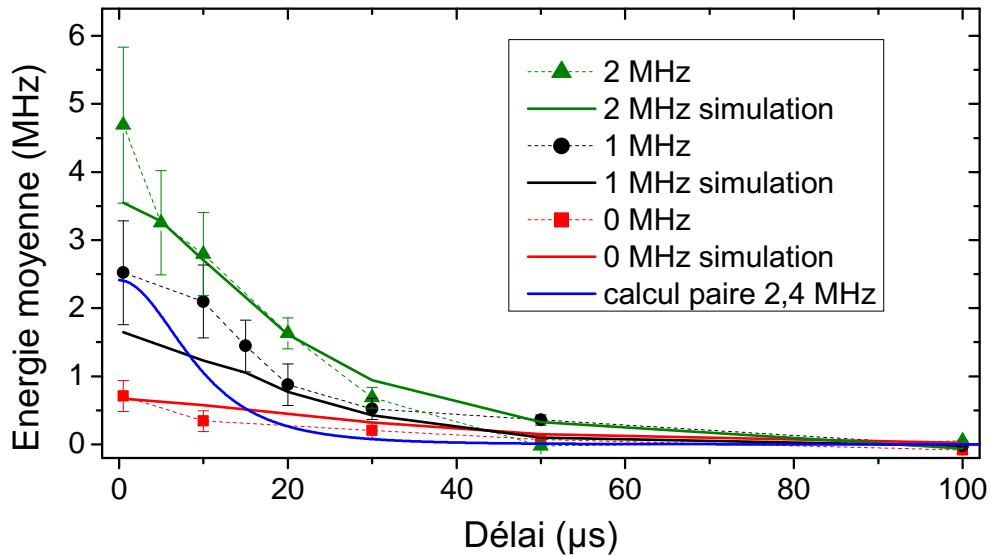
FIGURE IV.19 – Évolution de l'énergie moyenne des spectres micro-onde d'un ensemble d'atomes 60S excités à plusieurs désaccords laser, comme fonction du temps, à partir des spectres montrés dans les figures IV.15, IV.17 et IV.18. Nous voyons que le mouvement d'expansion mécanique du nuage reproduit bien l'évolution temporelle de ces spectres. En comparaison, nous montrons la courbe calculée pour une paire d'atomes avec énergie d'interaction initiale égale à 2,4 MHz. Elle évolue à une échelle de temps plus rapide que les ensembles à plusieurs atomes.
