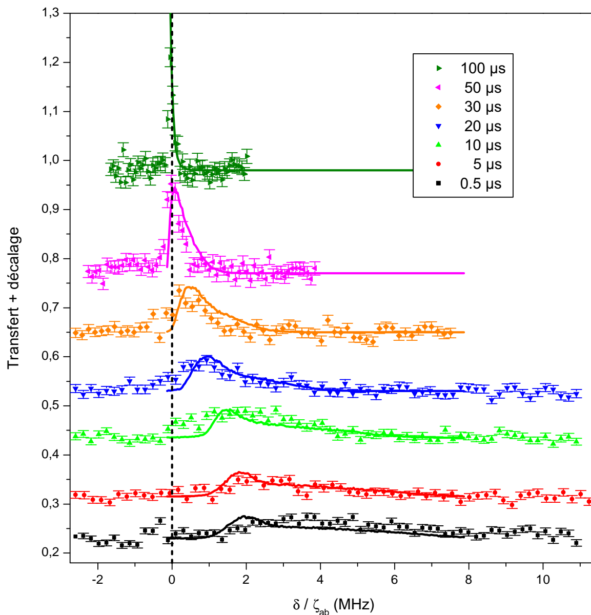
FIGURE IV.18 – Spectres micro-onde de la transition 60S \rightarrow 57S , enregistrés à des délais différents entre l’impulsion laser d’excitation et l’impulsion micro-onde (indiqués dans la légende). L’origine de l’axe vertical des spectres est décalée différemment, pour la visibilité. Le désaccord entre la somme des fréquences des deux photons laser et la transition 5S \rightarrow 60S est de 2 MHz. L’axe des abscisses est divisé par le facteur \zeta_{60S,57S} = 1,31 . L’amplitude et l’origine de l’axe vertical des simulations de Monte Carlo sont ajustées aux courbes expérimentales. Les fréquences de Rabi et durées des impulsions micro-onde utilisées pour enregistrer chaque spectre sont : 500 kHz et 1 \mu s pour les délais 0,5, 5 et 10 \mu s ; 300 kHz et 1,7 \mu s pour 20 et 30 \mu s ; 167 kHz et 3 \mu s pour 50 \mu s ; et 83 kHz et 6 \mu s pour le délai 100 \mu s.
