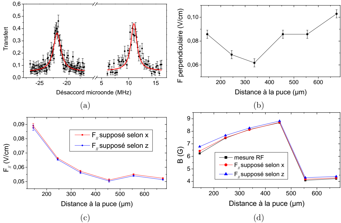
FIGURE III.14 – (a) : spectre des transitions |60S_{1/2}, m_J = 1/2\rangle \rightarrow |60P_{3/2}, m'_J\rangle , m'_J = -1/2 (à gauche) et m'_J = +3/2 (à droite), dans un piège à 455\ \mu\text{m} . Le zéro de désaccord correspond à la fréquence de la transition en absence de champ magnétique et électrique. Les courbes en rouge sont des ajustements Lorentziens, et les largeurs sont de 1,4\ \text{MHzm} limitées par l'exploration des gradients de champ électrique par l'extension spatiale du nuage, et par le bruit électrique sur les électrodes. (b) : champ électrique résiduel perpendiculaire à la puce, mesuré par création d'un champ de compensation de même module avec les électrodes I1 et I2, , comme fonction de la distance à la puce. Les barres d'erreur viennent de la discrétisation de la tension envoyée aux électrodes I1 et I2, à cause du générateur de fonctions placé au début du circuit de contrôle (schématisé dans la figure III.3). (c) : champ électrique parallèle à la puce, mesuré à partir des transitions |60S_{1/2}, m_J = 1/2\rangle \rightarrow |60P_{3/2}, m'_J\rangle , m'_J \in \{-1/2, +3/2\} , comme fonction de la distance à la puce. Les valeurs sont différentes de 2% si nous considérons que le champ électrique est parallèle à l'axe de quantification x , ou perpendiculaire à lui (selon z ), car les coefficients Stark sont différents. Les barres d'erreur proviennent de l'incertitude sur l'indétermination du centre des raies par ajustement Lorentzien. (d) : champ magnétique mesuré à partir des transitions |60S_{1/2}, m_J = 1/2\rangle \rightarrow |60P_{3/2}, m'_J\rangle , m'_J \in \{-1/2, +3/2\} , comme fonction de la distance à la puce. Le champ magnétique mesuré indépendamment par évaporation RF est aussi montré.
