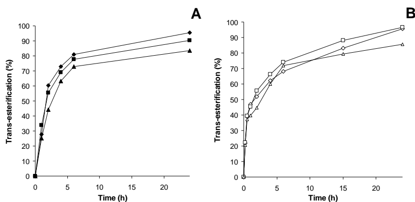
Figure 1. Pourcentage d'estérification de DHAEE à DHA-Nicotinol avec différents ratios, dans 2M2B (A) et SFS (B). (◆) 2M2B ratio 1:1, (■) 2M2B ratio 1:1.5, 2M2B ratio 1:3 (▲), (◇) SFS 1:1, (□) SFS 1:1.5 and (△) SFS 1:3. Temperature 60°C. N435 (7% w/w).
