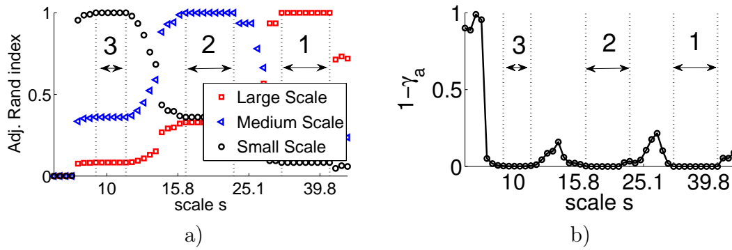
FIGURE 2.18: Résultat de l'algorithme comparé à la mesure de stabilité proposée. Les trois intervalles où les partitions théoriques sont retrouvées sont reportés sur la figure d'instabilité : ils correspondent très bien aux intervalles où l'instabilité 1 - \gamma_a est minimale.
