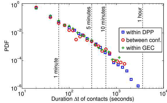
FIGURE 3.8: Distributions cumulées de la durée de contacts intra-DPP, intra-GEC, et entre les deux conférences du jeu de données SLC.
