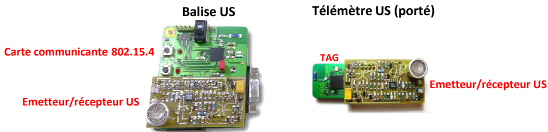
Figure 34. Balise US et Télémètre US
