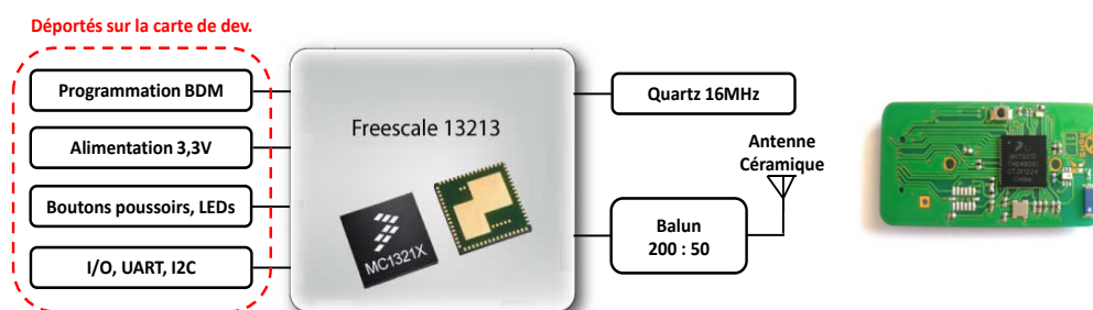
Figure 3. Schéma bloc du dispositif Balise
