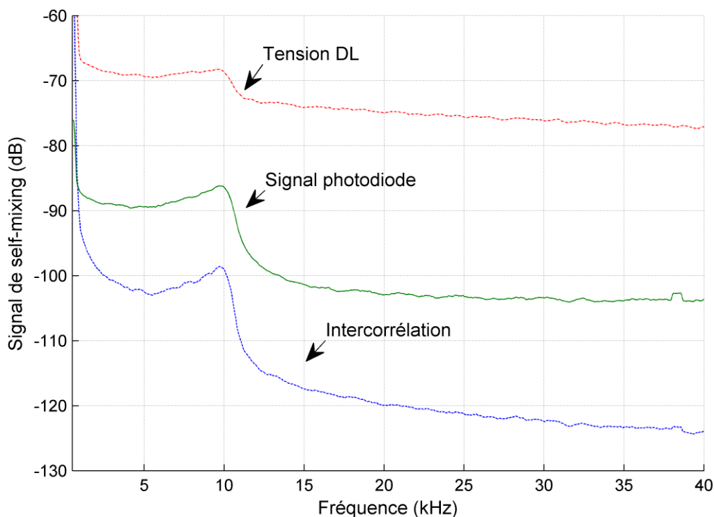
Figure IV-7. Signaux de self-mixing mesurés aux bornes de la jonction laser (DL), à la sortie de la photodiode (PD), et l'intercorrélation des ces deux signaux. Le signal d'intercorrélation présente un meilleur rapport signal sur bruit.
