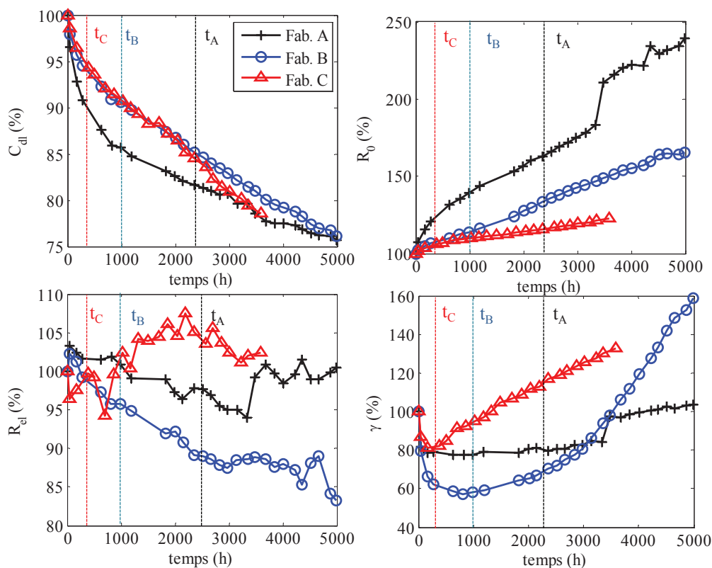
Figure 3.6 Evolution relative des paramètres du modèle CPE pour un vieillissement CS 60°C 2.8V
