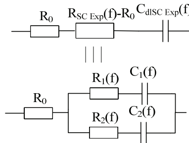
Figure 2.33 Equivalence entre les résultats expérimentaux d'impédance et le modèle multipore deux branches dans la zone correspondant à l'effet combiné des branches 1 et 2
