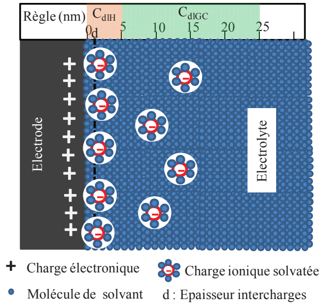
Figure 1.8 Principe du stockage d'énergie en double couche électrique
