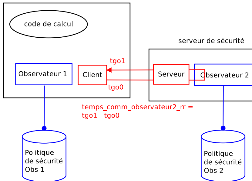
FIGURE 4.8 – Prise du temps avec une communication et un observateur en mode distant
