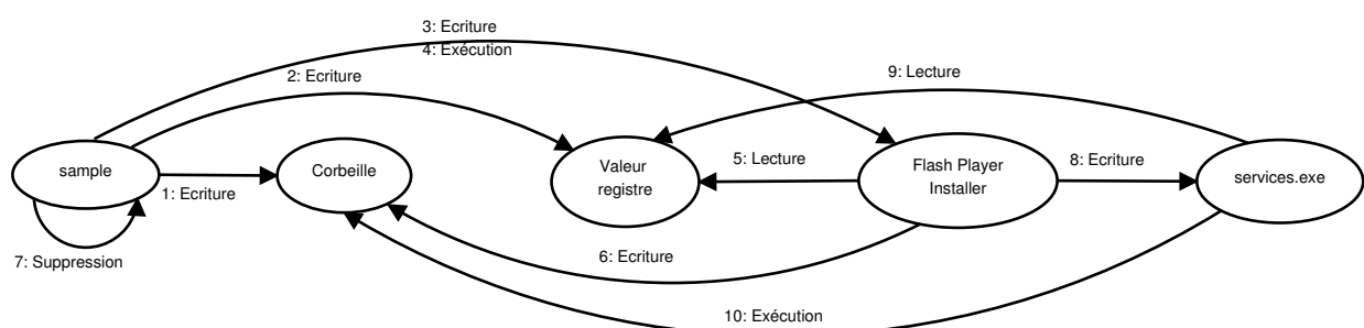
FIGURE 5.12 – Automate complet des interactions réalisées par le logiciel malveillant
