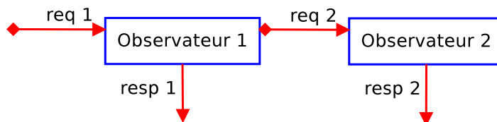
FIGURE 3.15 – Mode d'association : continuation
