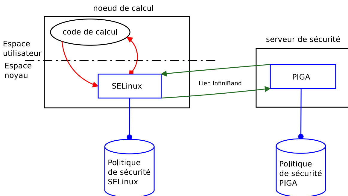
FIGURE 4.12 – Architecture décentralisée
