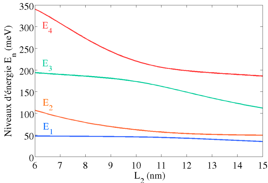
FIGURE I.4 – Variations des énergies propres de la structure 10 \text{ nm}/2 \text{ nm}/L_2 d' \text{In}_{0.53}\text{Ga}_{0.43}\text{As}/\text{GaAs}_{0.51}\text{Sb}_{0.49} en fonction de la largeur de puits L_2 . Les paramètres de calcul sont : m_w^* = 0.043m_0 , m_b^* = 0.045m_0 , V_b = 360 \text{ meV} et F_{\text{bias}} = 12 \text{ kV.cm}^{-1} [54]. Ces courbes ont été obtenues en résolvant l'équation (I.5) par dichotomie numérique où le champ \vec{F}_{\text{bias}} a été discrétisé le long de l'axe z .
