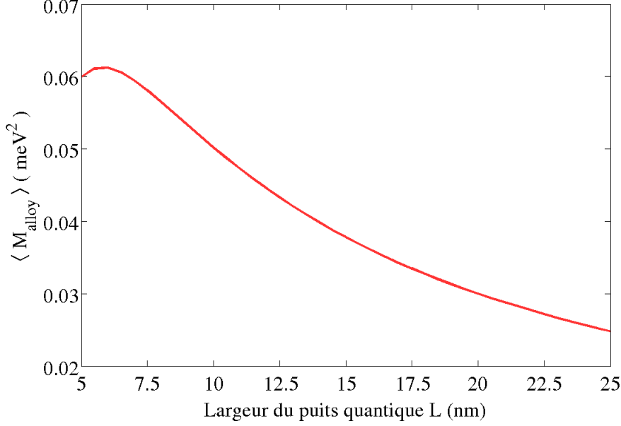
FIGURE I.10 – Evolution de l'élément de matrice effectif \langle M_{\text{alloy}} \rangle = \langle |\langle 1\vec{k} | V_{\text{alloy}} | 2\vec{k}' \rangle|^2 \rangle_{av} en fonction de la longueur L_z de la structure de simple puits d' \text{In}_{0.53}\text{Ga}_{0.43}\text{As}/\text{GaAs}_{0.51}\text{Sb}_{0.49} . Les paramètres de calcul sont : m_w^* = 0.043m_0 , m_b^* = 0.045m_0 , V_b = 360 meV et \Delta V = 0.6 eV.
