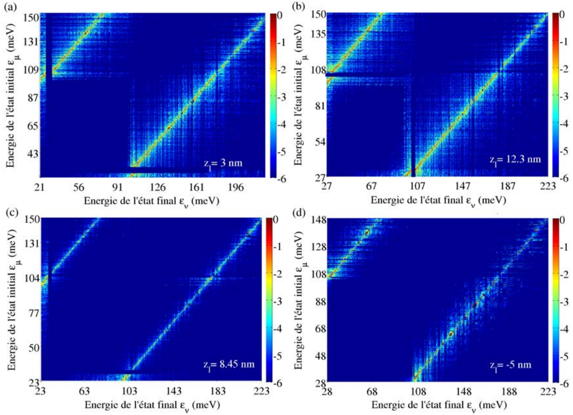
FIGURE III.20 – Élément dipolaire normalisé pour l'ensemble des transitions \varepsilon_\nu - \varepsilon_\mu (logarithme décimale de l'élément dipolaire). Le terme de désordre V_{\text{dis}} dans H correspond au potentiel coulombien écranté créé par la distribution de 8 impuretés ionisées sur le plan z_l = 3 nm (a), z_l = 12.3 nm (b), z_l = 8.45 nm (c) et z_l = -5 nm (d). n_e = 2.17 \times 10^{10} \text{ cm}^{-2} . E_2 - E_1 = 73.8 meV. Moyenne sur 50 configurations aléatoires d'impuretés.
