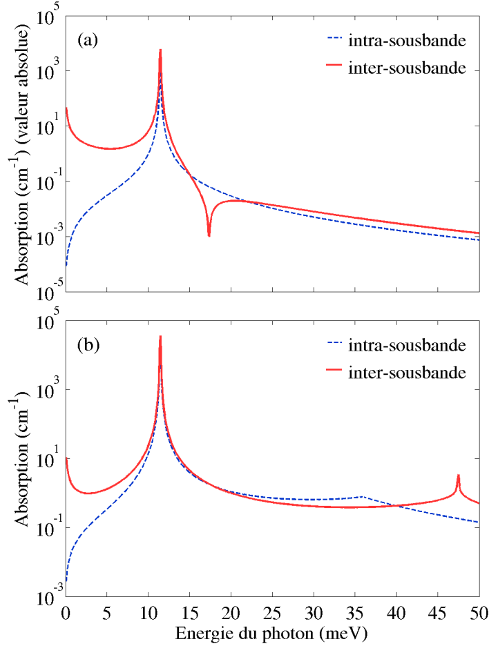
FIGURE II.16 – Coefficient d'absorption par porteurs libres \alpha_{nm}^{LO,abs/em} assistée par (a) l'absorption et (b) l'émission de phonon LO. Les contributions associées aux transitions intra-sousbande |2\vec{k}\rangle \rightarrow |2\vec{k}'\rangle (pointillé bleu) et inter-sousbande |2\vec{k}\rangle \rightarrow |3\vec{k}'\rangle (continu rouge) sont représentées. T_L = 100 K et T = 150 K. E_3 - E_2 = 11.46 meV. n_e = 2.17 \times 10^{10} cm⁻². \hbar\omega_{LO} = 36 meV. Structure 23/2/12 nm de GaAs/Al 0.15 GaAs 0.85 .
