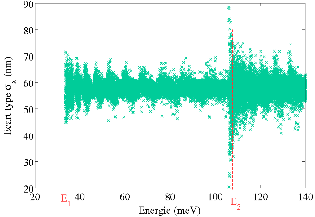
FIGURE III.6 – Ecart-type \sigma_x des états propres du Hamiltonien H en fonction de leur énergie, en présence de défauts d'interface. E_1 = 33.67 meV et E_2 = 107.46 meV. \sigma = 3.6 nm, f_{\text{def}} = 0.30 et h_{\text{def}} = 2.83 Å. N_{\text{att}} = N_{\text{rep}} = N_{\text{def}}/2 . Moyenne effectuée sur 50 configurations aléatoires de défauts.
