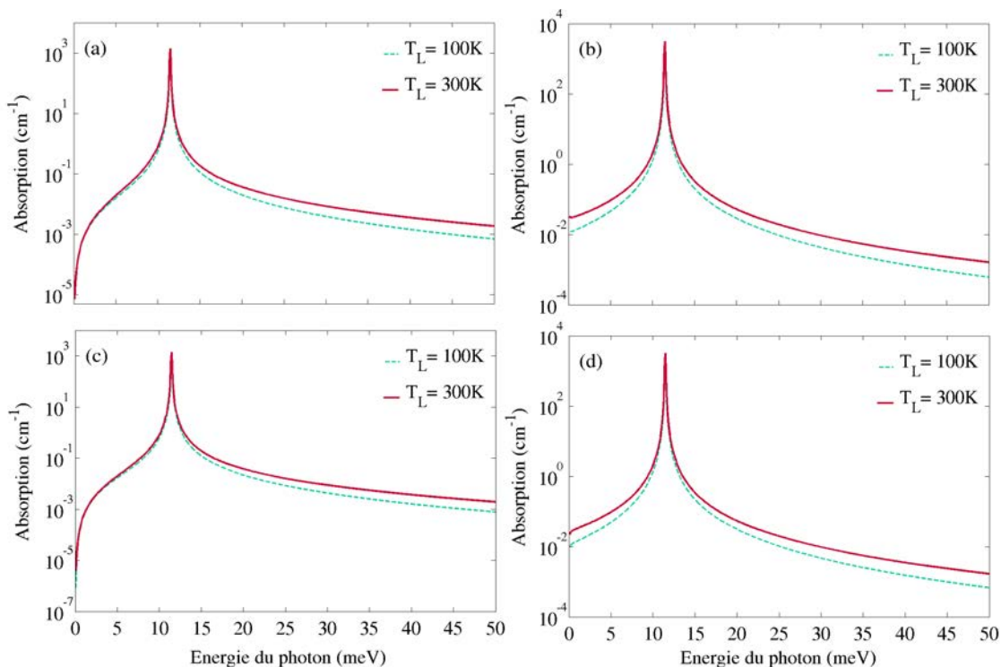
FIGURE II.17 – Coefficient d’absorption par porteurs libres assistée par l’interaction électron-phonon LA. Panneaux supérieurs : absorption d’un phonon LA ( \alpha_{nm}^{LAabs} ). Les graphes a et b correspondent aux transitions intra-sousbande |2\vec{k}\rangle \rightarrow |2\vec{k}'\rangle et inter-sousbande |2\vec{k}\rangle \rightarrow |3\vec{k}'\rangle respectivement. Panneaux inférieurs : émission d’un phonon LA ( \alpha_{nm}^{LAemi} ). Les graphes c et d correspondent aux transitions intra- et inter-sousbande respectivement. Deux températures du réseau sont considérées : T_L = 100 K (pointillé vert) et T_L = 300 K (continu rouge). E_3 - E_2 = 11.46 meV. n_e = 2.17 \times 10^{10} cm ^{-2} . D = 8.6 eV. T = T_L . Structure 23/2/12 nm de GaAs/Al _{0.15} GaAs _{0.85} .
