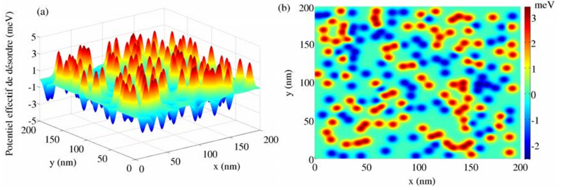
FIGURE I.12 – Allure du potentiel effectif de désordre d'interface (moyenné sur l'état \chi_1^2 ) dans les plan (x, y) de la structure 9/2/3 nm de GaAs/Al 0.25 GaAs 0.75 . Les paramètres de désordre sont : \sigma = 3.6 nm, h_{\text{def}} = 2.83 Å et f_{\text{def}} = 0.30 , soit 172 défauts répartis sur l'interface z_0 = 9 nm ( N_{\text{att}} = N_{\text{rep}} = 86 ). (a) Représentation du potentiel sur le plan des couches (x, y) . (b) Cartographie de la surface désordonnée (vue à deux dimensions).
