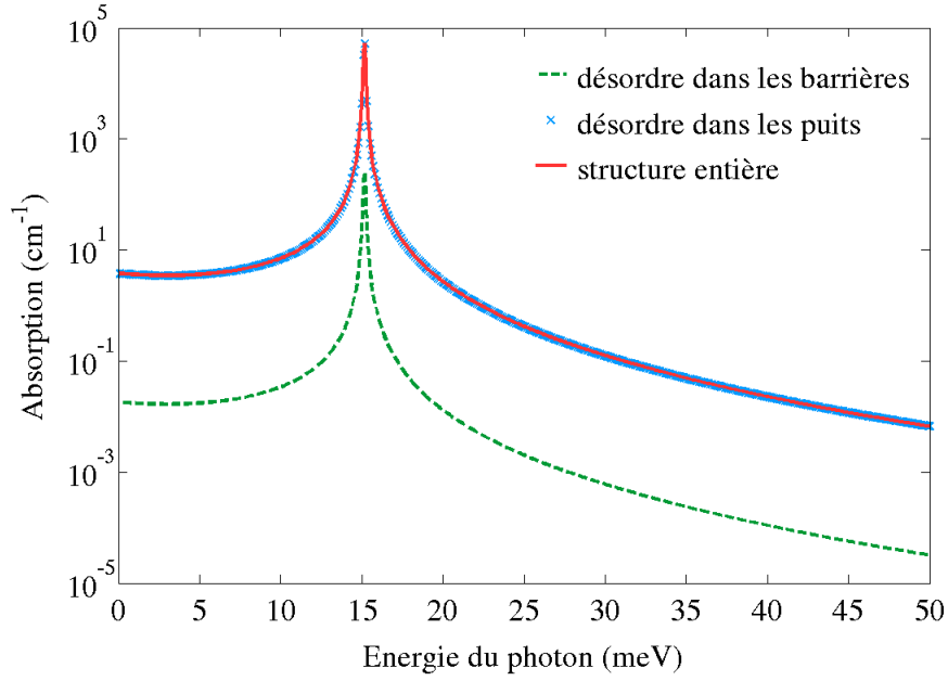
FIGURE II.11 – Coefficient d'absorption par porteurs libres médiate par le désordre d'alliage ( \alpha_{\text{alloy}} ) associé aux transitions obliques intra-sousbande |2\vec{k}\rangle \rightarrow |2\vec{k}'\rangle pour une localisation du désordre d'alliage dans les barrières (pointillé vert), les puits quantiques (croix bleues) ou dans la structure entière 23/2/12 nm d' \text{In}_{0.53}\text{Ga}_{0.43}\text{As}/\text{GaAs}_{0.51}\text{Sb}_{0.49} (continu rouge). E_3 - E_2 = 11.46 meV. n_e = 2.17 \times 10^{10} \text{cm}^{-2} . \Delta V = 0.6 eV et x_{\text{alloy}} = 0.53 dans InGaAs et x_{\text{alloy}} = 0.51 dans GaAsSb. T = 100 K.
