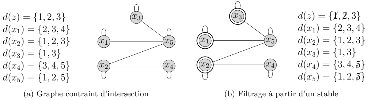
FIGURE 9.4 – Utilisation de \text{AMNV}\langle G_{\mathcal{CI}} | \text{MD} | \mathcal{R}_{1,2} \rangle sur notre exemple
