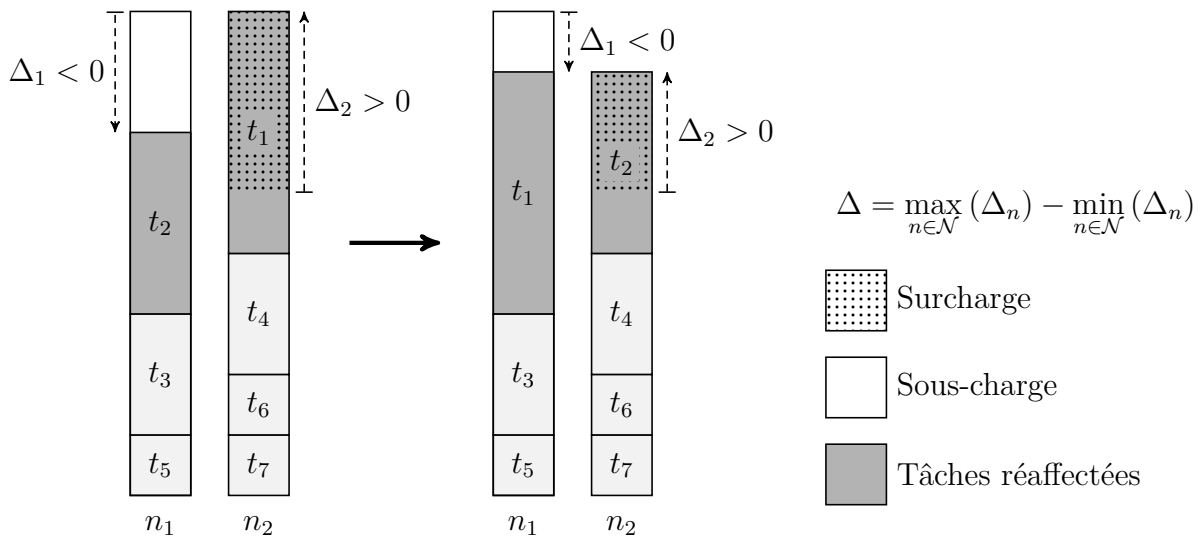
FIGURE 4.5 – Réduction de l'inégalité via H_\Delta , cas d'un échange
