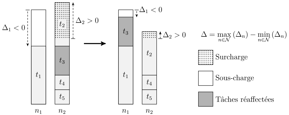
FIGURE 4.4 – Réduction de l'inégalité via H_\Delta , cas d'une insertion
