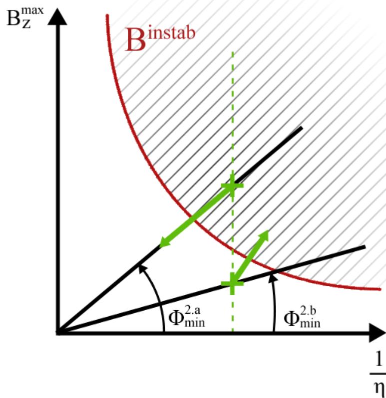
Figure A.5 – Schéma du critère d'activation périodique de la zone morte. Les cas 2.a et 2.b sont représentés par deux croix vertes. La ligne pointillée verte rappelle que la résistivité est identique dans les cas 2.a et 2.b. Les flèches vertes indiquent les parties de l'espace des paramètres qui seront explorées prochainement. Les hachures repèrent l'espace des paramètres qui conduisent à l'activation partielle de la zone morte.
