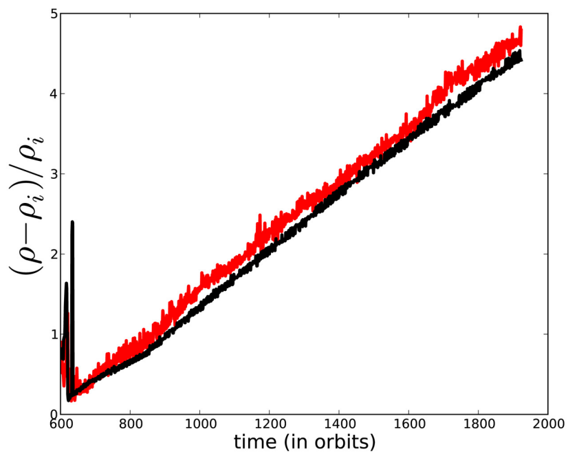
Figure 6.1 – Évolution de la perturbation relative de densité dans la simulation MHD du modèle IE-FIX (en rouge) et dans la simulation 2D du modèle visqueux de la région du bord interne de la zone morte (en noir). Dans la simulation MHD, la formation de vortex a été inhibée en réduisant l'ouverture angulaire du domaine. Aucun vortex ne se forme dans la simulation 2D avant l'introduction d'une perturbation au maximum de densité.
