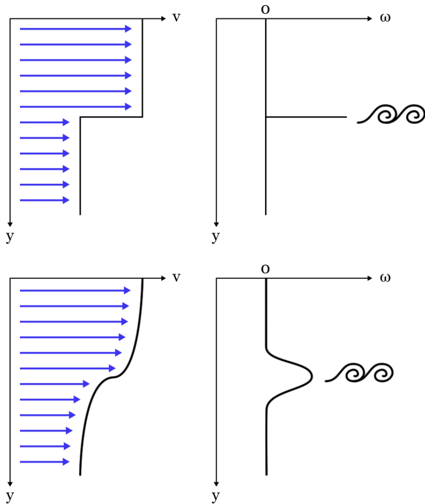
Figure 3.5 – Profils transverses de vitesse (à gauche) et de vorticit  (  droite) de deux  coulements bi-dimensionnels instables. Sur le profil de vitesse j'ai repr sent  quelques vecteurs vitesse par des fl ches bleues.
