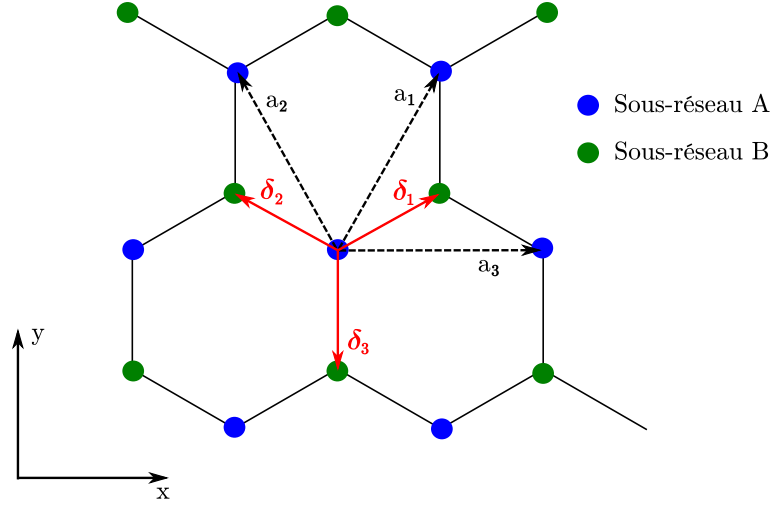
FIGURE 3.1 – Représentation schématique du réseau hexagonal du graphène. Les atomes des deux sous-réseaux A et B apparaissent en bleu et en vert respectivement. Les vecteurs \delta_1 , \delta_2 et \delta_3 entre atomes voisins (flèches rouges) et \mathbf{a}_1 , \mathbf{a}_2 , \mathbf{a}_3 entre seconds voisins (flèches en tirets noirs) sont également représentés.
