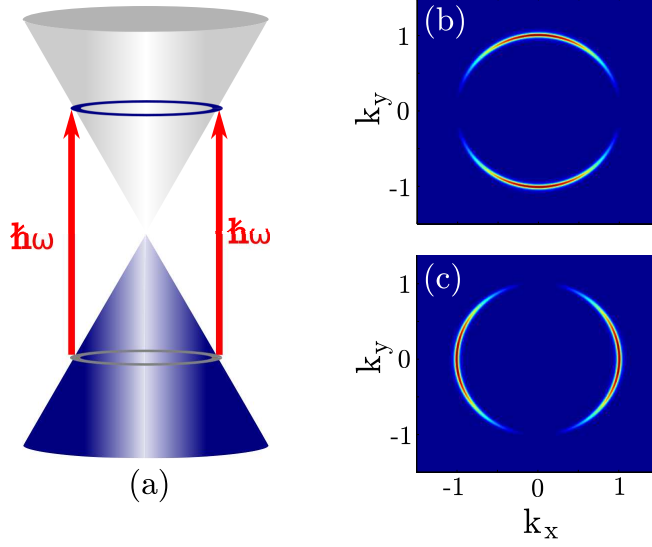
FIGURE 3.3 – (a) Représentation schématique de la structure de bande d'une monocouche de graphène. Les transitions interbandes provoquées par l'absorption d'un photon à l'énergie \hbar\omega sont représentées par des flèches rouges verticales. A droite, la population d'électrons photogénérés dans la bande de conduction est représentée en fonction du vecteur d'onde normalisée, pour une excitation polarisée suivant l'axe 0x (b) ou suivant l'axe 0y (c).
