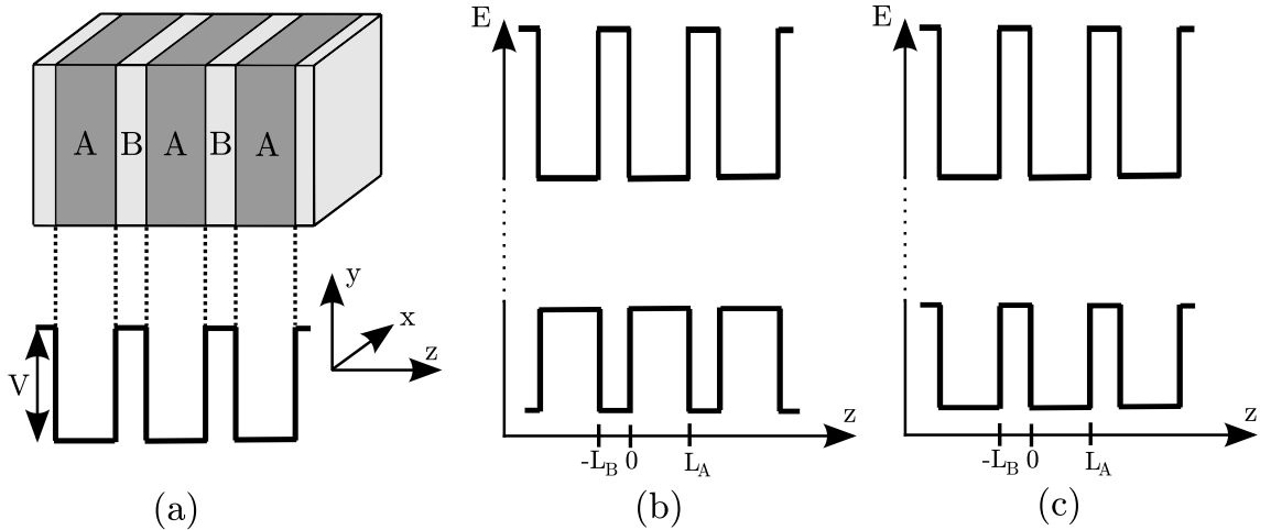
FIGURE 1.2 – (a) Représentation schématique d'un super-réseau de puits quantiques.
