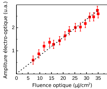
FIGURE 3.8 – Amplitude de la réponse électro-optique (unités arbitraires) en fonction de la fluence incidente sur le graphène. Les carrés rouges correspondent aux valeurs mesurées et les barres d'erreur à l'écart-type associé aux fluctuations de bruit. Les tirets noirs soulignent la dépendance linéaire.
