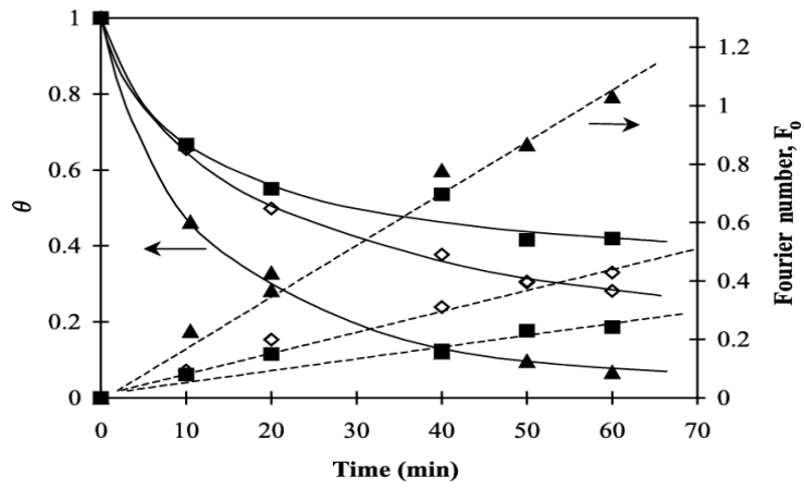
Figure 15. Estimation du coefficient de diffusion à partir de la pente du nombre de fourrier en fonction du temps (Chassagne-Bercès et al., 2009)
