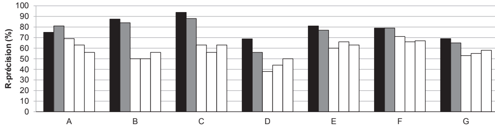
FIG. 4.16 – Distribution des R-précisions avec différentes indexations calculées pour chaque classe de versions. Les lettres en abscisse désignent la classe considérée (voir Tableau 3.2). Noir : aucune indexation, gris : indexation par la répétition majeure, blanc : de gauche à droite, indexations par les méthodes arbitraires I1, I2 et I3.
