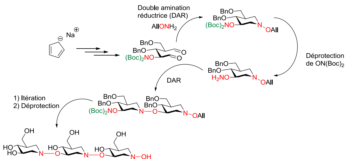
Schéma 144 : Récapitulatif de la stratégie de synthèse d'un trimère de type hydroxylamine.
