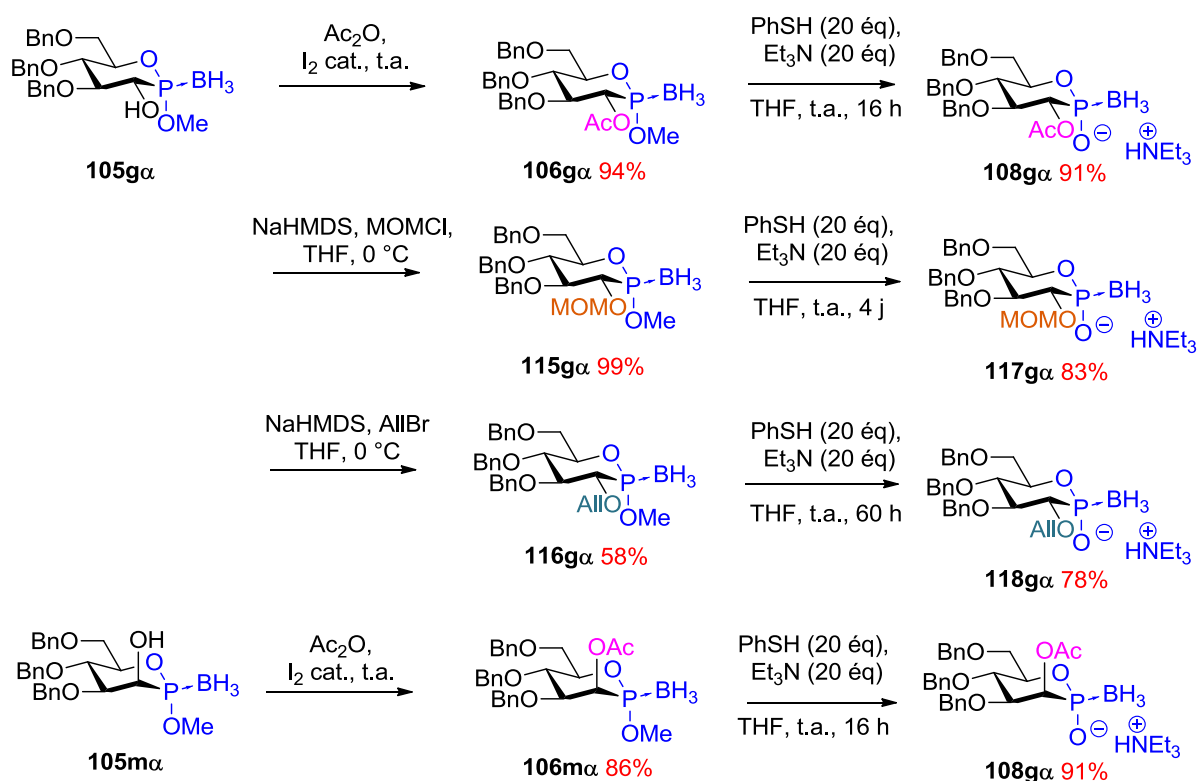
Schéma 58 : Protection de l'alcool libre des phosphonite-boranes 105g \alpha et 105m \alpha et déméthylation
