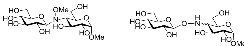
Figure 7 : Glycomimétiques développés par Dumy
