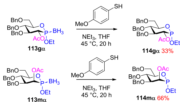
Schéma 57 : Déboration des phosphonite-boranes 113g \alpha et 113m \alpha
