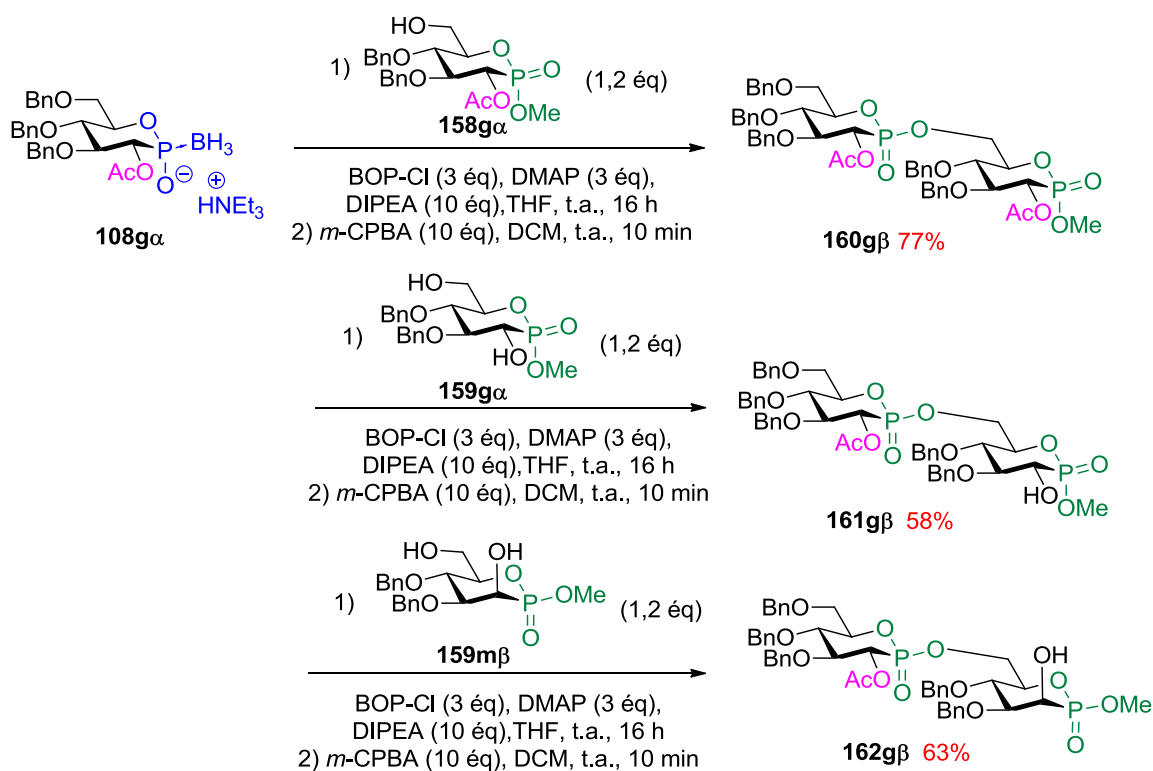
Schéma 73 : Formation de dimères phosphonite-phosphonate
