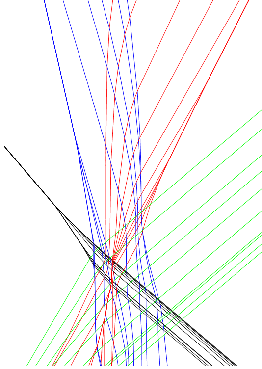
FIGURE 1.6 – Un exemple de trajectoire de la dynamique des particules collantes multitype. Les positions des particules sont représentées en abscisses, et le temps est en ordonnée. Chaque couleur est associée à un type de particule. Les particules de même type se collent aux collisions, et les collisions entre amas de types différents peuvent modifier les vitesses des amas, voire faire éclater ceux-ci.
