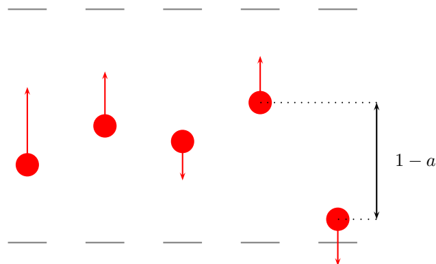
FIGURE 1.2 – Le modèle d’échange complet pour N = 5 molécules. L’écart entre les positions des molécules 4 et 5 a atteint la valeur 1 - a , ces molécules doivent donc échanger leur vitesse.
