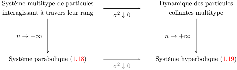
FIGURE 1.5 – Liens formels entre système multitype de particules interagissant à travers leur rang, dynamique des particules collantes et systèmes paraboliques (1.18) et hyperboliques (1.19). Dans ce manuscrit, on ne s’intéresse pas directement à la flèche grisée.
