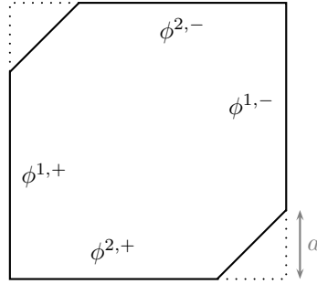
FIGURE 1.3 – La table de billard \bar{\Omega} . Les densités de mise à jour associées à chaque mur droit sont indiquées.
