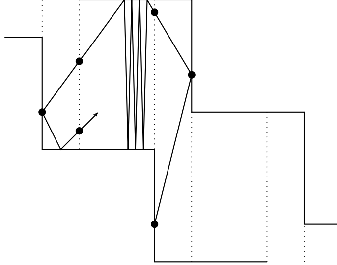
FIGURE 1.4 – Un exemple de trajectoire dépliée. Les bandes sont délimitées par le prolongement de tous les murs verticaux, ce prolongement est marqué en pointillés. Le temps mis par la boule pour traverser une bande est donné par la largeur de la bande divisée par la composante normale (par rapport au bord de la bande) de la vitesse au moment où la boule se trouve sur le bord de la bande. Tant que la boule reste dans une bande, ses composantes horizontale et verticale évoluent indépendamment. La chaîne (Y_n)_{n \geq 0} est obtenue en repliant les configurations obtenues à chaque instant d'observation sur le processus déplié.
