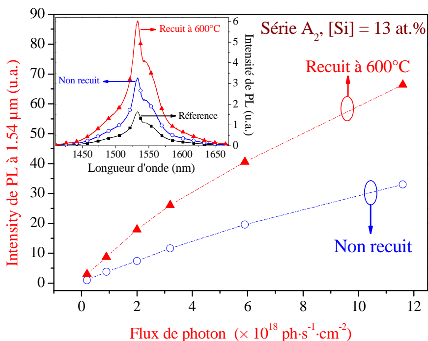
Figure IV.13 : Evolution typique de I_{PL}^{Er} à 1,54 µm en fonction de flux de photons pour un échantillon de la série A 2 , avant et après recuit à 600°C. La longueur d'onde d'excitation est 476 nm. L'encart reporte les spectres de l'émission de l'Er pour les mêmes échantillons à un flux de 6 \times 10^{19} ph·s -1 ·cm -2 .
