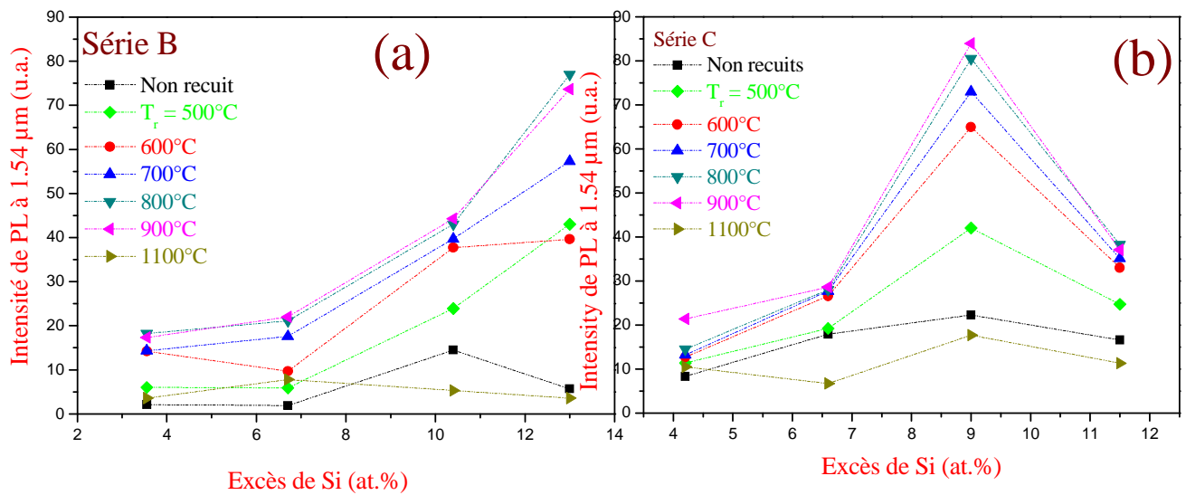
Figure IV. 14 : Evolution de I_{PL}^{Er} à 1,54 \mu\text{m} en fonction de l'excès de Si avant et après recuit à différentes T_s . (a) Série B. (b) Série C. Le flux des photons incidents sur l'échantillon est de 8 \times 10^{18} \text{ ph} \cdot \text{s}^{-1} \cdot \text{cm}^{-2} .
