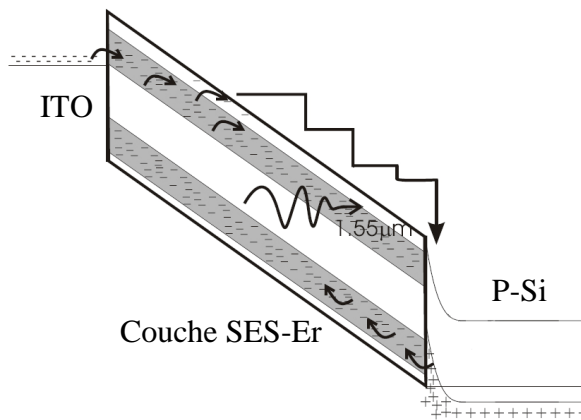
Figure I.22 : Diagramme d'énergie dans la structure ITO/SiO x :Er/p-Si pour une forte tension.
