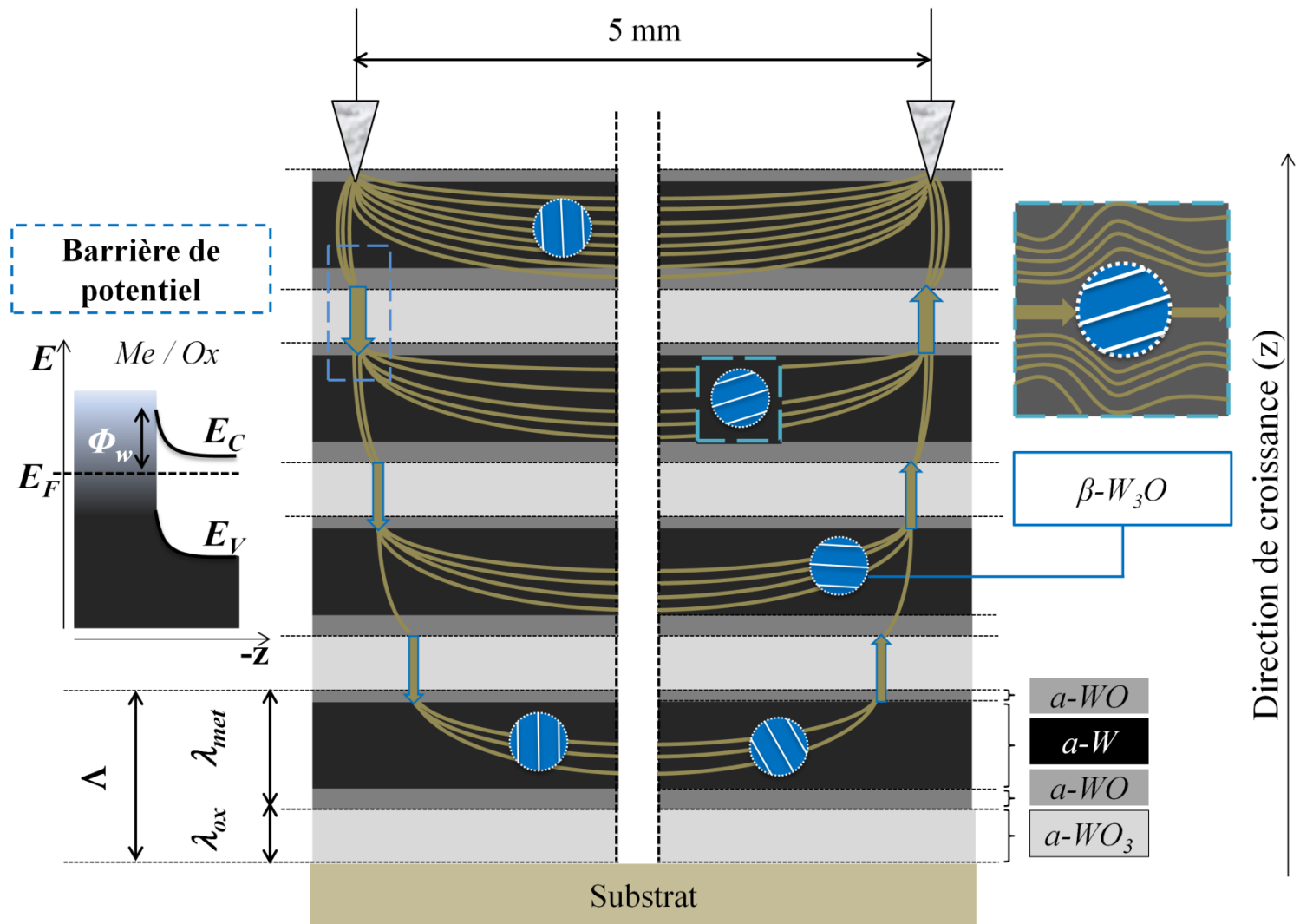
Figure V.12. Proposition d'un modèle de conduction dans les structures multicouches périodiques WO/W/WO/WO 3 .
