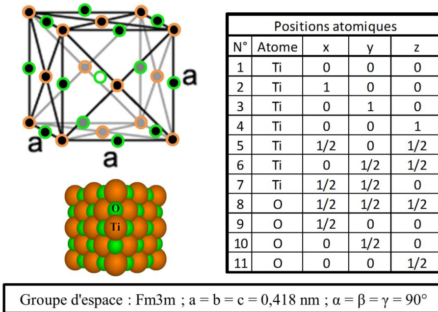
Figure II.12. Schéma de la structure cubique à faces centrées cfc-TiO avec l'annotation des positions atomiques du titane et de l'oxygène, ainsi qu'une projection 3D sur 4 mailles dans la direction \langle 111 \rangle .
