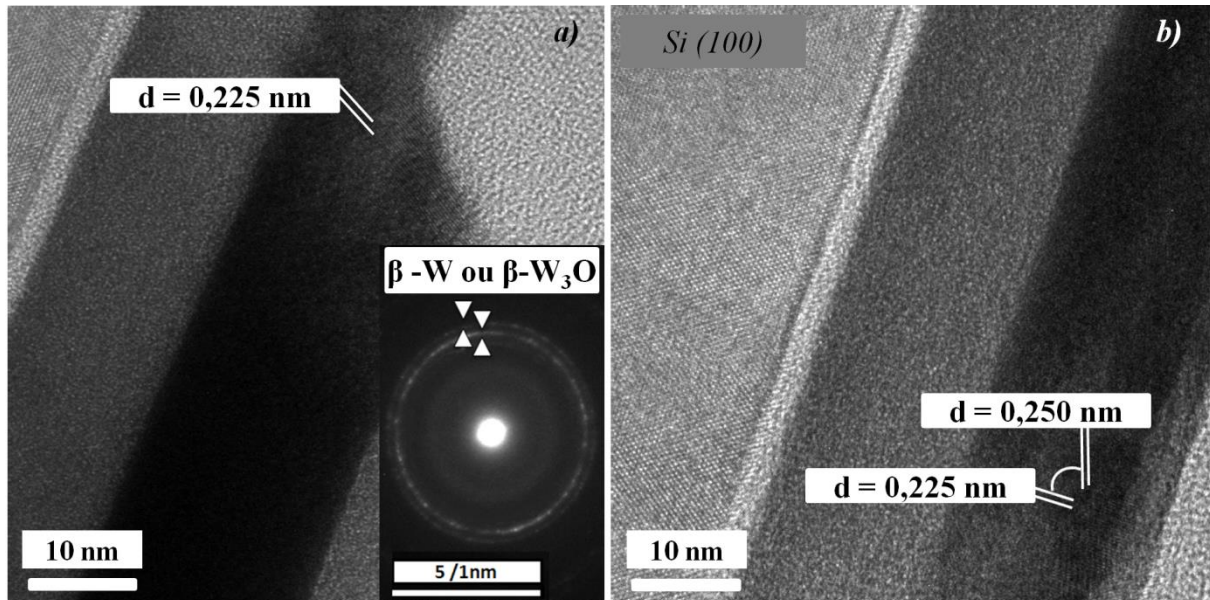
Figure IV.8. a) Image METHR de l'échantillon \text{WO}_x/\text{W} de période \Lambda = 26,5 \text{ nm} avec insertion d'un cliché de diffraction SAED, pointant les distances d_{200} et d_{210} des phases de structure cristalline identique \beta\text{-W} et/ou \beta\text{-W}_3\text{O} . Cet exemple est représentatif de l'ensemble des échantillons \text{WO}_x/\text{W} pour \lambda_{\text{met}} > 9,0 \text{ nm} , b) Un axe de zone [001] de la phase \beta\text{-W} ou \beta\text{-W}_3\text{O} avec les distances interplanaires d_{200} et d_{210} .
