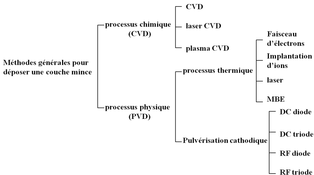
Figure I.2. Méthodes générales de dépôt de couches minces sous vide.
