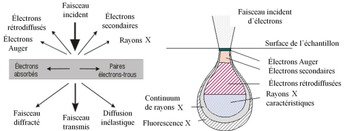
Figure. III.7. Interaction électron-matière pour un échantillon mince à gauche et pour un échantillon épais à droite.
