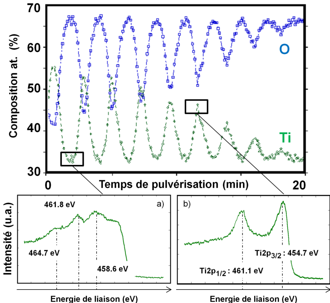
Figure IV.3. Profil XPS obtenu pour un échantillon \text{TiO}_x/\text{Ti} de période \Lambda = 34,6 nm avec les fenêtres énergétiques de la raie \text{Ti}_{2p} de spectres XPS sélectionnées a) sur une couche métallique et b) sur une couche oxydée.
