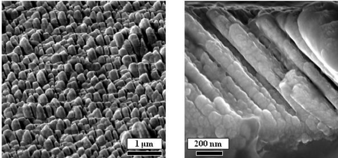
Figure VI.4. Clichés MEB en mode électrons secondaires a) de la surface et b) de la tranche d'un échantillon colonnaire W/WO x .
