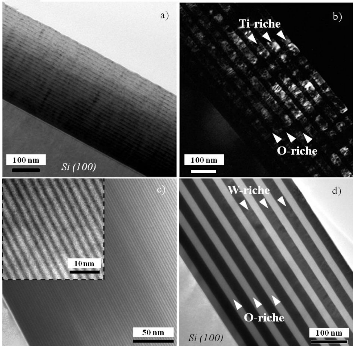
Figure IV.2. Images MET d'une coupe transverse des films multicouches déposés sur substrat Si(100) pour différentes périodes \Lambda a) TiO_x/Ti b) TiO_x/Ti en mode d'imagerie champ sombre et c)-d) WO_x/W .
