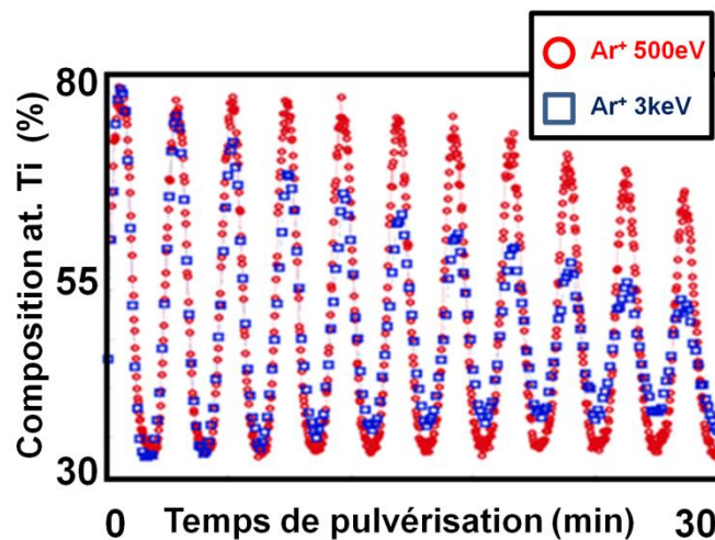
Figure IV.4. Influence de la baisse de l'énergie des ions \text{Ar}^+ primaires avec le même angle d'émergence des électrons sur la résolution en profondeur d'un profil XPS pour un échantillon titane de période \Lambda = 40,0 \text{ nm} .
