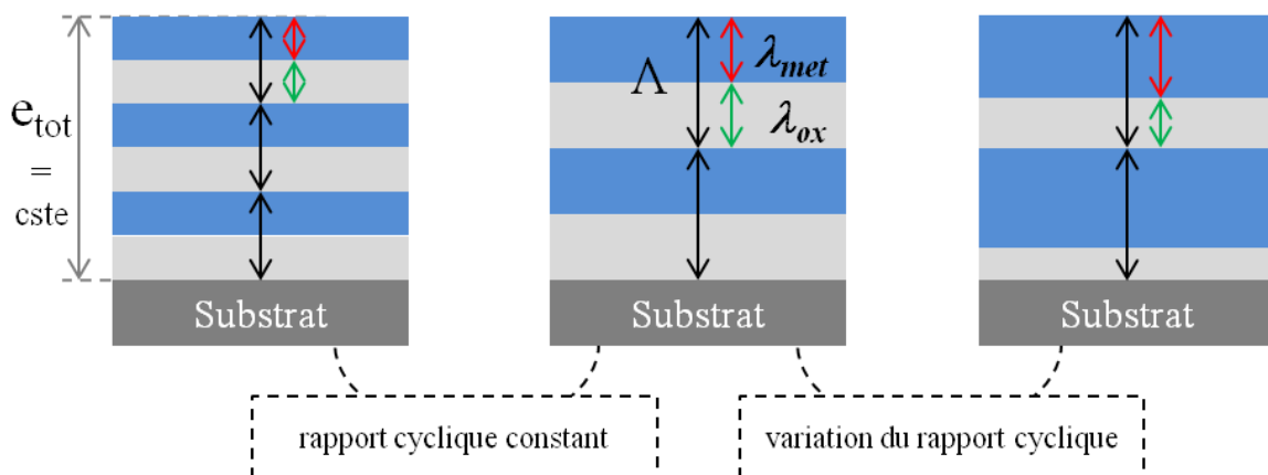
Figure III.5. Schéma représentant la variation des paramètres caractéristiques des multicouches périodiques en fonction du rapport cyclique t_{on}/T .
