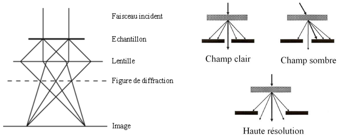
Figure III.9. Principe de fonctionnement du microscope électronique en transmission.
