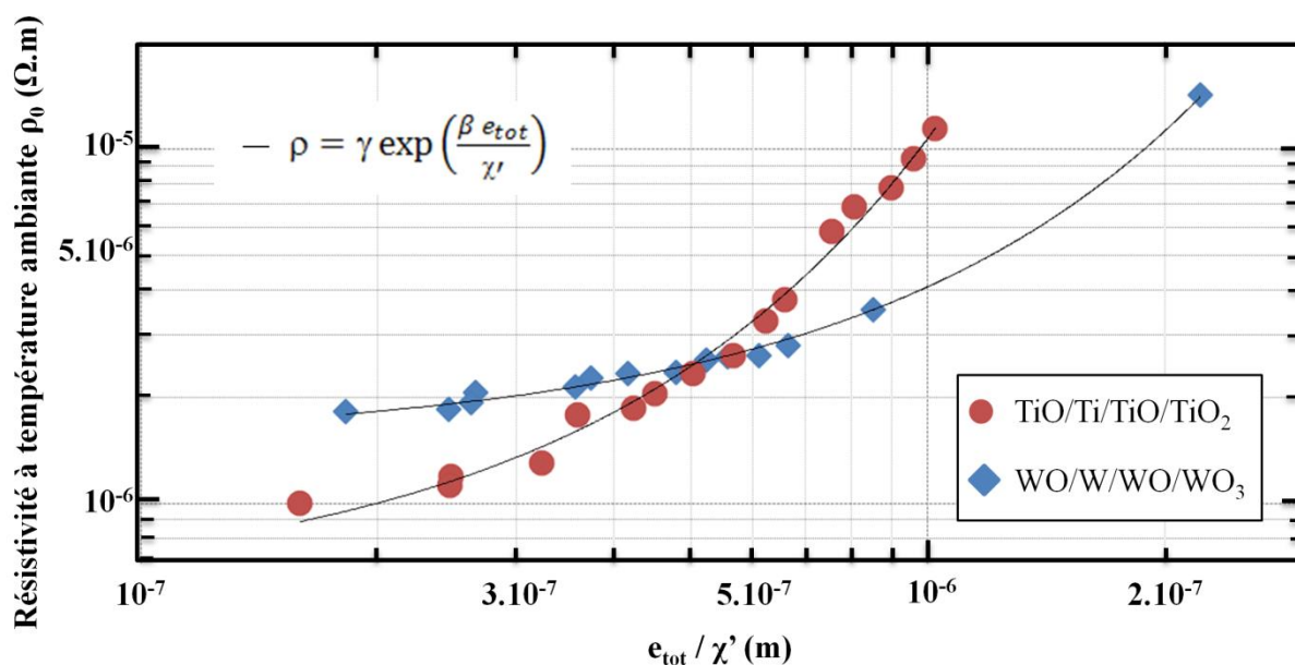
Figure V.9. Résistivité à température ambiante \rho_0 en fonction du rapport e_{tot}/\chi' pour les systèmes métal/oxyde produits par RGPP.
