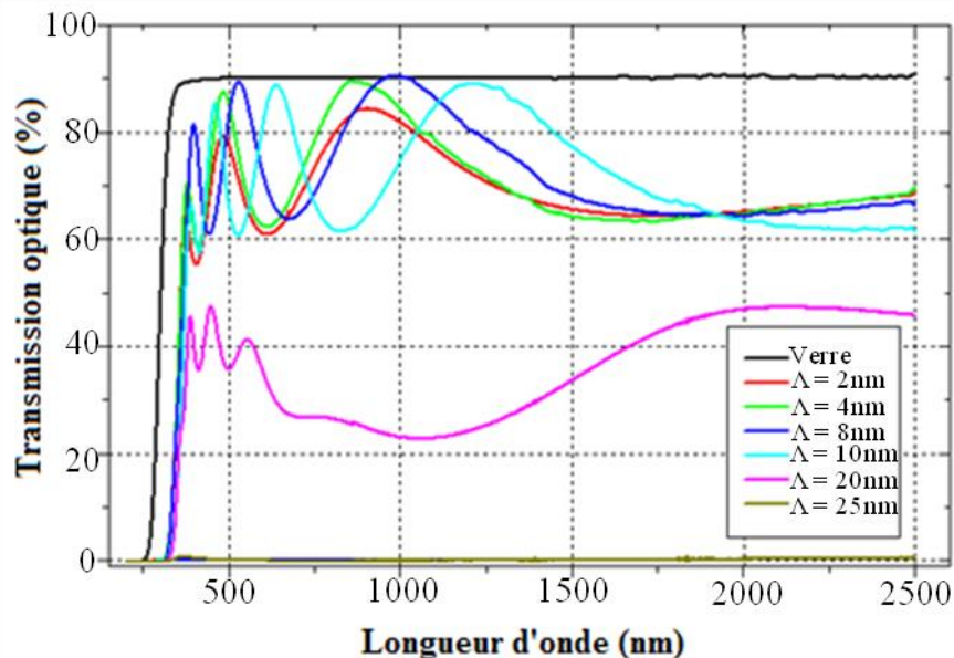
Figure II.6. Transmission optique des multicouches Ti/TiO_x de période \Lambda < 25 nm élaborées par le procédé de gaz réactif pulsé (RGPP).
