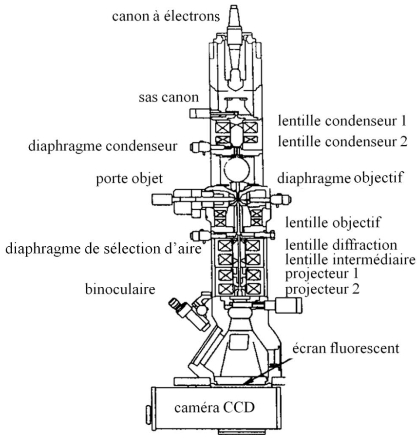
Figure III.8. Schéma d'un dispositif MET.
