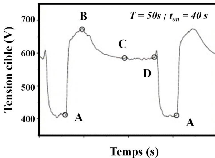
Figure III.15. Evolution du potentiel de la cible au cours d'une période d'impulsion d'oxygène pour des échantillons à base de tungstène [21].
