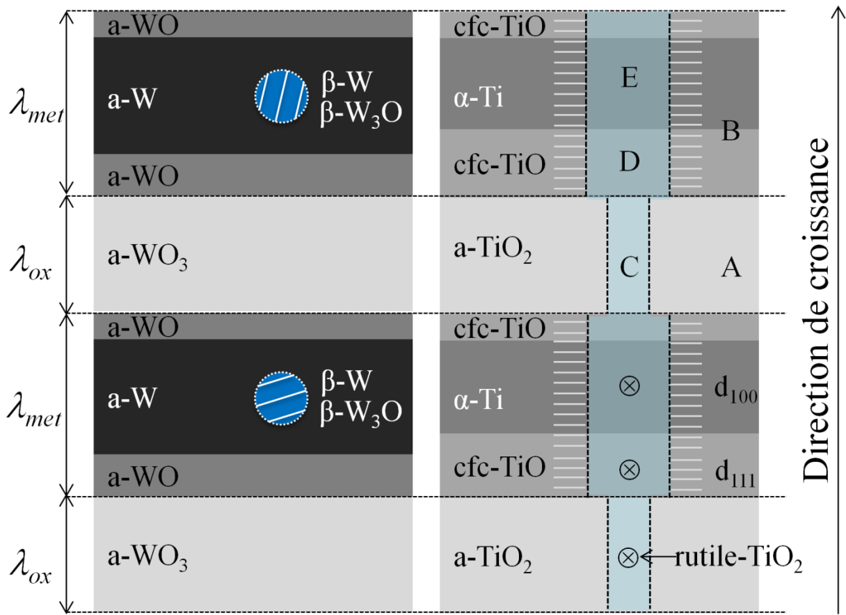
Figure IV.26. Comparaison des modèles de structures des deux systèmes avec \otimes les axes de zones des colonnes cristallines des multicouches à base de titane. En bleu, les cristallites ou réseaux cristallins, en blanc les distances interréticulaires.
