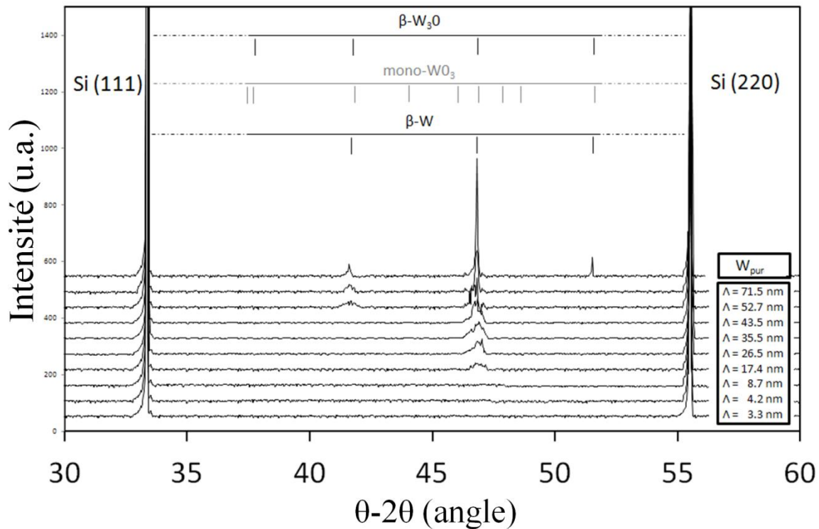
Figure IV.7. Diffractogrammes DRX de l'échantillon de référence W_{pur} et des dépôts de WO_3/W pour des périodes allant de 3,3 à 71,5 nm.
