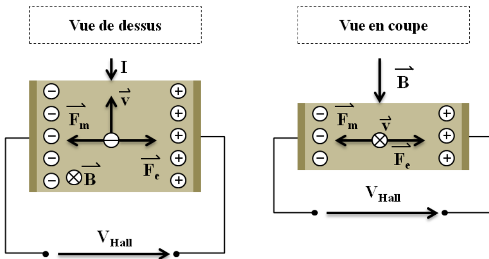
Figure III.14. Tension de Hall et force de Lorentz.
