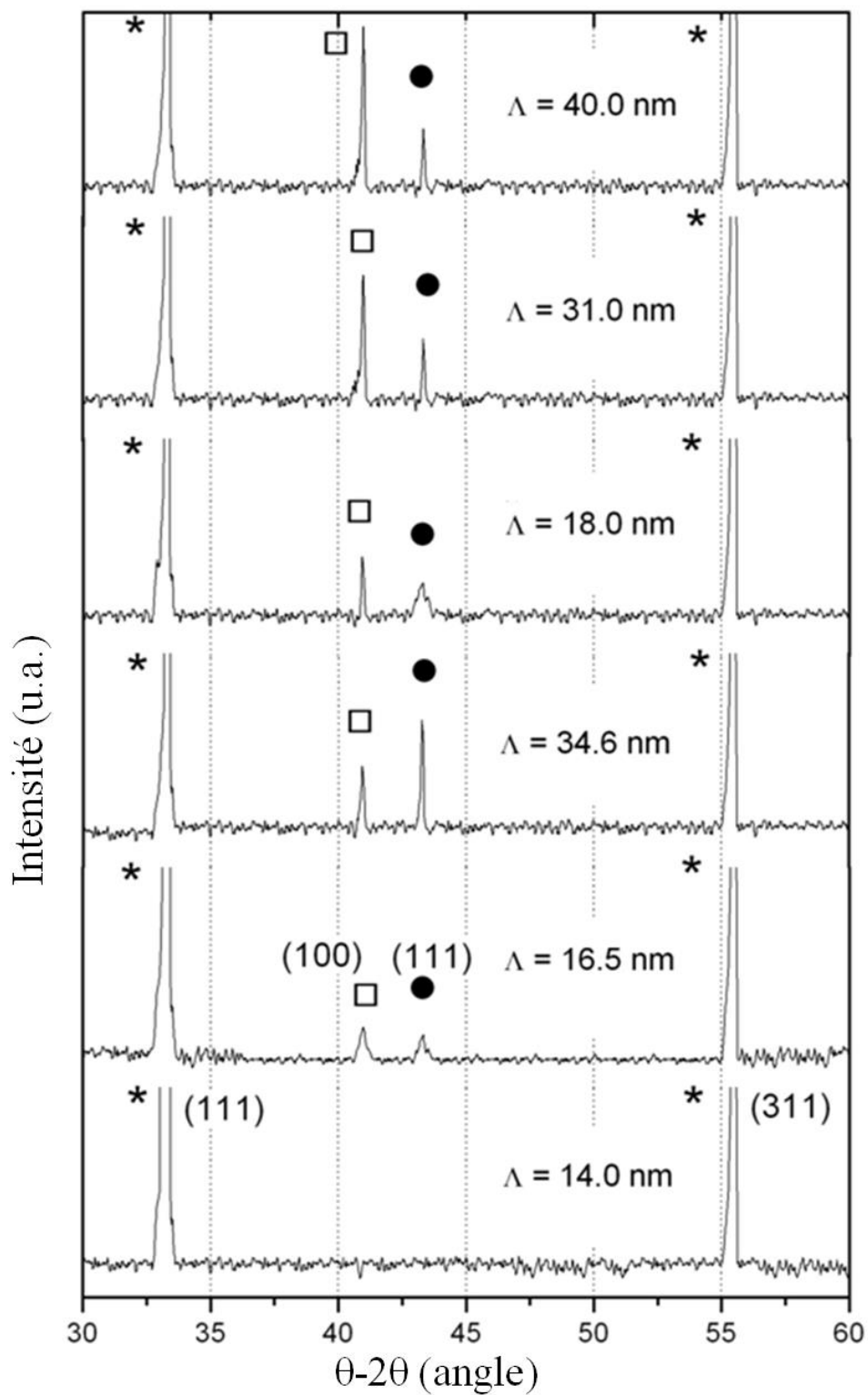
Figure IV.11. Diffractogrammes de rayons X des échantillons \text{TiO}_2/\text{Ti} de périodes allant de 14,0 à 40,0 nm. * = substrat Si ; ● = cfc- \text{TiO}_2 ; □ \alpha -Ti.
