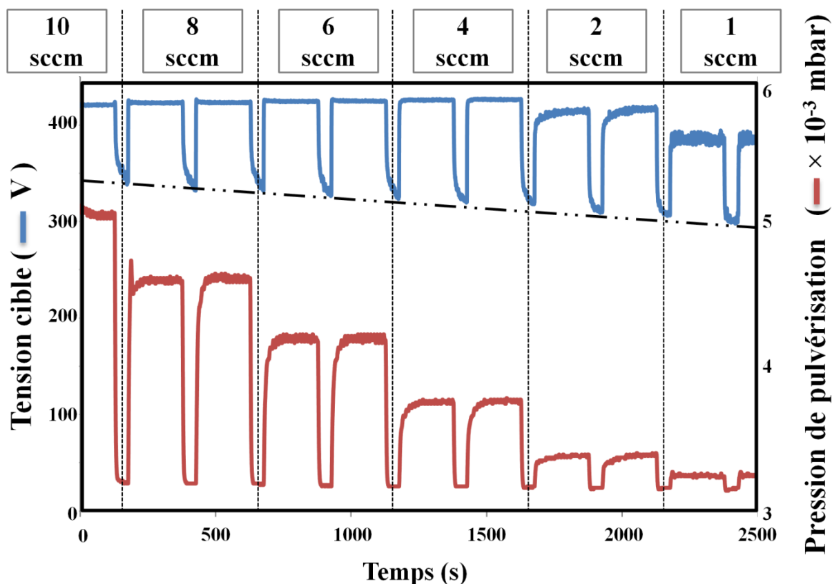
Figure VI.2. Relevés de tension et de pression en fonction du temps et du débit d'oxygène.
