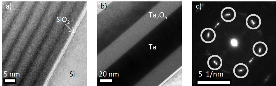
Figure IV.10. Images MET en section transverse du système TaO_x/Ta réalisées pour a) \Lambda = 5,4 \text{ nm} b) \Lambda = 78,6 \text{ nm} et c) cliché SAED des couches Ta_2O_5/Ta (les tâches correspondant à d_{100} de \alpha -Ta sont entourées).
