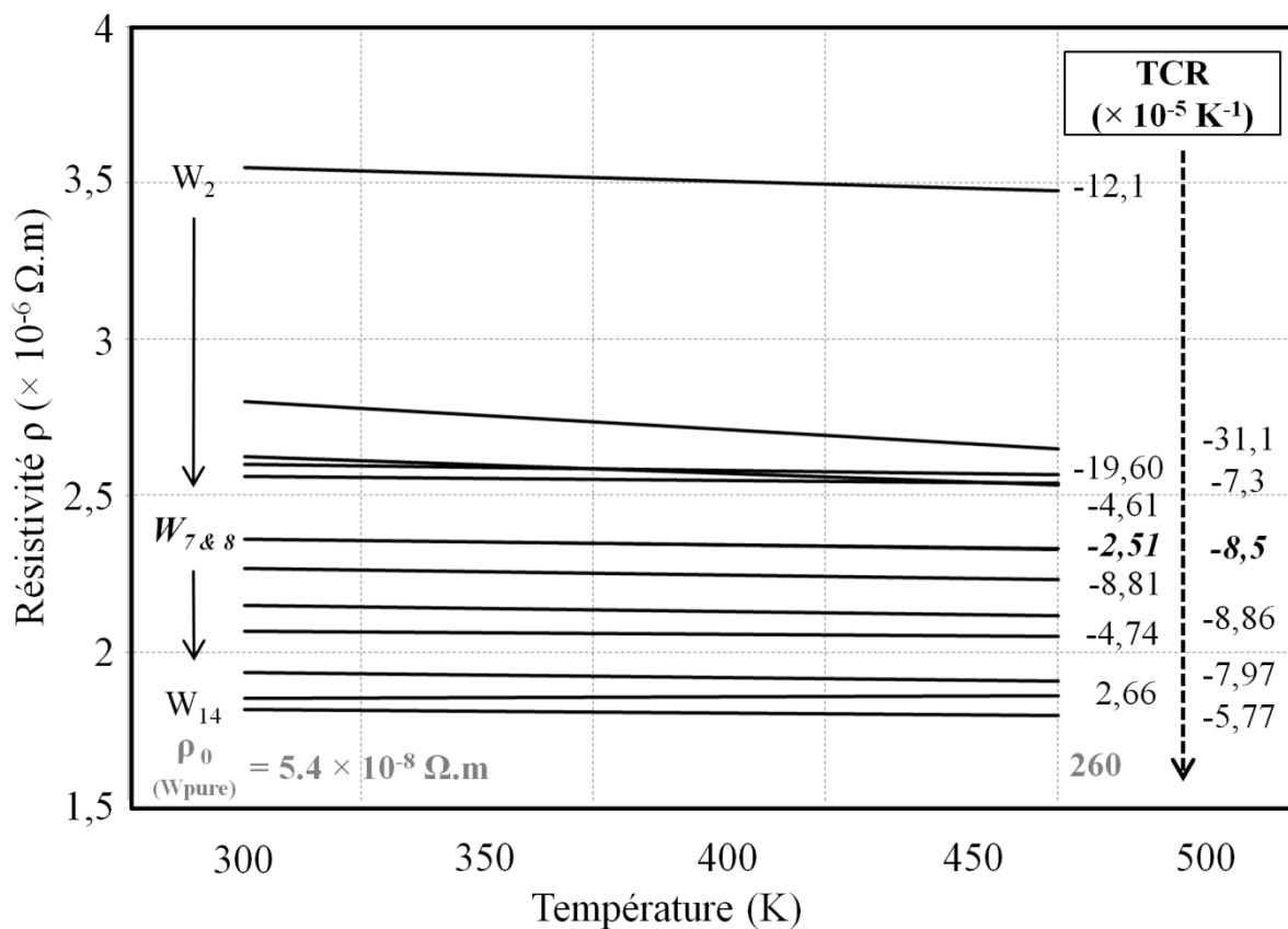
Figure V.3. Evolution de la résistivité en fonction de la température des multicouches périodiques WO/W/WO/WO_3 et leurs valeurs de TCR établie pour \rho_0 à 298 K.
