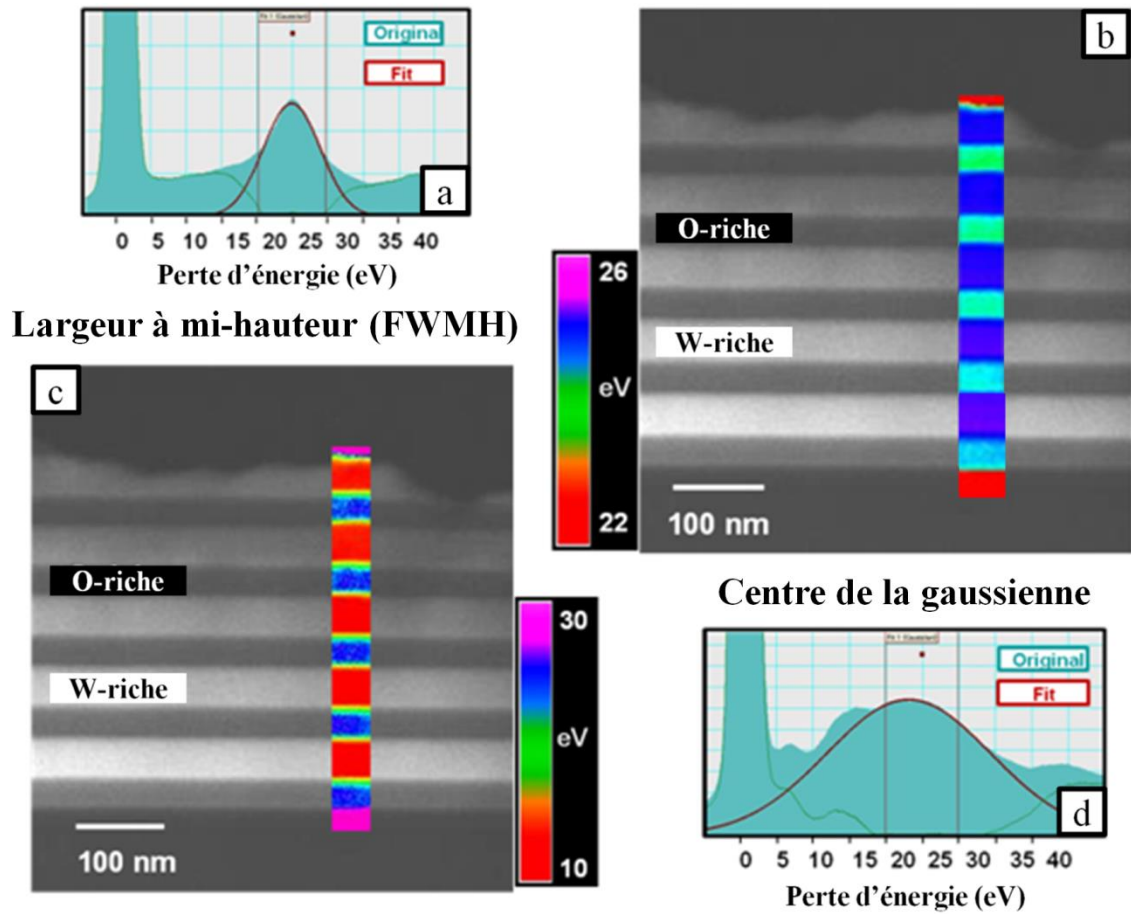
Figure IV.24. Cartographies du centre de la gaussienne (b) et de sa largeur à mi-hauteur (c) superposées à l'image STEM en champ sombre pour un échantillon à base de tungstène ( \lambda = 71,5 \text{ nm} ), spectres EELS extraits de l'image-spectre pour a) la couche W et d) la couche \text{WO}_3 .
