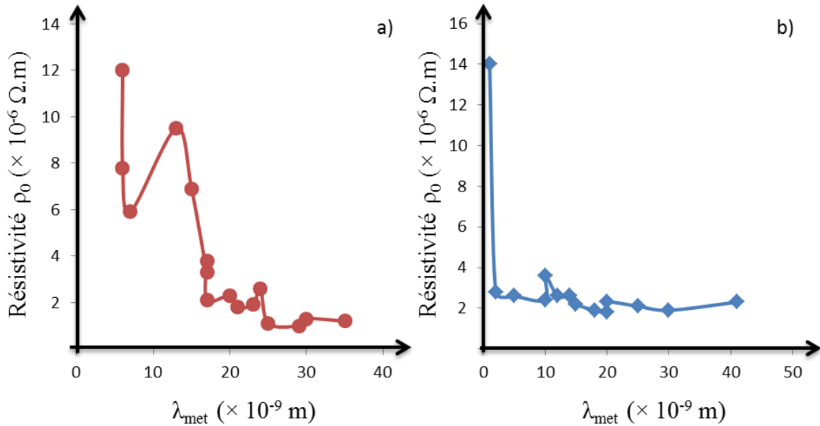
Figure V.4. Résistivité à température ambiante ( \rho_0 ) des systèmes a) TiO/Ti/TiO/TiO 2 et b) WO/W/WO/WO 3 , pour une variation croissante de l'épaisseur de couches \lambda_{\text{met}} .
