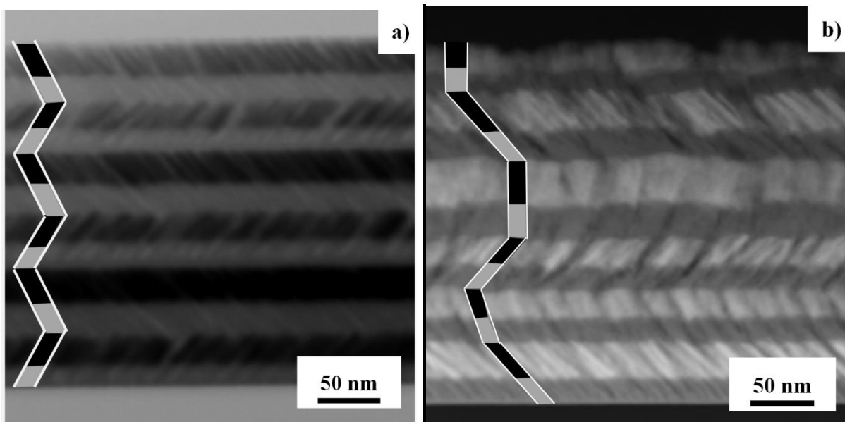
Figure VI.6. Cliché STEM a) en champ clair et b) en champ sombre des structures périodiques métal/oxyde (Ta/Ta 2 O 5 ) colonnaires avec leurs représentations graphiques a) en 2D zigzag sur une période \Lambda = 52 nm et b) en 3D pour une spire carrée sur une période \Lambda = 50 nm.
