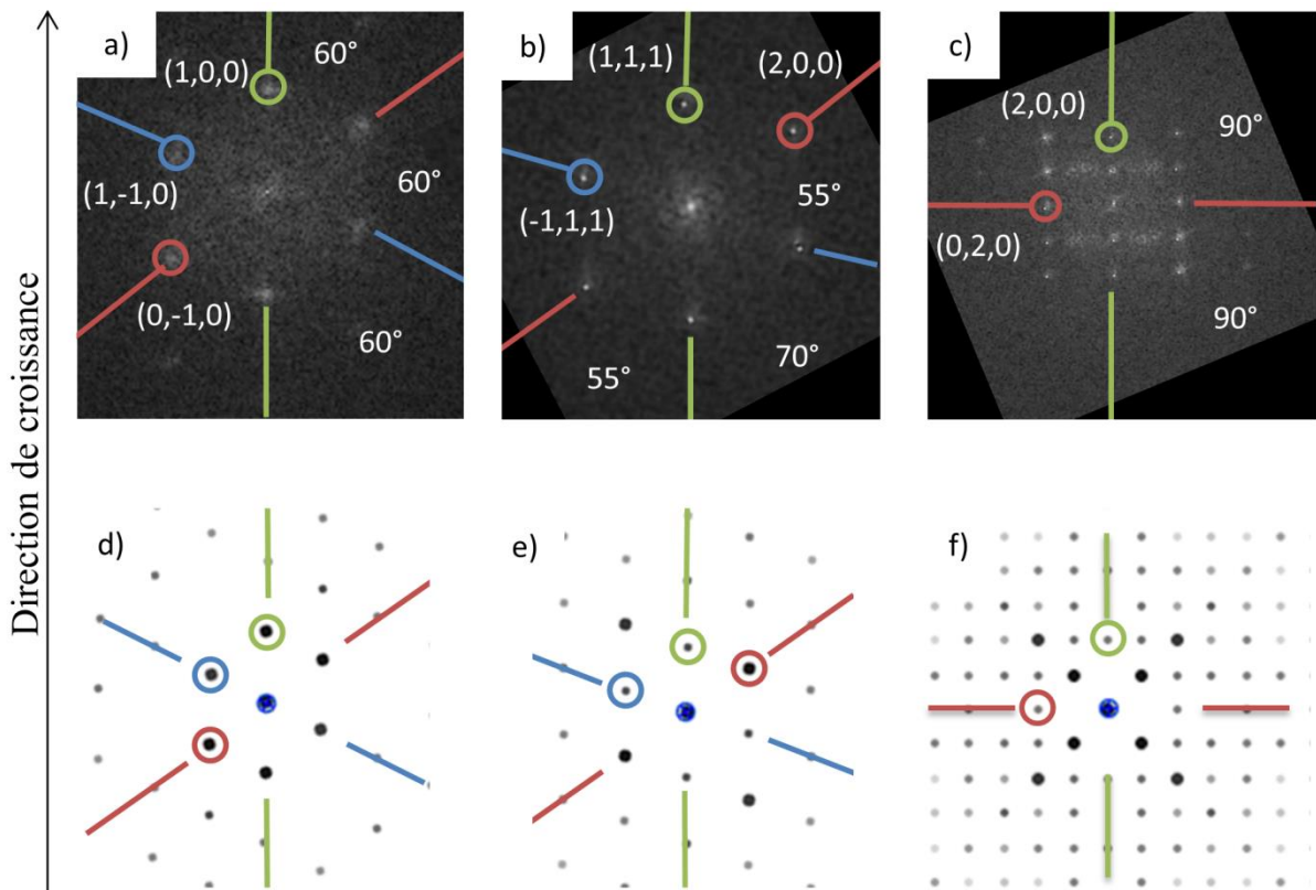
Figure IV.16. Transformées de Fourier obtenues d'un cliché METHR sur une cristallite de la phase a) hexagonale de titane, b) cubique face centré de monoxyde de titane et c) rutile de dioxyde de titane ; ainsi que leurs simulations respectives d), e) et f).
