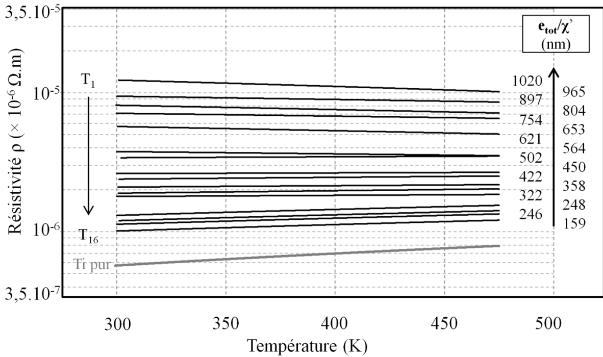
Figure V.8. Résistivité électrique DC \rho en fonction de la température mesurée sur les multicouches TiO/Ti/TiO/TiO 2 . La valeur du rapport e_{tot}/\chi' est systématiquement annoté.
