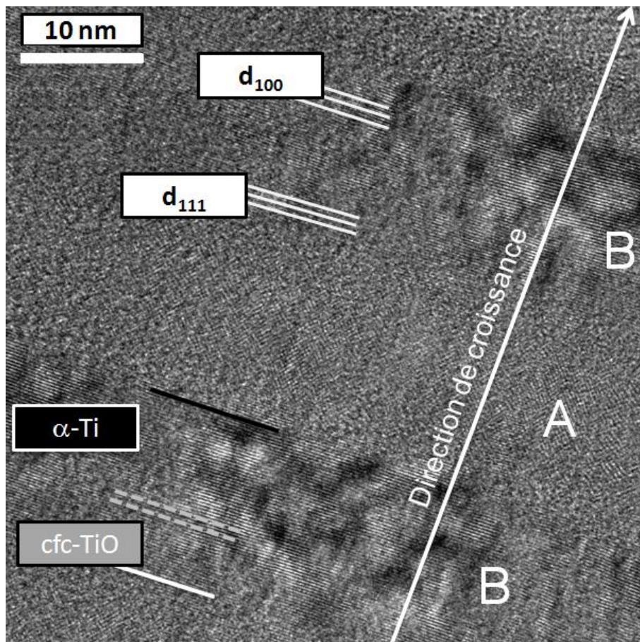
Figure IV.13. Cliché METHR des domaines faiblement cristallisés (A et B) avec l'indexation dans la direction de croissance des distances interréticulaires d_{111} = 0,241 \text{ nm} du cfc-TiO puis d_{100} = 0,255 \text{ nm} de la phase \alpha -Ti.
