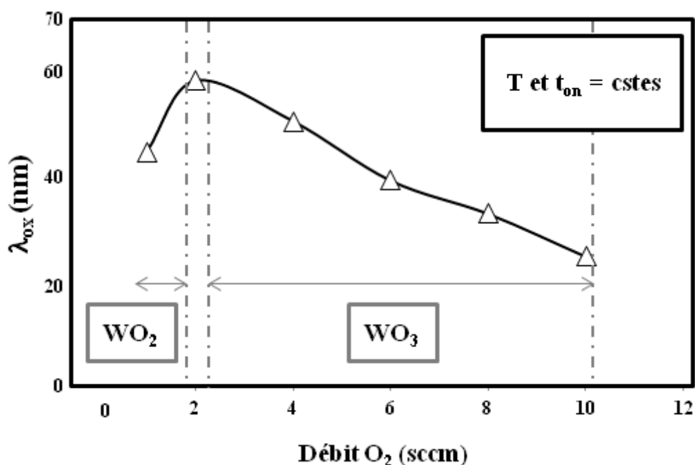
Figure VI.1. Variation de l'épaisseur d'oxyde déposée en fonction du débit d'oxygène injecté avec annotation des stœchiométries relevées par EDX.
