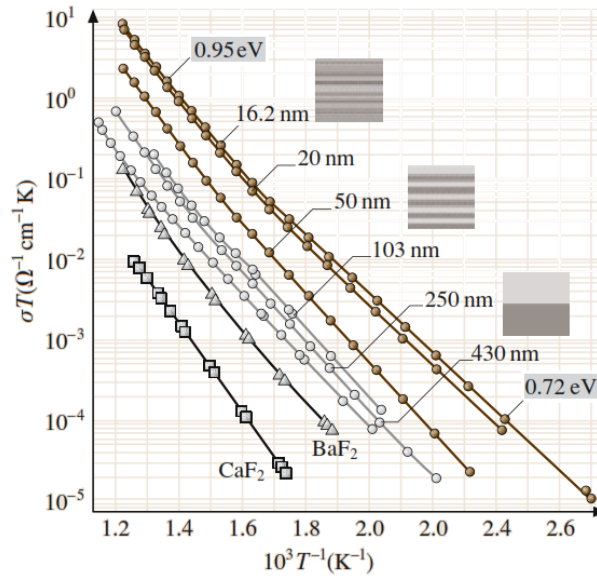
Figure II.2. Conductivité en température des multicouches périodiques \text{CaF}_2/\text{BaF}_2 en fonction de l'épaisseur de leurs sous-périodes [28].
