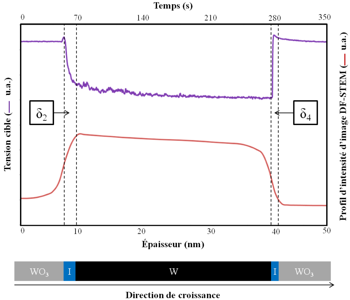
Figure IV.23. Tension de la cible en fonction du temps mise en relation avec le profil d'intensité d'une image DF-STEM mesuré sur une période métallique (avec I représentant les sous-couches interstitielles).
