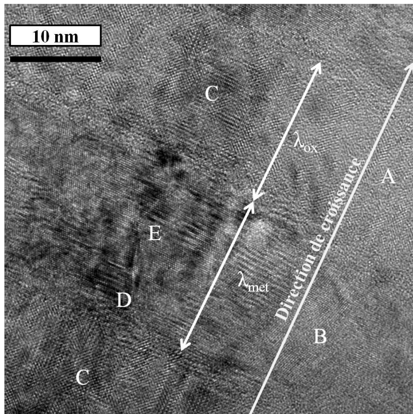
Figure IV.14. Cliché METHR de l'interface des domaines faiblement cristallisés (A et B) et totalement cristallins (C, D et E) d'un échantillon de période \Lambda = 30 nm.
