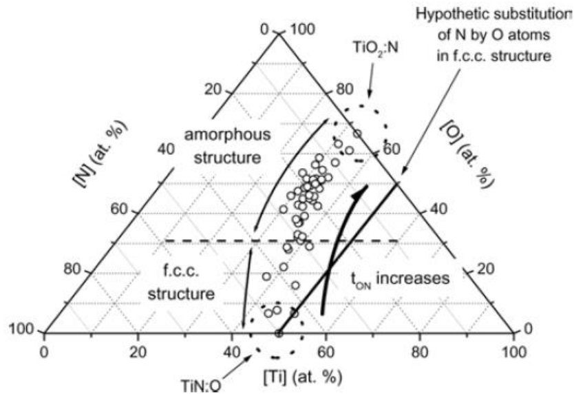
Figure I.3. Exemple de variation de composition chimique de films d'oxynitrides de titane élaborés par pulvérisation cathodique réactive [18].
