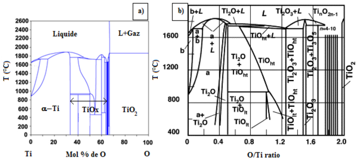
Figure IV.19. Diagrammes de phases Ti-O a) calculé par Cancarevic et al. [11] et b) établi par Diebold [10].
