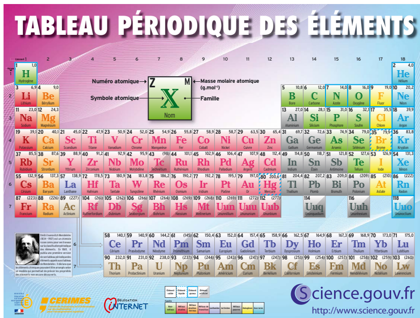
FIGURE 1.1 – Tableau périodique de Mendeleïev
