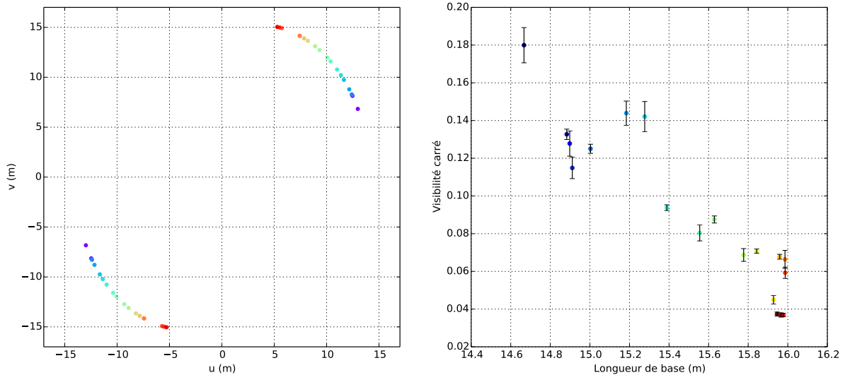
FIGURE 5.7 – Gauche : Plan (u,v) des données VINCI, l'échelle de couleur correspond à l'angle projeté de la base sur le ciel. Droite : Visibilitées mesurées par VINCI sur L 2 Pup, l'échelle de couleur correspond à l'angle projeté de la base sur le ciel.
