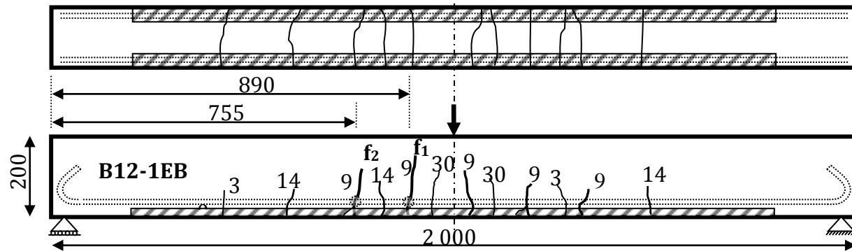
Figure III-27 : Cartes des fissurations de la poutre B12-1EB au niveau de pré-chargement de 13.5 kN.m.
