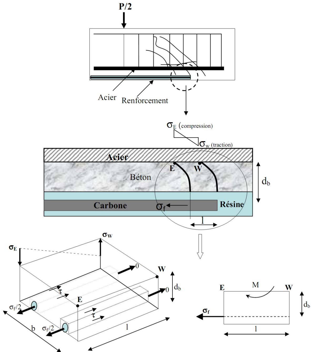
Figure I-21 : Répartition des contraintes dans le béton et les joncs de carbone entre les deux dernières fissures à l'extrémité des joncs de carbone.
