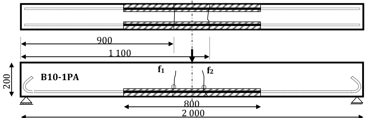
Figure III-28 : Cartes des fissurations de la poutre B10-1PA au niveau de pré-chargement de 13.5 kN.m.
