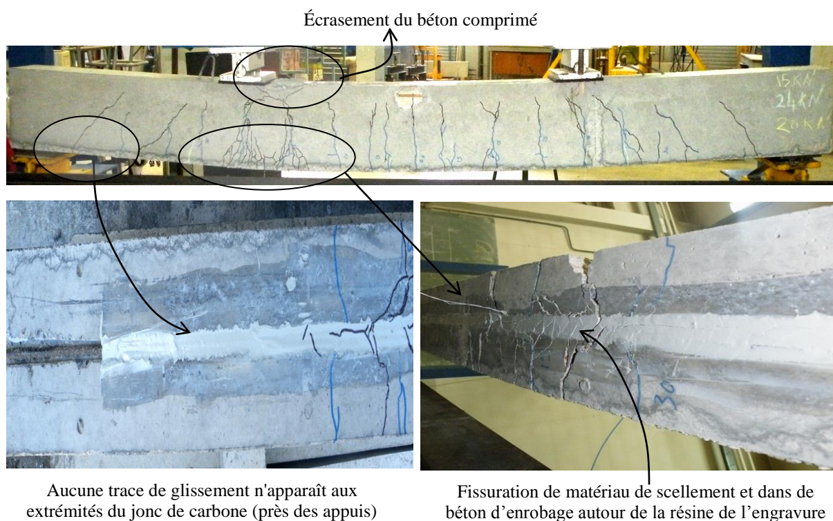
Figure IV-40 : Mode de ruine de la poutre réparée P72-72.
