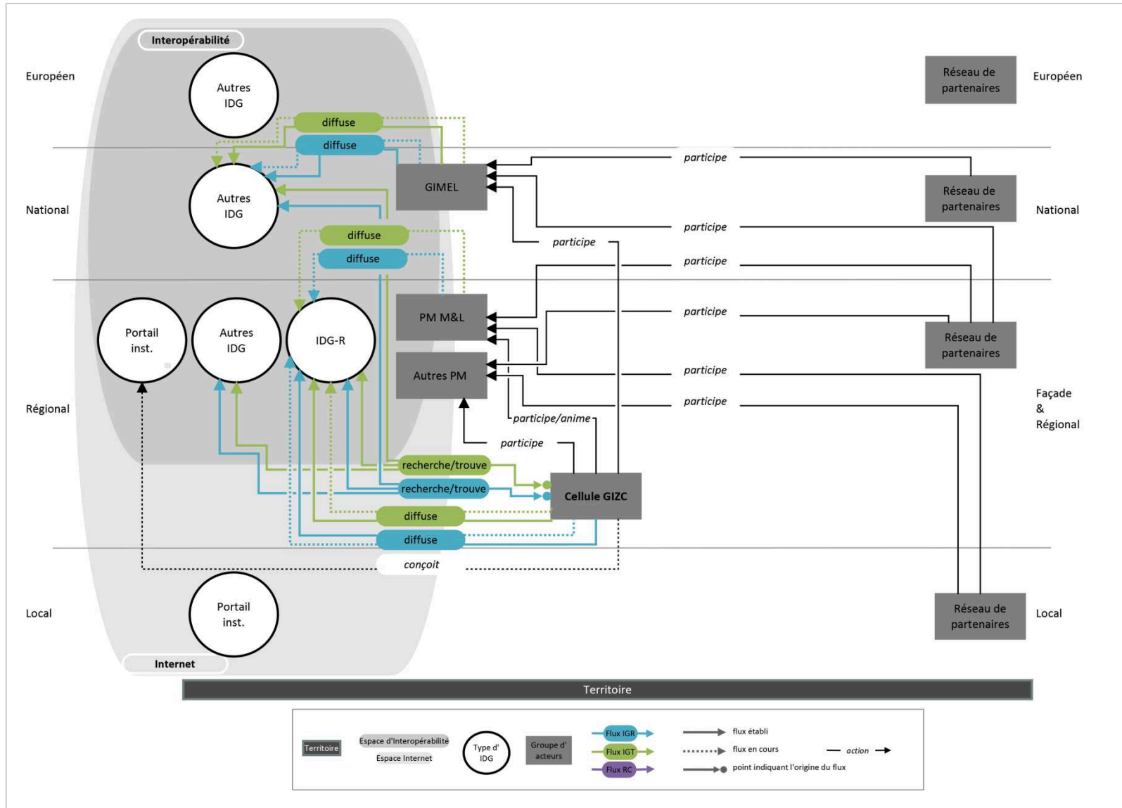
Figure 52. Diagramme DFD de contexte du cas Bretagne- cellule GIZC régionale/de façade
