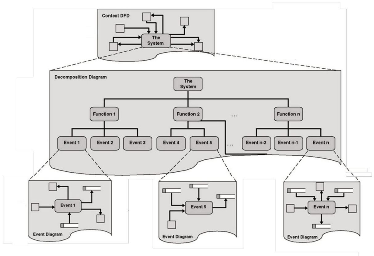
Figure 45. Emboîtement des diagrammes (Whitten et Bentley, 2005)
