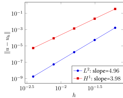
3.1.4. P4 mortar FEM
