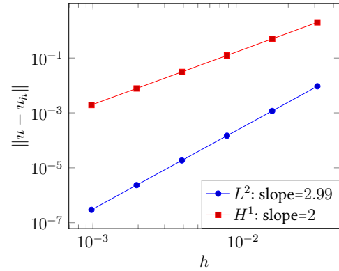
3.1.2. P2 mortar FEM
