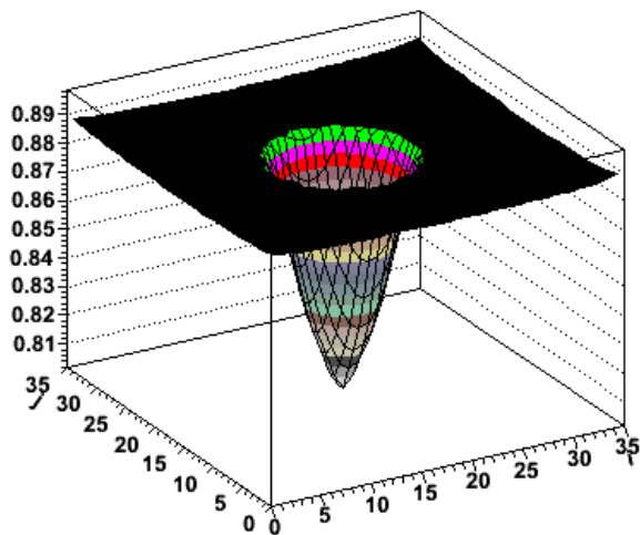
FIGURE 6.16 – Mesures versus modélisation de la transmission du filtre g_M éclairé par les LEDs 400 et GD2. Le modèle décrit la variation radiale de la transmission des filtres, mais il ne tient pas compte des reflets (comme celui de la lentille L3), visible au centre du graphique représentant l'image de la LED 400 (en haut, à gauche). Le modèle ne reproduit pas non plus l'amplitude moyenne : l'image réelle et la simulation de la transmission du filtre éclairé par la LED GD2 sont en désaccord de 3%.
