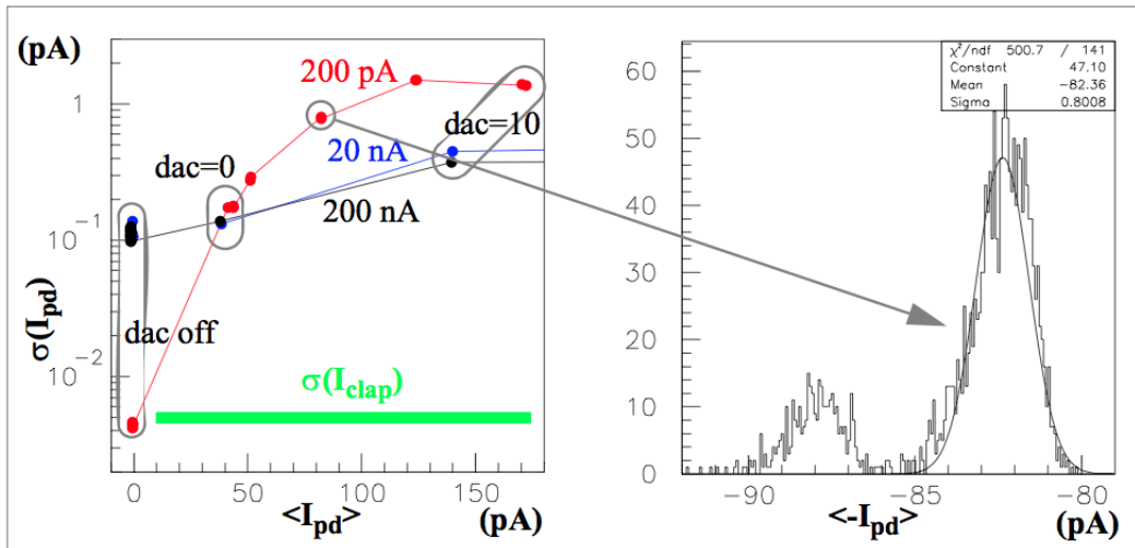
FIGURE 2.19 – A gauche : comparaison de la lecture du photocourant et du bruit par trois différents calibres du pico-ampèremètre : rouge, bleu et noir pour le 200 pA, 20 nA and 200 nA. Les points ayant le même niveau DAC sont entourés en gris (off, 0, 10). A droite : l’histogramme montre la distribution bimodale du bruit mesuré par le calibre 200pA.
