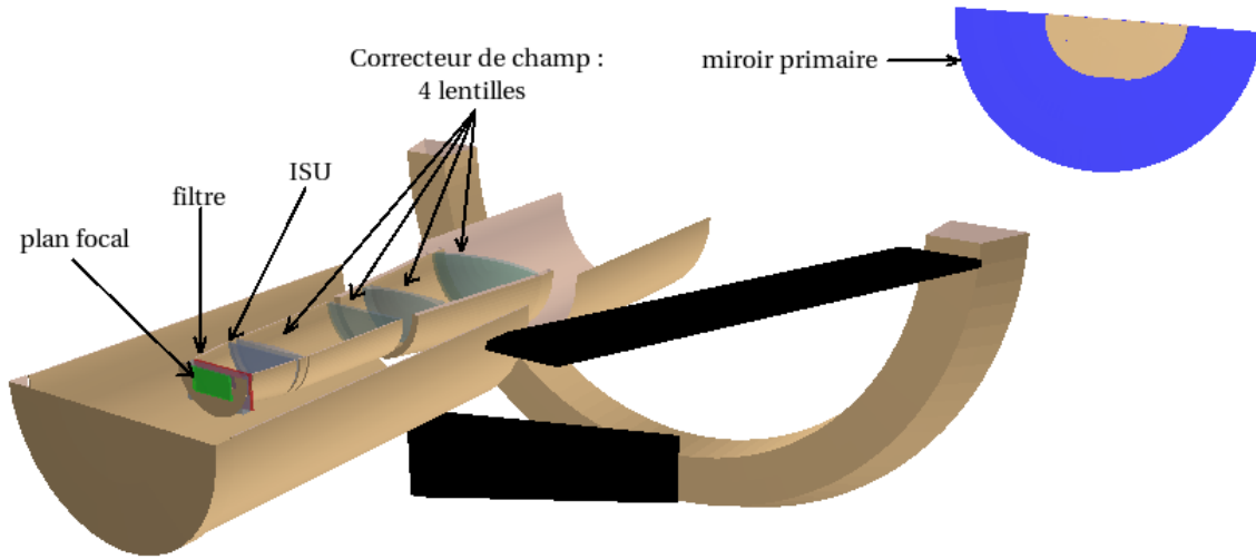
FIGURE 1.3 – Modélisation 3-D en coupe de MegaPrime au CFHT. Le miroir primaire est représenté, à droite, en bleu, ainsi que l’occultation centrale (en beige). A gauche, MegaPrime est constitué d’une armature rigide supportant la caméra MegaCam (rectangle vert), installée au plan focal, devant un jeu de filtres interchangeable (en rouge). L’ISU ( Image Stabilizing Unit ), une plaque épaisse en verre qui permet de stabiliser l’image ( http://www.lesia.obspm.fr/Stabilisateur-d-image-pour-le.html ), et les lentilles apparaissent en bleu-gris sur le chemin optique.
