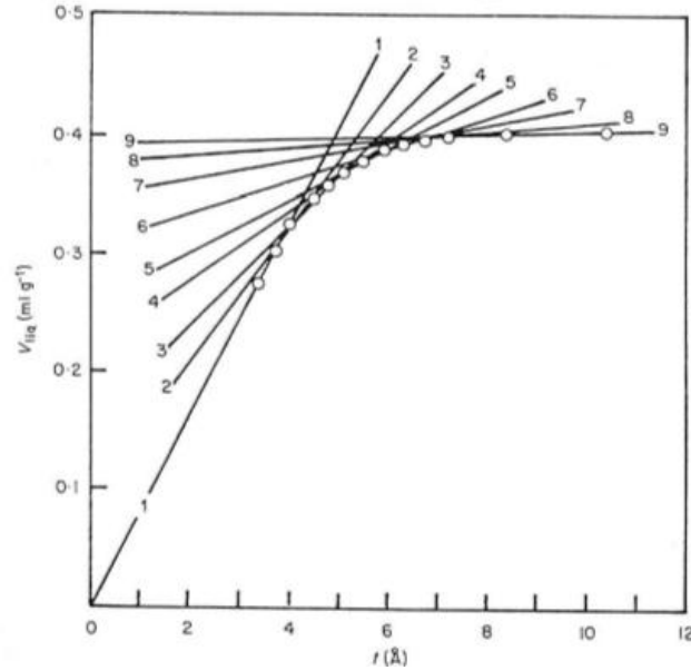
Figure II.1.4. Exemple de courbe du volume condensé, V_c , en fonction de t et de son traitement par la méthode MP [88].
