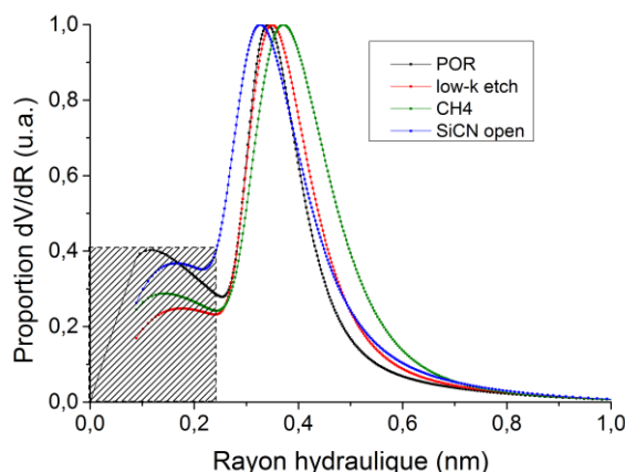
Figure VII.2.17. Distributions en taille de pores pour le LDR3 bulk gravé par les différents plasmas, selon la méthode MP. La zone grisée correspond à un artefact de la méthode.
