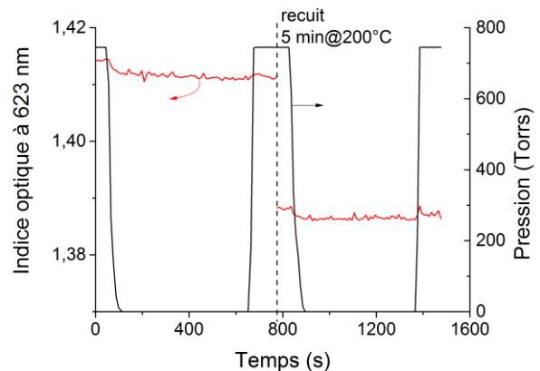
Figure VII.2.11. Effet de la mise sous vide sur l'indice optique d'un échantillon stack gravé par plasma.
