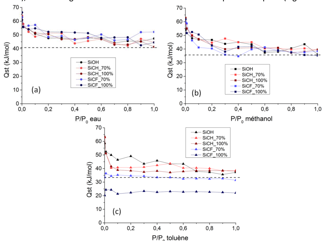
Figure VII.1.11. Chaleurs isostériques extraites des modélisations d'adsorption (a) de l'eau, (b) du méthanol, et (c) du toluène sur les cinq surfaces (noir : SiOH, rouge : SiCH 3 ( \eta = 70\% ), marron : SiCH 3 ( \eta = 100\% ), bleu clair : SiCF 3 ( \eta = 70\% ), bleu foncé : SiCF 3 ( \eta = 100\% ). Les lignes pointillées représentent l'enthalpie de vaporisation.
