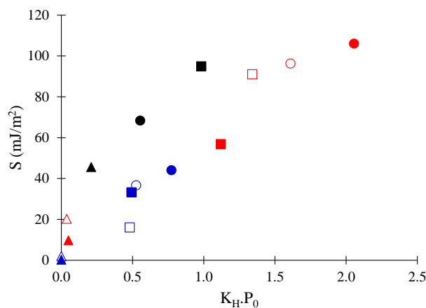
Figure VII.1.14. Coefficient d'étalement S en fonction de la constante de Henry corrigée par la pression de vapeur saturante K_H' = K_H P_0 pour l'eau (cercles), le méthanol (carrés) et le toluène (triangles) adsorbés sur les surfaces de silice hydroxylée (noir), méthylée (rouge) et trifluorométhylées (bleu). Les symboles vides sont pour \eta = 70\% , et les pleins pour \eta = 100\% .
