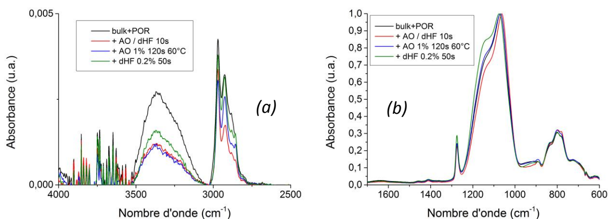
Figure VI.2.10. Spectres FTIR-ATR du low- k LDR3 bulk gravé par le POR (noir) et LDR3 modifié par les traitements de nettoyage (a) de 4000 à 2500 \text{cm}^{-1} , et (b) de 1700 à 600 \text{cm}^{-1} .
