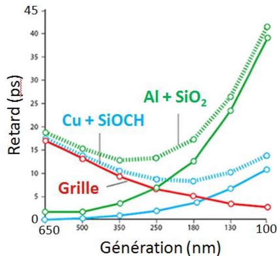
Figure I.1.3. Retard du signal dû à la grille et aux interconnexions, d'après l'ITRS [8].
