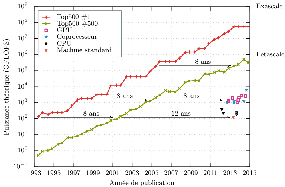
Figure 1.3. – Évolution du classement du TOP500
