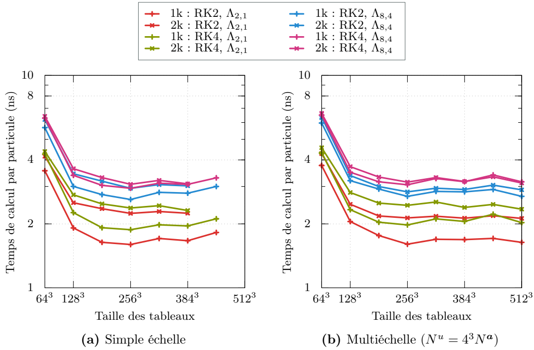
Figure 5.24. – Performances globales de la méthode pour un transport de scalaire 3D
