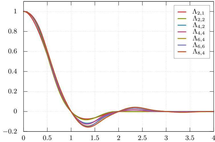
Figure 2.10. – Noyaux de remappage de type \Lambda_{p,r}
