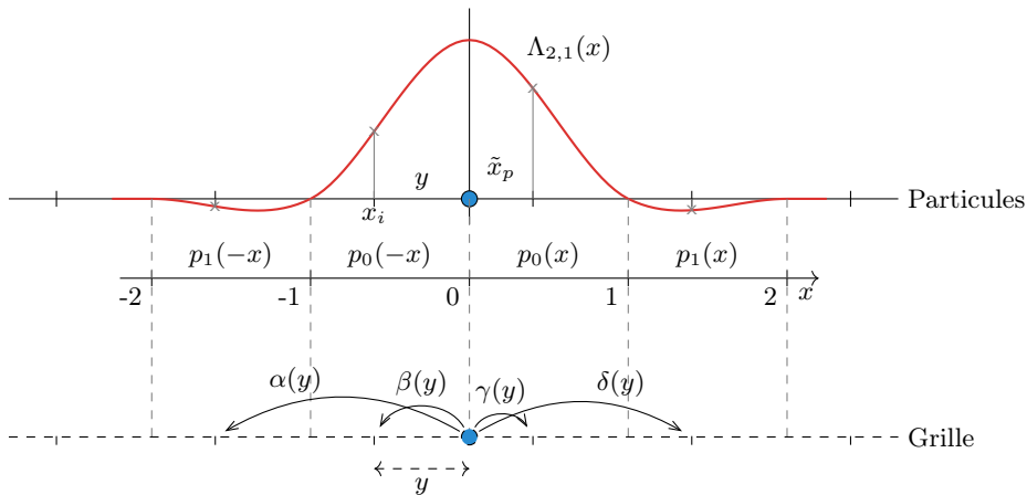
Figure 2.11. – Obtention des poids de remappage pour une formule de support [-2; 2]
