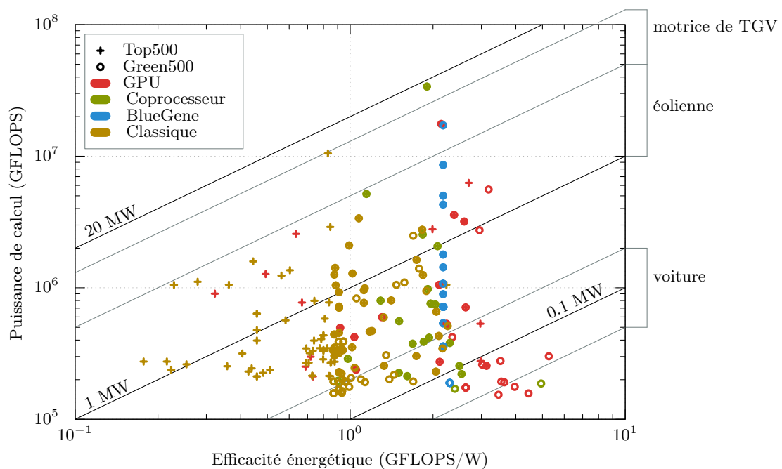
Figure 1.6. – Comparaison des performances énergétiques des 150 premières machines du Top500 et Green500 selon le matériel (classements de novembre 2014).
