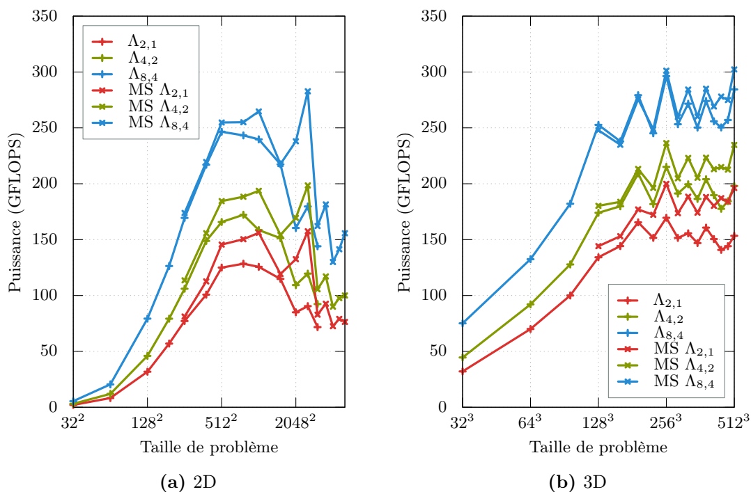
Figure 5.17. – Performances des noyaux d'advection et remaillage pour un schéma RK2
