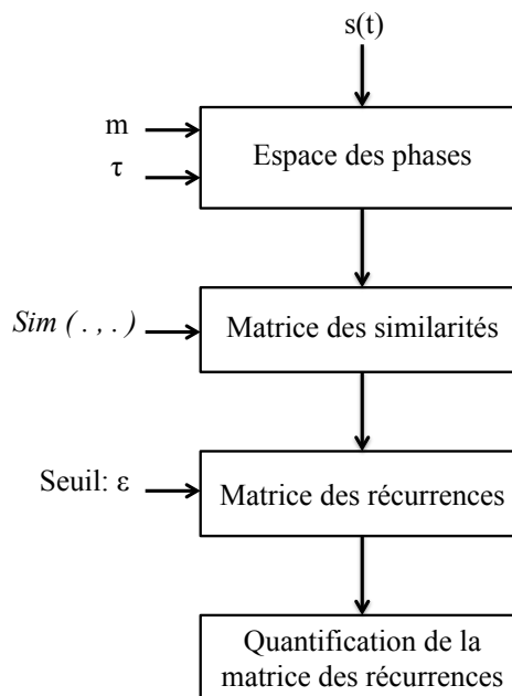
FIGURE 3.1 – Schéma bloc des étapes de construction menant à la détection des récurrences de phase d'un signal. Quatre degrés de liberté sont nécessaires : \tau le délai et m la dimension permettent de reconstruire l'espace des phases, Sim(. , .) la fonction utilisée pour calculer la matrice des similarités, \varepsilon le seuil de détection pour calculer la matrice des récurrences .
