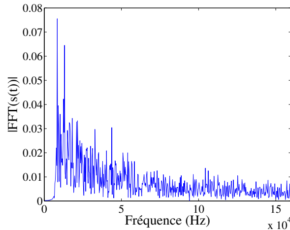
FIGURE 4.15 – Spectre de 7000 échantillons du bruit, tirés de la base de données. Le spectre est décroissant à mesure que la fréquence augmente, ce qui montre sa non-blancher.
