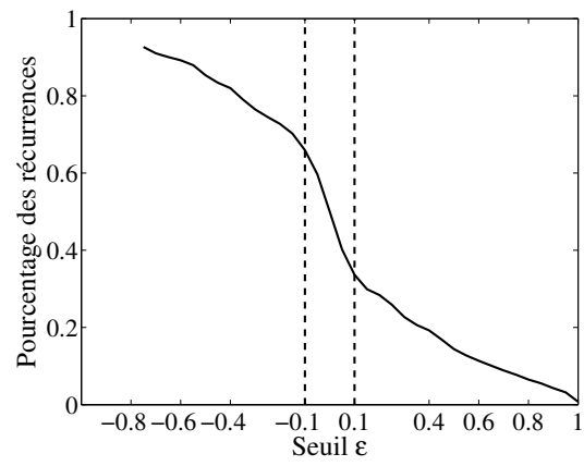
FIGURE 3.10 – Évolution du pourcentage de récurrences dans les images de la figure 3.9 en fonction du seuil \epsilon .
