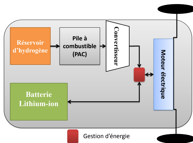
Figure I.18 – Structure de la chaîne énergétique : PAC, batterie
