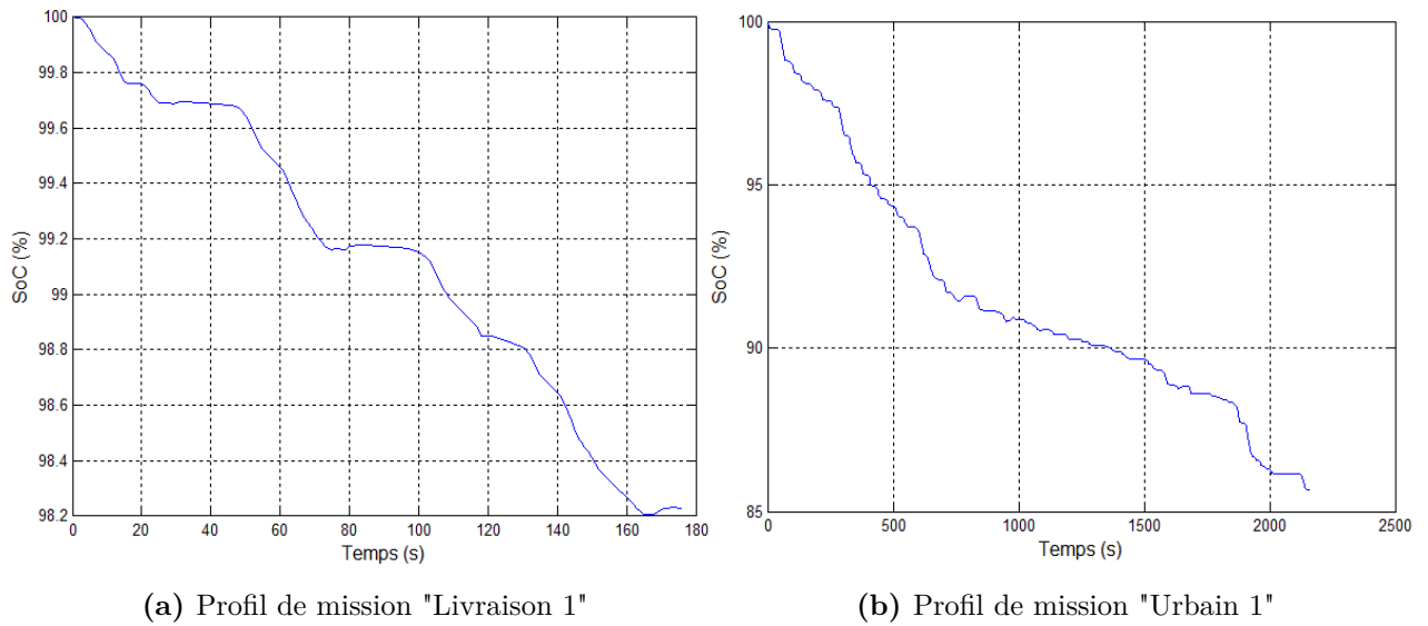
Figure IV.17 – Décharge de la batterie
