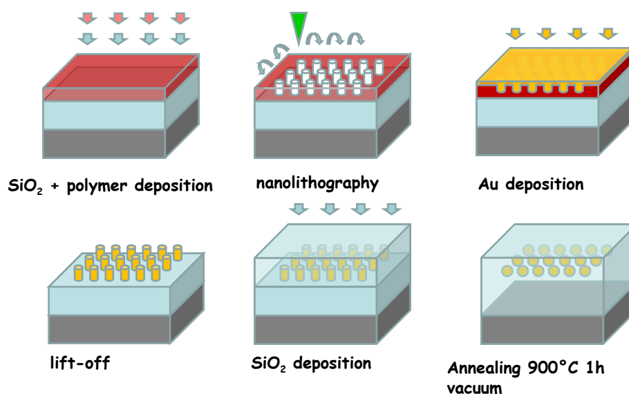
FIGURE 4.1 – Les différentes étapes de la nanolithographie. Figure extraite du travail de l'équipe de G. Rizza.
