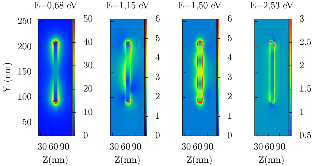
FIGURE 4.12 – Carte 2D du rapport E/E_0 d'un nanofil d'or de rapport d'aspect R = 12 obtenue par ADE-FDTD.
