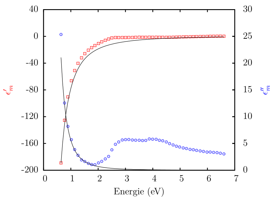
FIGURE 2.15 – Comparaison de la permittivité relative (partie réelle et imaginaire) pour l'or entre les données expérimentales de Johnson-Christy (symboles) et le modèle de Drude (lignes) ( \omega_p = 1,35 \cdot 10^{16} \text{ rad.s}^{-1} , \gamma = 1,08 \cdot 10^{14} \text{ rad.s}^{-1} )
