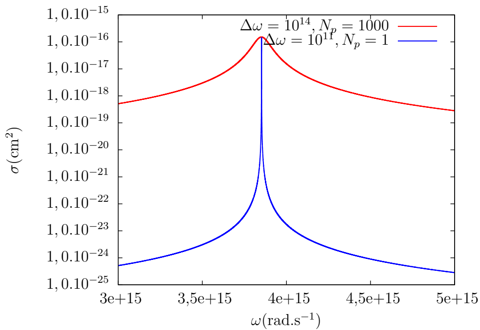
FIGURE 3.7 – Section efficace en fonction de la pulsation \omega pour une transition avec \omega_{ij} = 3,8 \cdot 10^{15} \text{ rad.s}^{-1} pour deux couples de paramètres (largeur de raie \Delta\omega , nombre de polarisations N_p ) conduisant à la même section efficace lorsque \omega = \omega_{ij}
