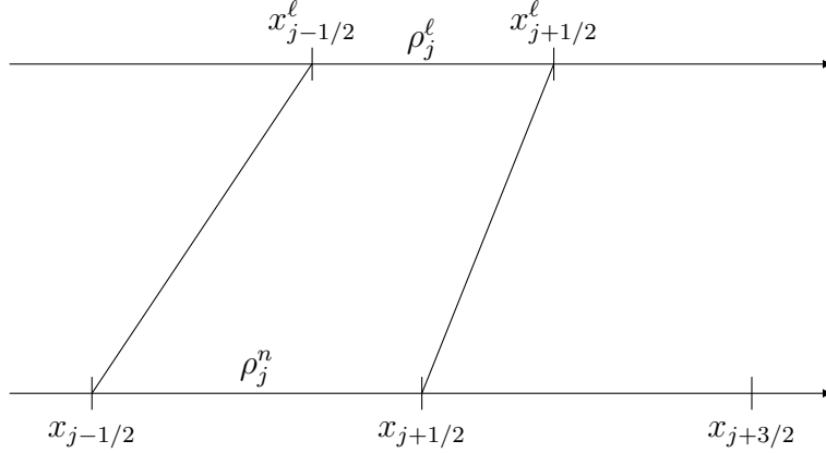
FIGURE 2.12 – Etape Lagrangienne.
