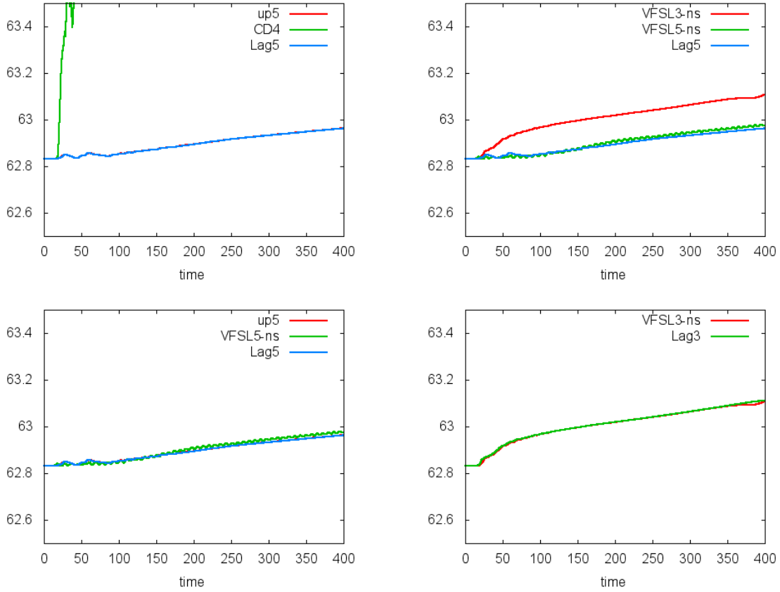
FIGURE 4.7 – Cas test Bump On Tail : évolution en temps de la norme L^1 pour la méthode de "Banks" (CD4 et up5), pour la méthode Vfls sans splitting (Vfsl3-ns et Vfsl5-ns) et pour la méthode semi-Lagrangienne (Lag3 et Lag5). N_x = N_v = 128 , \Delta t = 0.01 .
