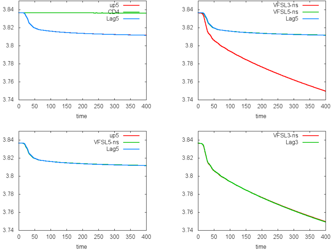
FIGURE 4.6 – Cas test Bump On Tail : évolution en temps de la norme L^2 pour la méthode de "Banks" (CD4 et up5), pour la méthode Vfsl sans splitting (Vfsl3-ns et Vfsl5-ns) et pour la méthode semi-Lagrangienne (Lag3 et Lag5). N_x = N_v = 128 , \Delta t = 0.01 .
