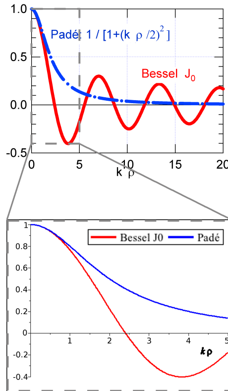
FIGURE 8.1 – La fonction de Bessel J_0(k\rho) comparée à son approximation de Padé 1/[1 + (k\rho)^2/4] .
