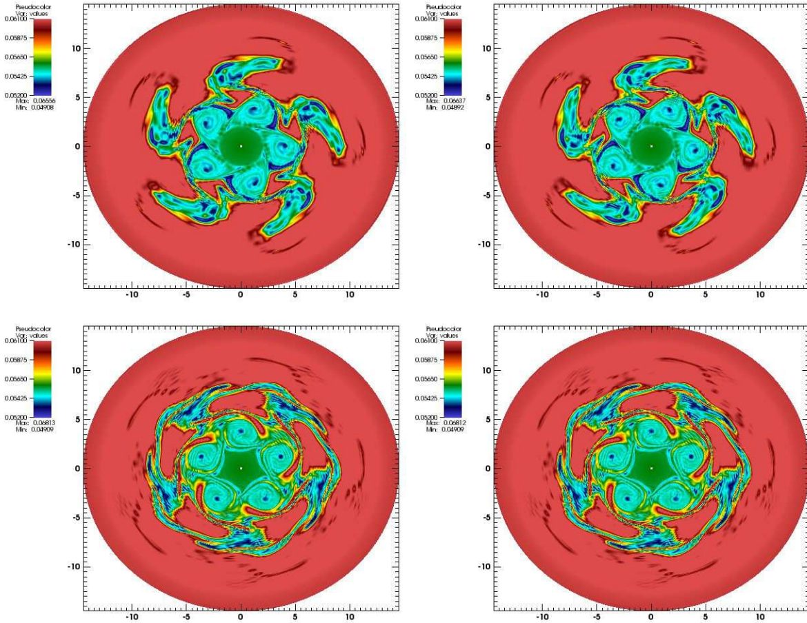
FIGURE 8.7 – Coupe polôïdale f(r, \theta, z = 0, v_{\parallel} = 0) au temps T = 5000 pour 128 \times 128 \times 128 \times 128, \Delta t = 1 . En haut (de gauche à droite) : \mu = 0.1 avec Hermite et puis Padé ; en bas (de gauche à droite) : \mu = 0 , avec Hermite et puis Padé.
