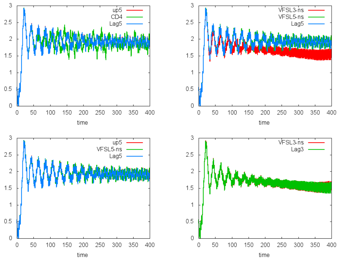
FIGURE 4.3 – Cas test Bump On Tail : évolution en temps de l'énergie électrique pour les méthodes de "Banks" (CD4 et up5), pour les méthodes Vfl non splittées (Vfl3-ns et Vfl5-ns) et pour la méthode demi-Lagrangienne (Lag5). N_x = N_v = 128 , \Delta t = 0.01 .
