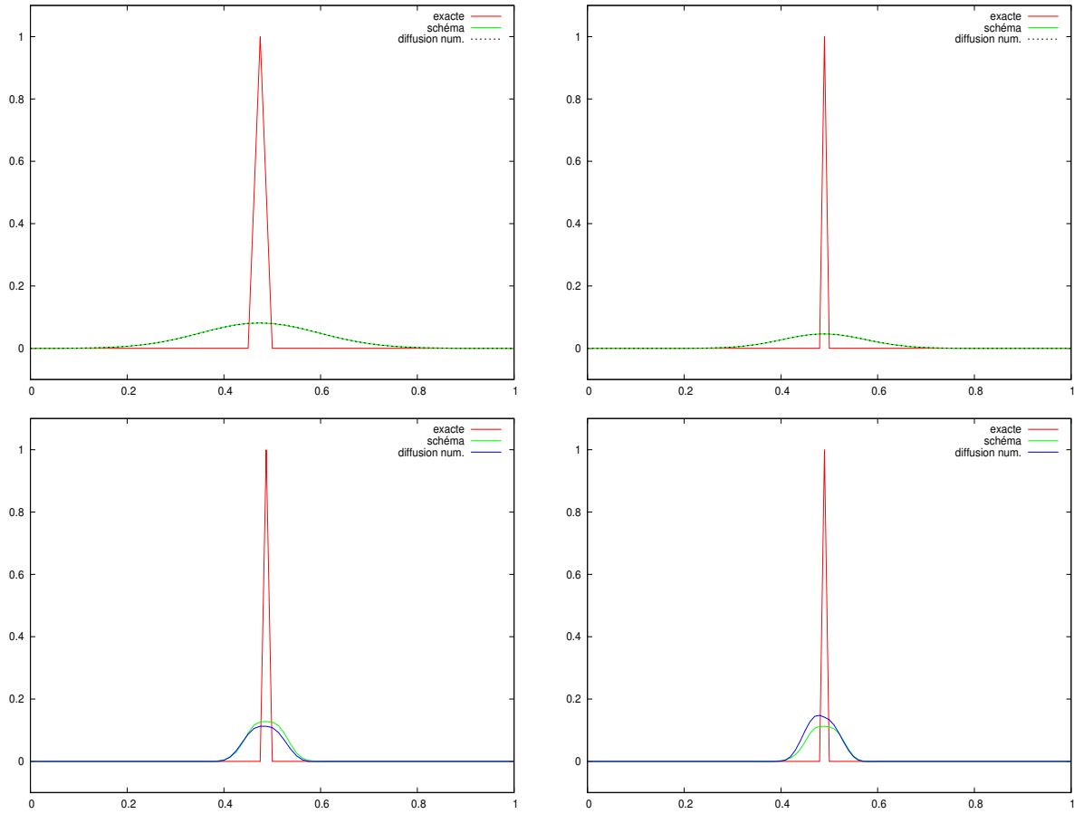
FIGURE 2.14 – Dirac discret, sans limiteur de pente, \Delta x = 1/40 , \Delta t = 0.01 , \eta = 0.4 (en haut à gauche), \Delta x = 0.01 , \Delta t = 0.0025 , \eta = 0.25 (en haut à droite) ; avec limiteur de pente, \Delta x = 1/80 , \Delta t = 0.005 , \eta = 0.4 (en bas à gauche), \Delta x = 0.01 , \Delta t = 0.0025 , \eta = 0.25 (en bas à droite).
