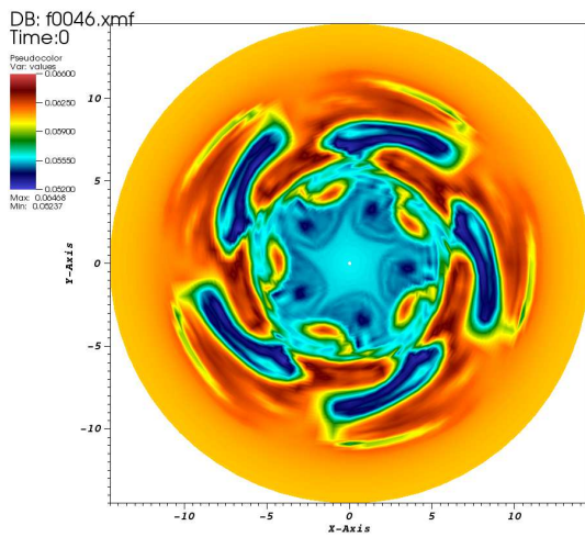
FIGURE 7.1 – Coupe polioïdale f(r, \theta, z = 0, v_{||} = 0) pour 64 \times 64 \times 32 \times 64 , T = 4600 avec \Delta t = 4 (à gauche) et \Delta t = 2 (à droite); LAG3 (en haut), LAGH5 (au milieu) et LAGH9 (en bas).
