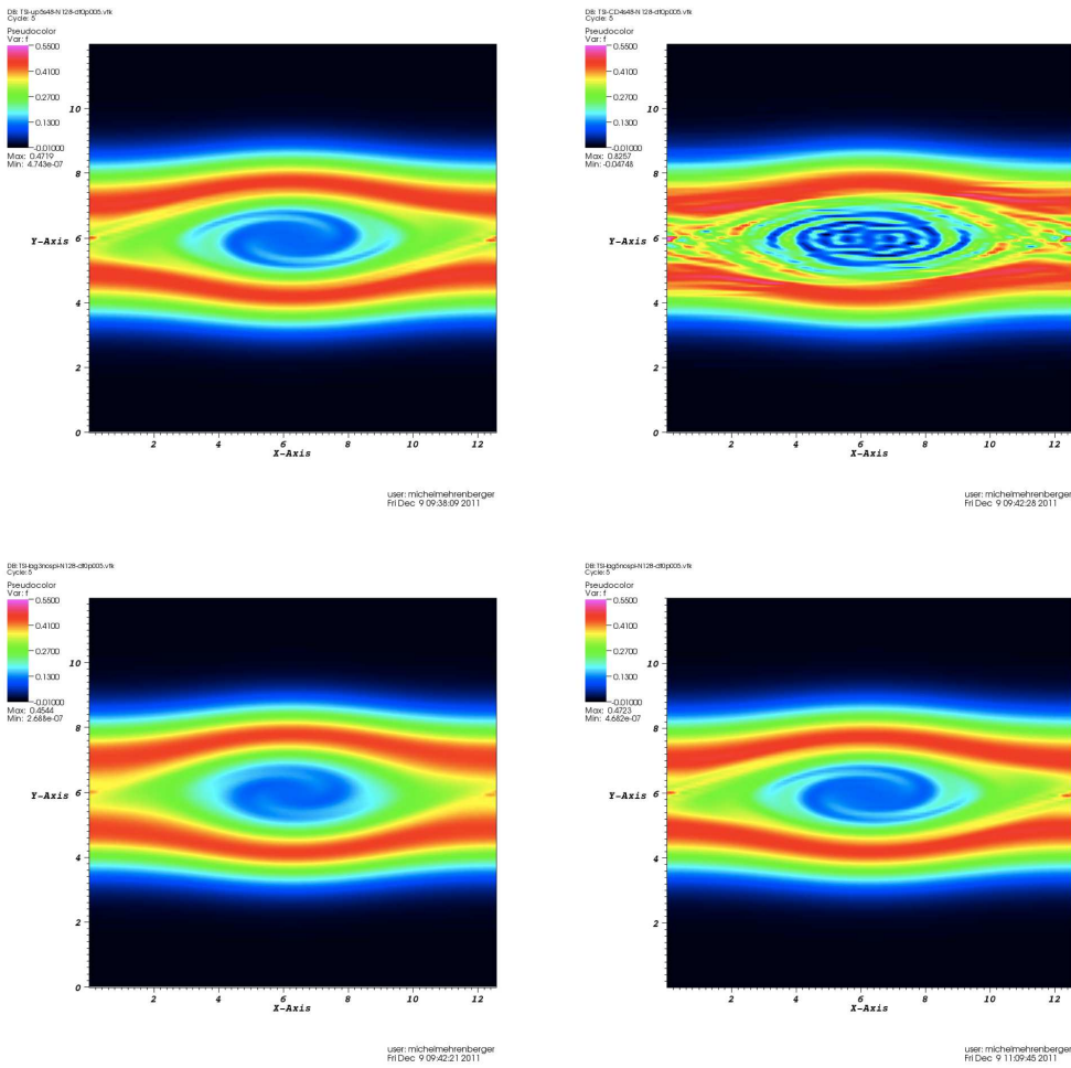
FIGURE 4.8 – Cas test Instabilité double faisceaux : fonction de distribution en fonction de x et v au temps t = 53 pour (du haut vers le bas et de gauche à droite) : up5, CD4, Vfl3-ns, Vfl5-ns. N_x = N_v = 128 , \Delta t = 0.005 .
