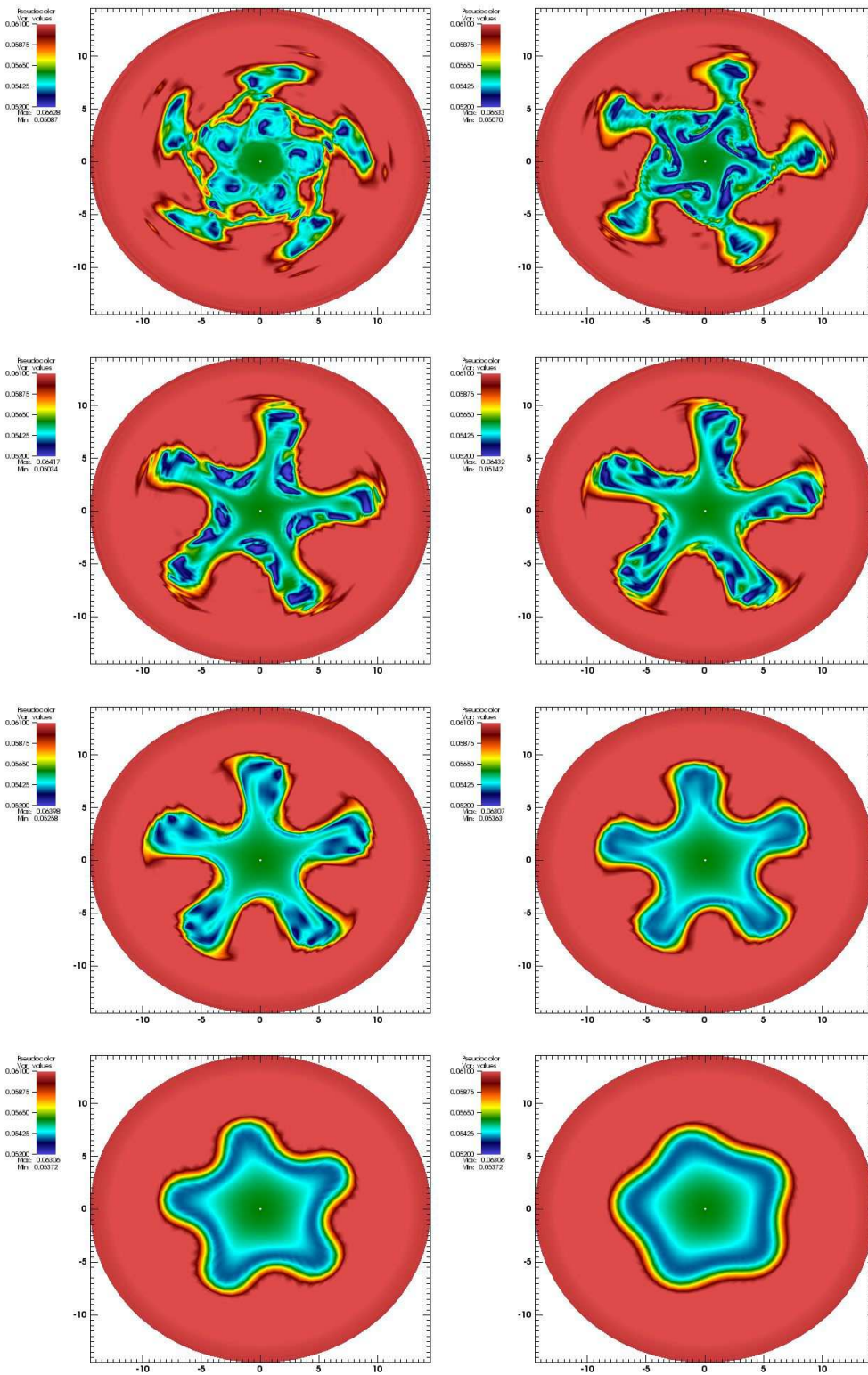
FIGURE 8.8 – coupe polôidale f(r, \theta, 0, 0) au temps T = 5000 avec 64 \times 64 \times 32 \times 64 points et \Delta t = 5 , Hermite avec \mu = 0.1, \dots, 0.8 (de gauche à droite et de haut en bas).
