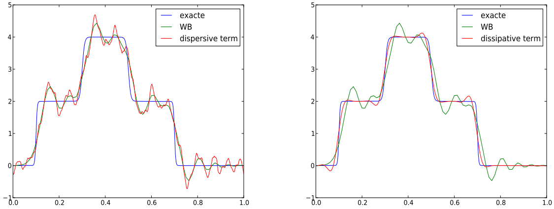
FIGURE 2.3 – Profils de la solution exacte (en bleu), de la solution du schéma de Warming-Beam (en vert) et la solution discrétisée par différences finies de l'équation équivalente (en rouge) en considérant uniquement le terme en \partial_x^3 u (à gauche) et en considérant uniquement le terme en \partial_x^4 u (à droite). \Delta x = 1/80 , \Delta t = 0.01 , a = 1 .
