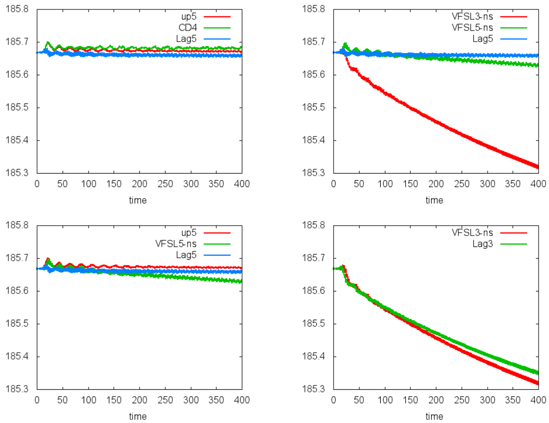
FIGURE 4.5 – Cas test Bump On Tail : évolution en temps de l'énergie totale pour la méthode de "Banks" (CD4 et up5), pour la méthode VfsL sans splitting (Vfsl3-ns et Vfsl5-ns) et pour la méthode semi-Lagrangienne (Lag3 et Lag5). N_x = N_v = 128 , \Delta t = 0.01 .
