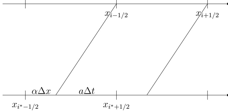
FIGURE 2.4 – Méthode semi-Lagrangienne.
