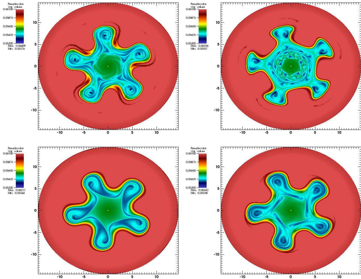
FIGURE 8.6 – Coupe poloidale f(r, \theta, z = 0, v_{\parallel} = 0) au temps T = 7000 pour 128 \times 256 \times 128 \times 128, \Delta t = 2 . En haut (de gauche à droite) : \mu = 0.5 avec Hermite et puis Padé ; en bas (de gauche à droite) : \mu = 1 , avec Hermite et puis Padé.
