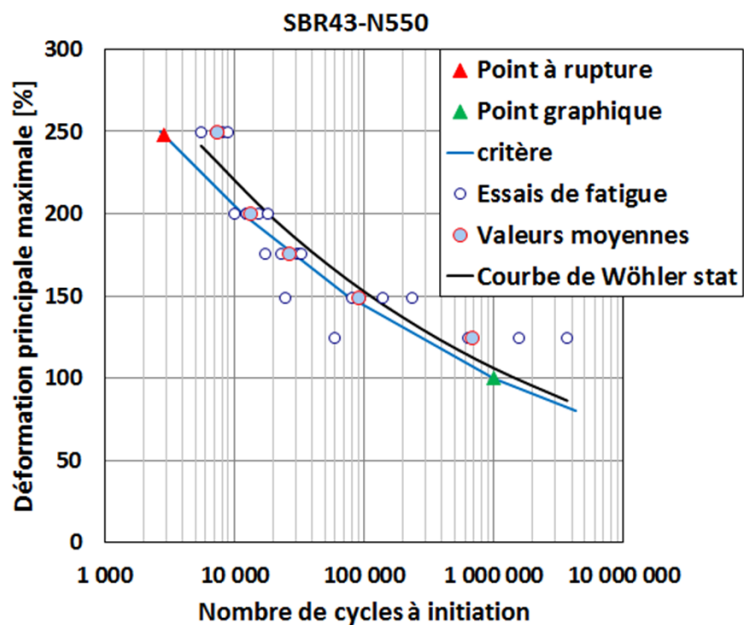
Figure 5.18 – Prédiction du critère énergétique pour le SBR43-N550.
