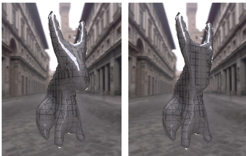
(a) Résolution avec 1445 éléments dont 490 tétraèdres, 217 prismes, 427 pyramides et 311 hexaèdres.
