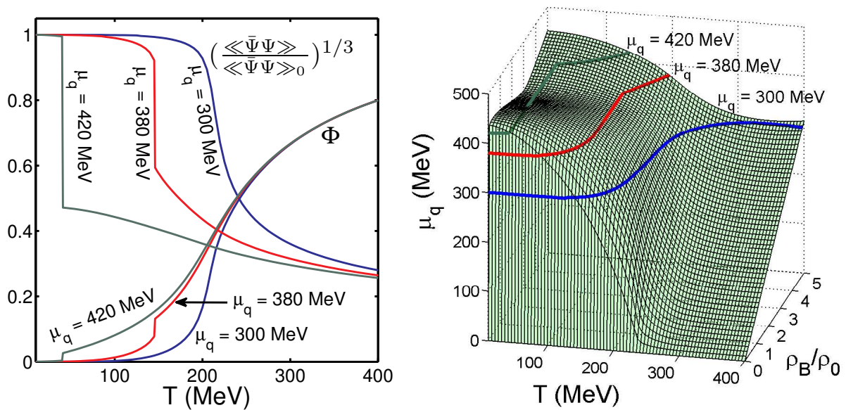
Figure 9. Etude des paramètres d'ordre pour plusieurs potentiels chimiques, et « trajectoires » associées dans le plan T - \rho_B .
