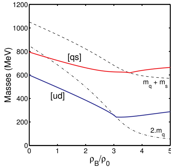
Figure 4. Masses des diquarks scalaires en fonction de la densité baryonique.
