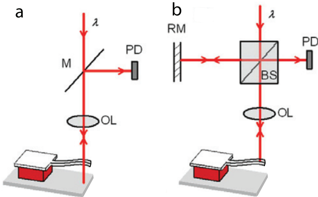
FIGURE 2.18: Deux dispositifs pour la détection interférométrique. a : Cavit  Fabry-P rot form e entre le r sonateur semi-transparent (NEMS ici doublement encastr ) et le substrat. L'intensit  lumineuse r fl chie est une fonction de l' paisseur de la cavit  et varie lorsque le r sonateur est en mouvement. Ce type de d tection est utilis  dans cette th se. b : Interf rom tre de Michelson : le faisceau lumineux r fl chi interf re avec un faisceau de r f rence cr e par un beam-splitter (BS) et un miroir de r f rence (RM). Figure issue de [143].
