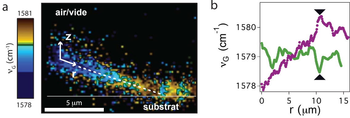
FIGURE 4.3: Contraintes mécaniques dans une membrane suspendue de graphène multicouche au repos. a : Cartographie Raman obtenue en microscopie confocale dans le plan (R, Z) . À chaque pixel est associé la fréquence de la bande G, en nombre d'onde. Les points noirs correspondent aux endroits où il n'y a pas de graphène multicouche. b : fréquence de la bande G le long de la membrane (●), et le long du même échantillon après effondrement sur le substrat de \text{SiO}_2 (●). Les marques noires représentent la position de la charnière.
