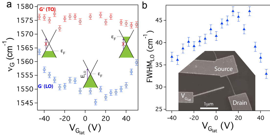
FIGURE 1.23: Modulation électrostatique du couplage électron-phonon dans un nanotube de carbone métallique. a : Evolution de la fréquence des modes LO (◐) et TO (◑) (bande G) d'un nanotube métallique au sein d'un petit faisceau dont le niveau de Fermi est modulé électrostatiquement par une grille latérale. Les trois schémas représentent la modulation du niveau de Fermi par rapport au point de Dirac (états occupés en vert). Les flèches représentent la possibilité (ou l'impossibilité) pour un électron de réaliser une transition interbande selon la position du niveau de Fermi. La longueur de ces flèches est égale à l'énergie du phonon en jeu (soit \sim 195 meV pour le mode LO). b : Evolution de la largeur à mi-hauteur ( FWHM_{LO} ) du mode Raman LO en fonction du potentiel de grille. L'encart montre une micrographie MEB du dispositif. Les électrodes de source et drain sont mises à la masse.
