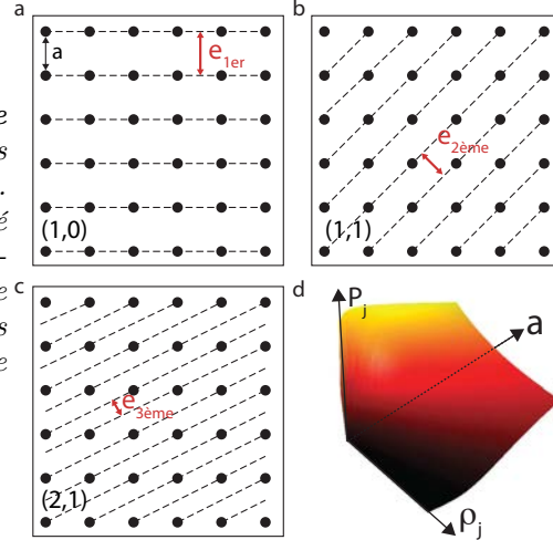
FIGURE 1.28: Configuration des plis du graphène dans un réseau carré de piliers. a-c : les lignes de plis (pointillées) relient les piliers (points) entre eux. L'espacement e_j entre deux lignes de plis est représenté en rouge. d : tracé de la probabilité P_j d'avoir un système de densité de plis \rho_j , en fonction du paramètre de maille a du réseau de piliers et de la densité de plis \rho_j (équation (1.21)). L'échelle de couleur est identique à l'axe P_j .
