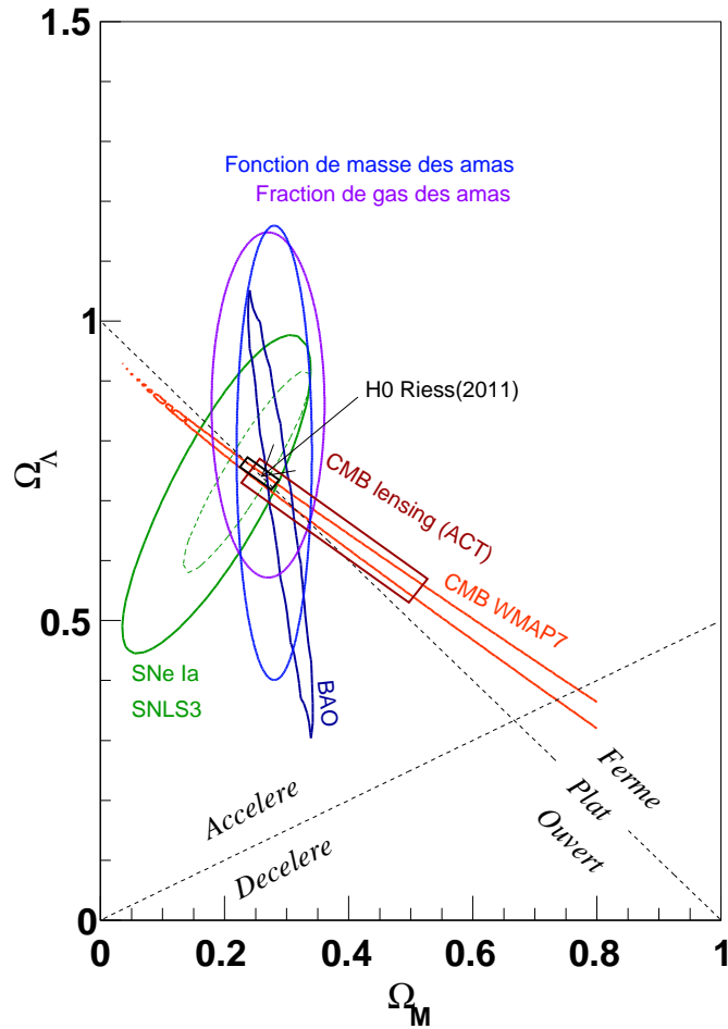
FIGURE 1.1 – Contours de confiance à 68% dans le plan \Omega_m \Omega_\Lambda pour les supernovae Ia (Conley et al. 2011) (contours tiretés : sans les incertitudes systématiques), les oscillations de baryon (Eisenstein et al. 2005; Beutler et al. 2011; Blake et al. 2011b; Sánchez et al. 2012), le CMB (Komatsu et al. 2011), et contours approximatifs pour la fraction de baryon (Allen et al. 2008) et la fonction de masse des amas observés en X (Vikhlinin et al. 2009). Sont aussi représentées les combinaisons de WMAP7 avec la mesure de H_0 par Riess et al. (2011) et les contraintes qu'apportent la détection du lensing du CMB (Sherwin et al. 2011).
