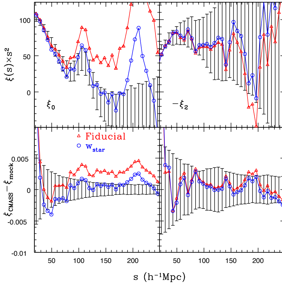
FIGURE 4.2 – Fonction de corrélation des galaxies BOSS (catalogue CMASS) en corrigeant (en bleu) ou en ne corrigeant pas (en rouge) de la perte d'efficacité dans les régions denses en étoiles. A gauche le monopôle, à droite le quadrupôle. En haut les données, en bas l'écart entre données et simulations (les barres d'erreur noires sont le RMS des simulations). On voit sur la figure en haut à gauche que la position du pic BAO n'est pas altérée par la correction en fonction de la densité d'étoiles. On voit aussi un deuxième pic significatif dans la fonction de corrélation à \simeq 200h^{-1} Mpc. Cette figure est tirée de Ross et al. (2012).
