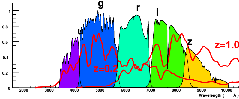
FIGURE 2.7 – Filtres de Megacam au CFHT et spectre d'une SN Ia au maximum de luminosité à z = 0.2 et z = 1 .
