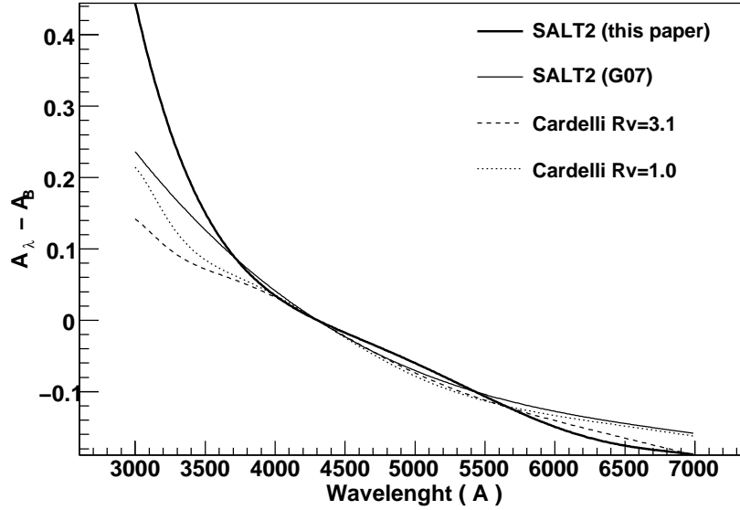
FIGURE 2.8 – Loi de couleur SALT2 comparée à la loi CCM pour différentes valeurs du paramètre R_V . Figure tirée de G10.
