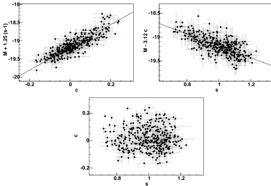
FIGURE 2.3 – Corrélations entre brillance, stretch et couleur de SNe Ia tirées de l’analyse des trois premières années du SNLS (comprenant des SNe proches et distantes). s est le paramètre “stretch” d’étirement ( s = 1.1 signifie une courbe de lumière 10% plus étirée que la moyenne), c est un paramètre de couleur, correspondant (en moyenne) à la couleur B - V au maximum de luminosité à une constante près. M est la magnitude absolue d’une SN moyenne (avec s = 1 et c = 0 ) en bande B pour h = 0.7 . Ces magnitudes absolues sont tirées des résidus à l’ajustement du diagramme de Hubble.
