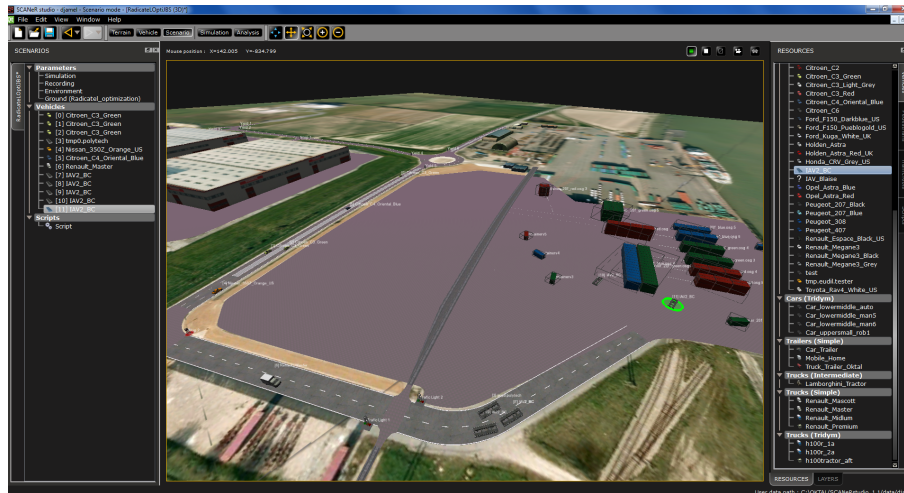
FIGURE 5.1 – Plate-forme de simulation routière SCANerStudio.
