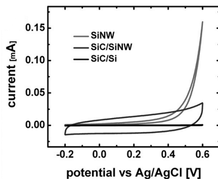
FIGURE 1.58 – Courbe Courant/potential pour un micro-super-capaciteur avec trois types d'électrodes différentes : nanofils de Si, nanofils de SiC et nanofils cœur-coquille Si-SiC. La montée brusque de la courbe pour l'électrode en nanofils de Si s'explique par l'oxydation du Si et donc la dégradation des performances de l'électrode. D'après [190].
