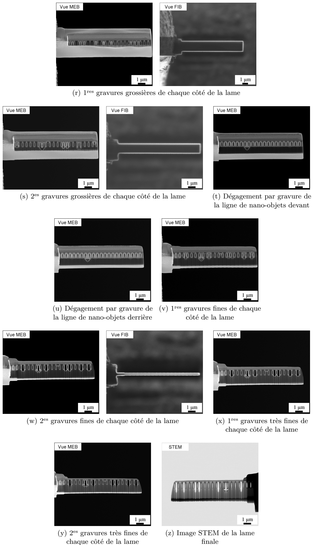
FIGURE 2.32 – (Fin) Images MEB et/ou FIB des différentes étapes de préparation d'une lame mince transversales de nano-objets.
