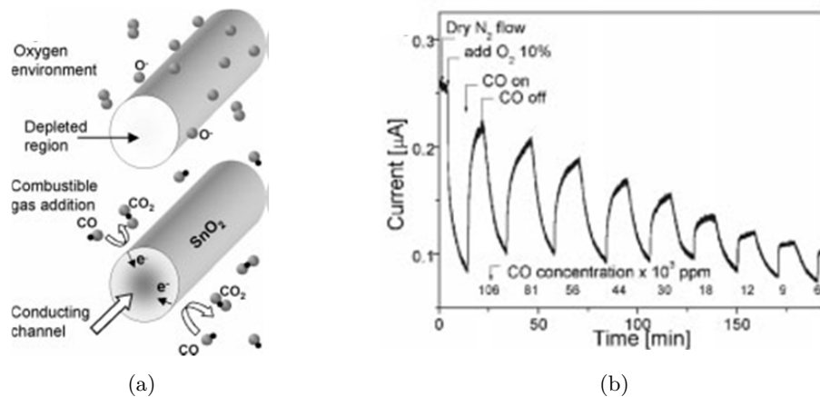
FIGURE 1.45 – (a) Représentation schématique d'un capteur de gaz (monoxyde de carbone) à base d'un transistor à nanofil de dioxyde d'étain. En environnement pur oxygène le transistor est fermé du fait d'une déplétion. Quand du CO approche de la surface la zone de déplétion disparaît et le courant augmente. (b) Courbe de réponse du capteur en fonction du temps. La réponse aux molécules de CO est bien identifiable, ainsi que le vieillissement du capteur au cours du temps. D'après [138].
