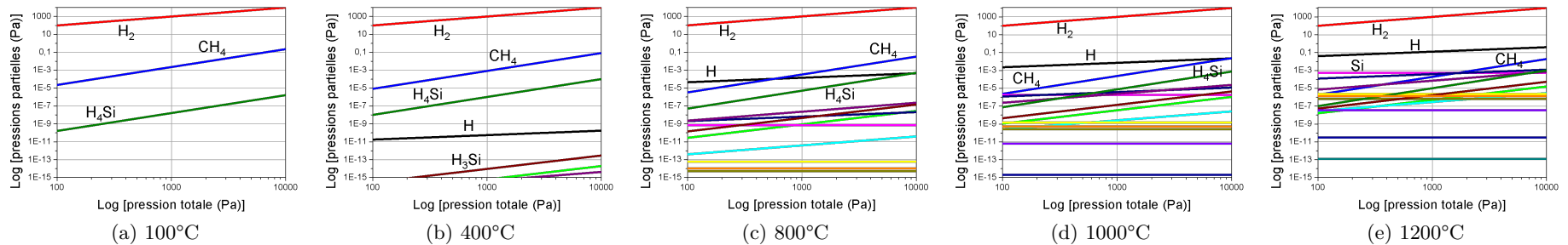
FIGURE 3.11 – Graphiques représentant les pressions partielles des 16 principaux gaz en équilibre avec les phases solides \langle\text{Si}\rangle et \langle\text{SiC}\rangle en fonction de la pression totale, pour différentes températures. Les échelles des abscisses et des ordonnées sont en log.
