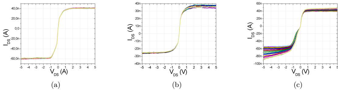
FIGURE 4.23 – Mesure du courant passant dans le drain pour différentes tensions imposées entre le drain et la source et pour une tension de grille V_G variant de -20 V à +20 V, pour les trois nano-transistors à nanofils cœur-coquille Si-SiC à grille face arrière. La légende des couleurs pour les différents V_G est présentée sur la figure 4.22.
