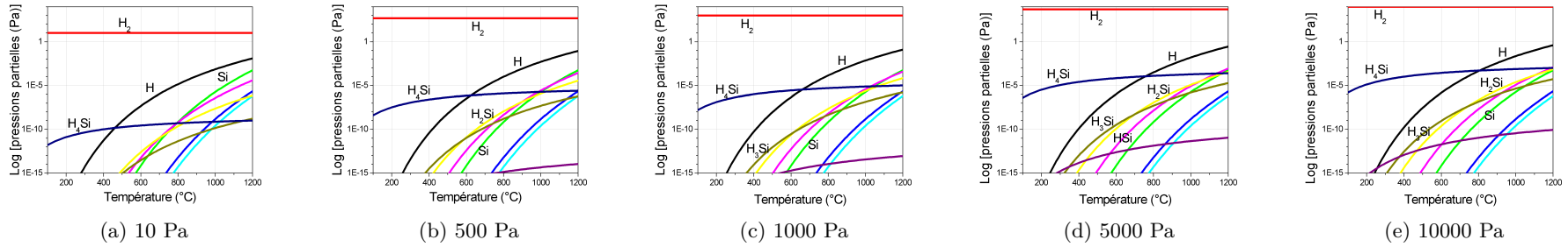
FIGURE 3.1 – Graphiques représentant les pressions partielles des 16 principaux gaz en équilibre avec la phase solide \langle\text{Si}\rangle et en fonction de la température, pour différentes pressions totales. Les échelles des ordonnées sont en log.
