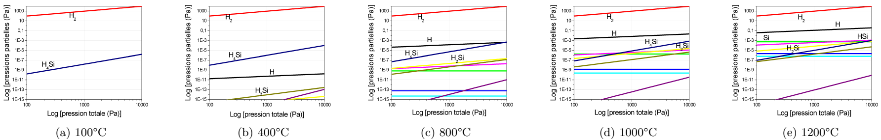
FIGURE 3.3 – Graphiques représentant les pressions partielles des 16 principaux gaz en équilibre avec la phase solide \langle\text{Si}\rangle en fonction de la pression totale, pour différentes températures. Les échelles des abscisses et des ordonnées sont en log.
