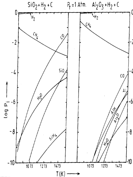
FIGURE 3.17 – Graphiques représentant les pressions partielles calculées des principales espèces gazeuses à l'équilibre en fonction de la température pour deux systèmes : \text{SiO}_2 + \text{H}_2 + \text{C} et \text{Al}_2\text{O}_3 + \text{H}_2 + \text{C} ; à 10^5 \text{ Pa} . D'après [10].
