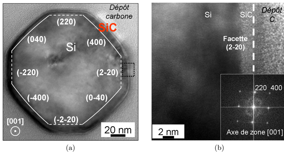
FIGURE 3.34 – (a) Image MET d'une rondelle de nanofil de Si carburé dans le bâti du LMI à 1150°C pendant 10 min. (b) Image MET haute résolution de la facette (220) de la rondelle où le cliché de diffraction révèle la présence de SiC monocristallin.
