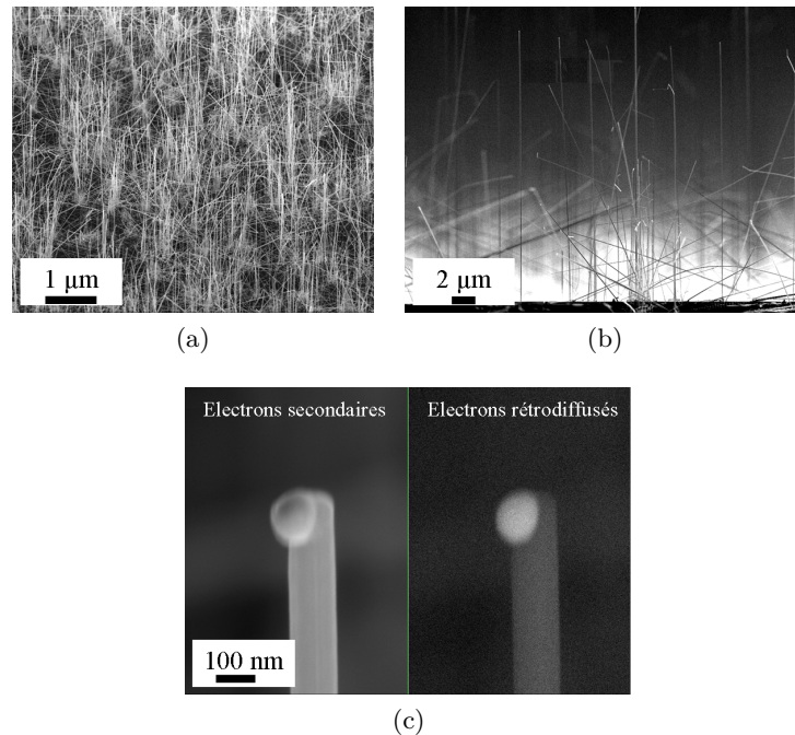
FIGURE 2.5 – Images MEB de nanofils de silicium longs ( \sim 20 \mu\text{m} ) obtenus par mécanisme VLS. (a) Vue générale à 25^\circ des nanofils de Si. (b) Vue à 90^\circ des nanofils de Si. (c) Zoom sur le haut d'un nanofil de Si où on aperçoit le catalyseur en or. On remarque le contraste chimique entre le catalyseur en or et le nanofil en silicium sur l'image en électrons rétrodiffusés.
