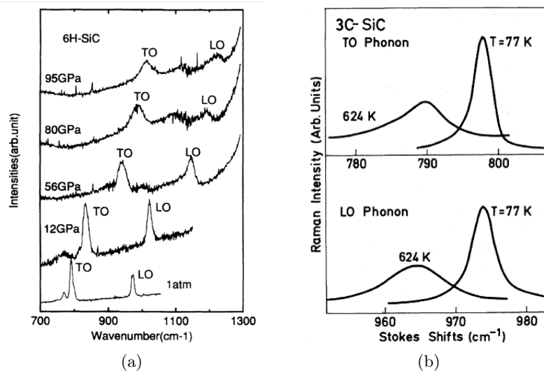
FIGURE 2.22 – (a) Spectres Raman d'un échantillon de 6H-SiC, placé dans un étai en diamant appliquant des contraintes successives sur l'échantillon. D'après [15]. (b) Spectres Raman des modes TO et LO du 3C-SiC observés à deux températures différentes (-196°C et 351°C) afin d'observer le décalage vers les faibles nombres d'ondes et l'élargissement des pics lors de l'augmentation de la température. D'après [11].
