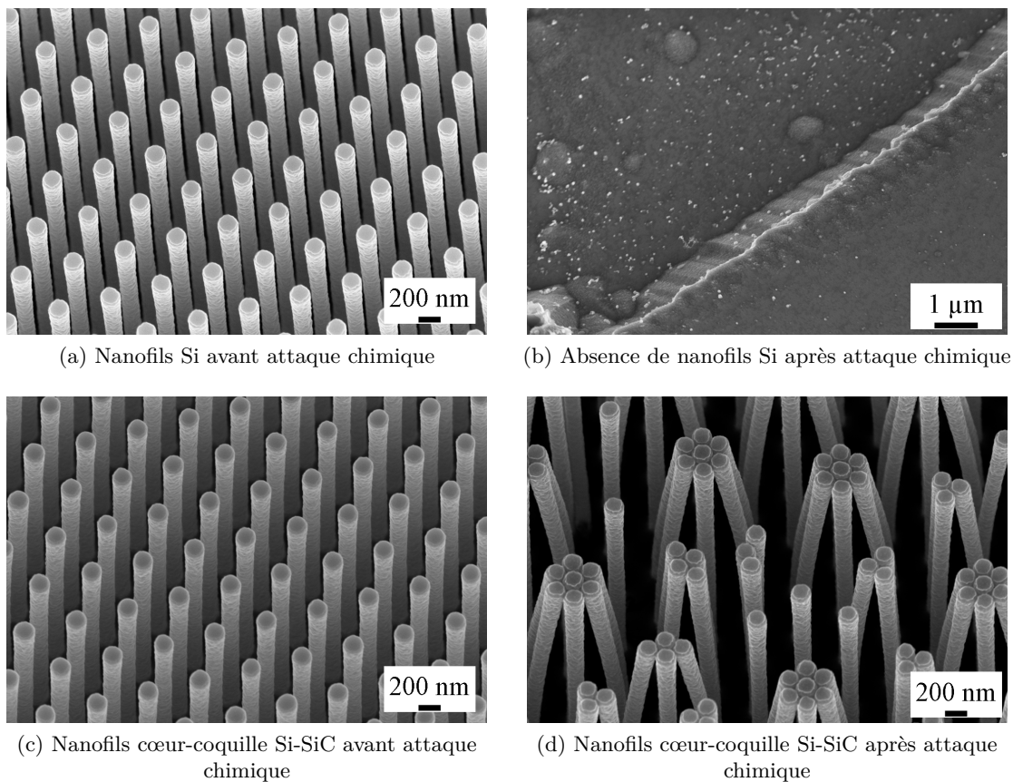
FIGURE 3.25 – Images MEB de : (a) nanofils de Si longs avant attaque chimique au KOH. (b) la zone après attaque chimique au KOH où se trouvaient les nanofils de Si. (c) nanofils de Si longs carburés avec un palier de 20 minutes à 1100°C, avant attaque chimique au KOH. (d) nanofils de Si longs carburés avec un palier de 20 minutes à 1100°C, après attaque chimique au KOH.
