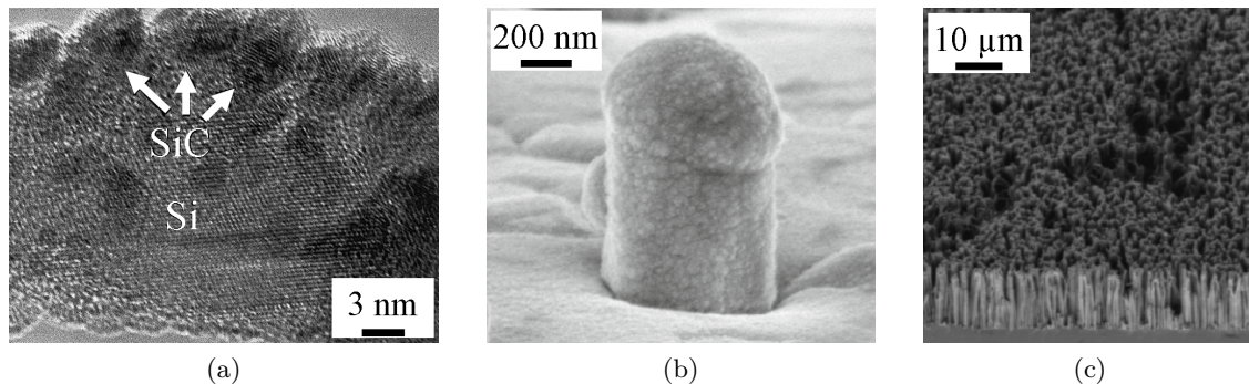
FIGURE 3.40 – (a) Image MET d'un nanofil cœur-coquille Si-SiC élaboré par X.T. Zhou et al. . (b) Image MEB d'un nanofil cœur-coquille Si-SiC obtenu par A.R. Beaber et al. . (c) Image MEB d'un réseau de nanofils cœur-coquille Si-SiC obtenus par J.P. Alper et al. . D'après [28–30].
