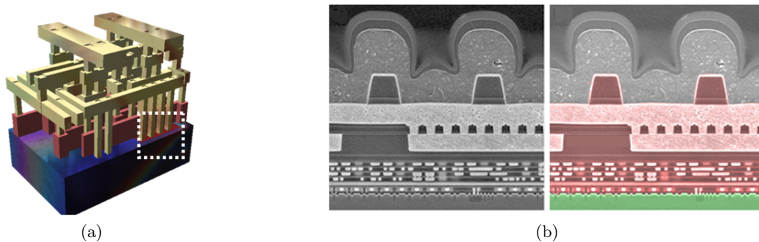
FIGURE 1.41 – (a) Représentation schématique d'un circuit intégré où le diélectrique a été enlevé. La partie entourée est agrandie à côté. (b) Images MEB originale et colorisée d'une coupe d'un circuit intégré A5 d'Apple utilisé dans l'iPad2 avec mise en évidence des zones front-end (en vert) et back-end (en rouge). Aucune échelle n'apparaît sur ces schémas, du fait du secret industriel qui entoure de tels objets. D'après [132].
