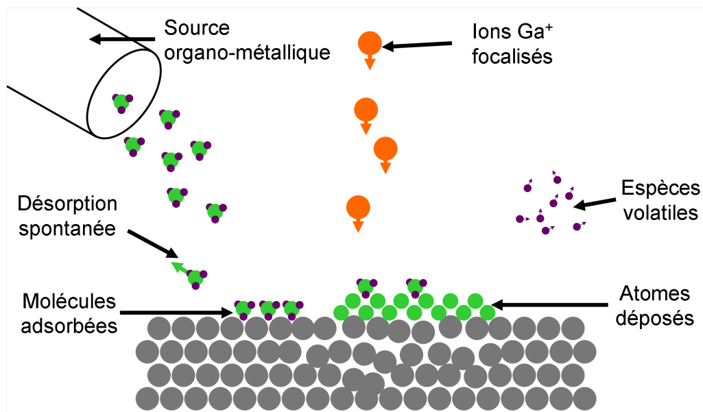
(b) Dépôt assisté par faisceau d'ions
