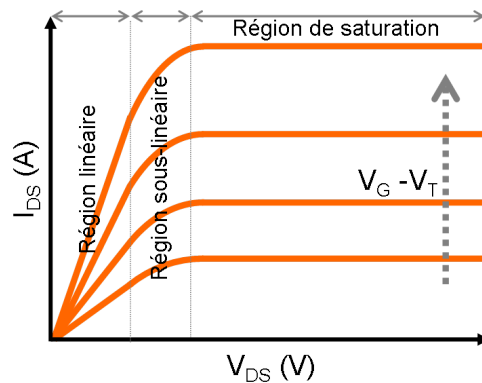
FIGURE 4.15 – Caractéristiques I_{DS} = f(V_{DS}) , pour différentes tension de grille, typiques d'un transistor à effet de champ. Trois régions sont distinguables : la région de linéarité, où le courant est proportionnel à la tension appliquée, la zone de saturation où quelle que soit la tension V_{DS} appliquée le courant I_{DS} est constant et la zone sous-linéaire qui correspond à la transition entre les deux précédentes.
