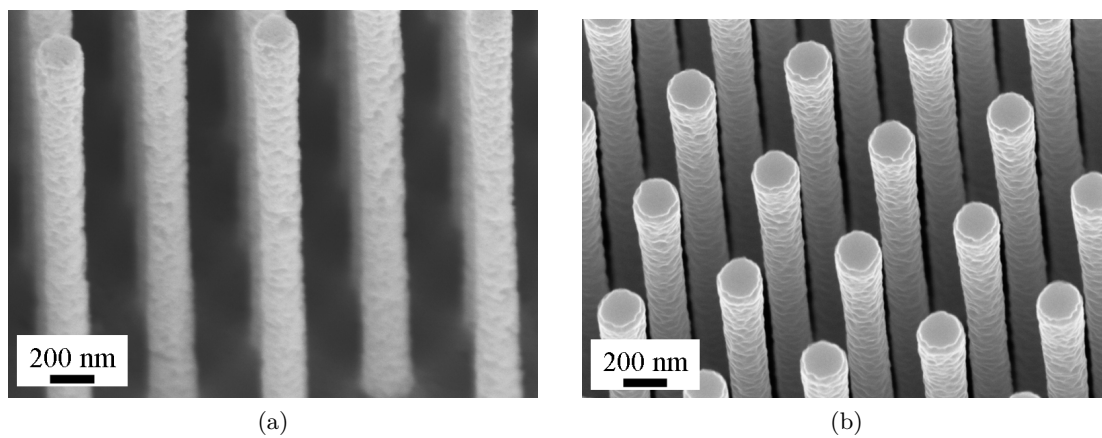
FIGURE 3.18 – Images MEB des nanofils de Si longs ayant subi une montée en température à 800°C sous flux de H_2 à une pression de 12 Pa : (a) dans un four en quartz nu. (b) Dans un four en quartz recouvert de silicium.
