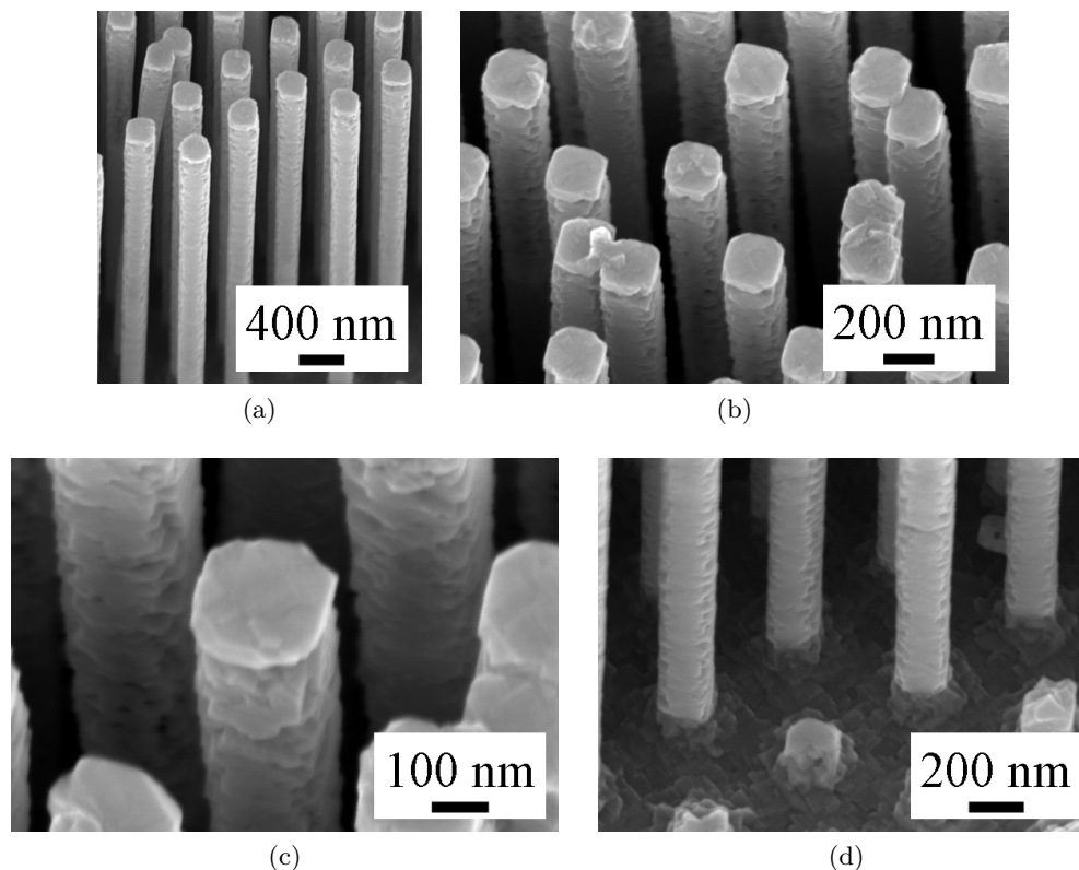
FIGURE 3.48 – Images MEB de nanotubes de SiC longs obtenus dans les conditions optimales des pressions P_1 et P_2 . (a) et (b) Vue générale à 25^\circ . (c) Zoom sur le haut des nanotubes de SiC. (d) Zoom sur le bas de plusieurs nanotubes de SiC.
