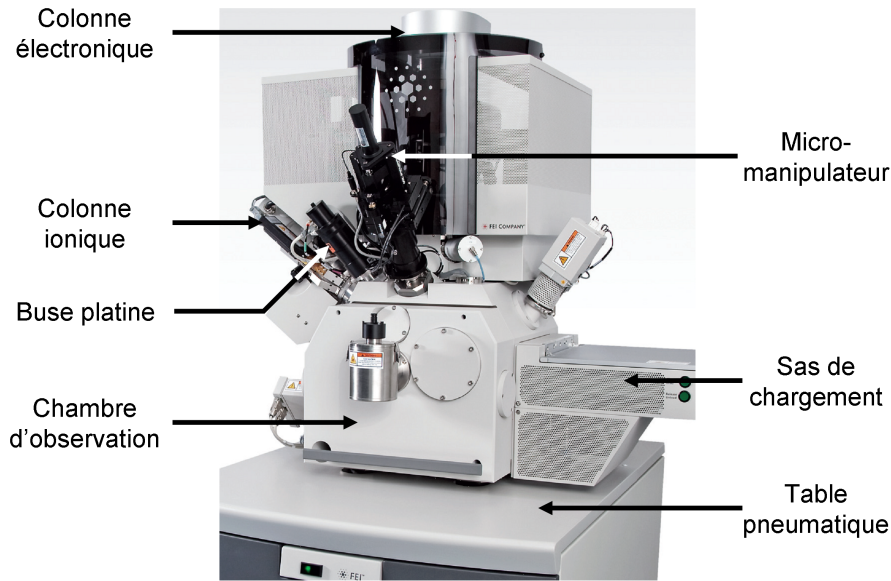
FIGURE 2.28 – Photographie du FIB/SEM Helios 450S de marque FEI avec indiqués les principaux organes le composant.
