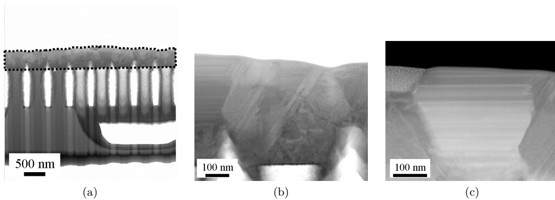
FIGURE 4.6 – (a) Image STEM en champ clair de la lame mince de type coupe transversale réalisée sur l'échantillon ayant une couche de SiC en surface. Cette couche est identifiée et mesure \sim 450 nm d'épaisseur. On peut constater que même le substrat de Si a été source d'atomes de Si pour la croissance de cette couche. (b) Zoom sur le haut d'un des anciens nanofils où un grain bien visible. (c) Image STEM en champ sombre où des défauts structuraux planaires sont visibles, ainsi qu'un contraste de grains.
