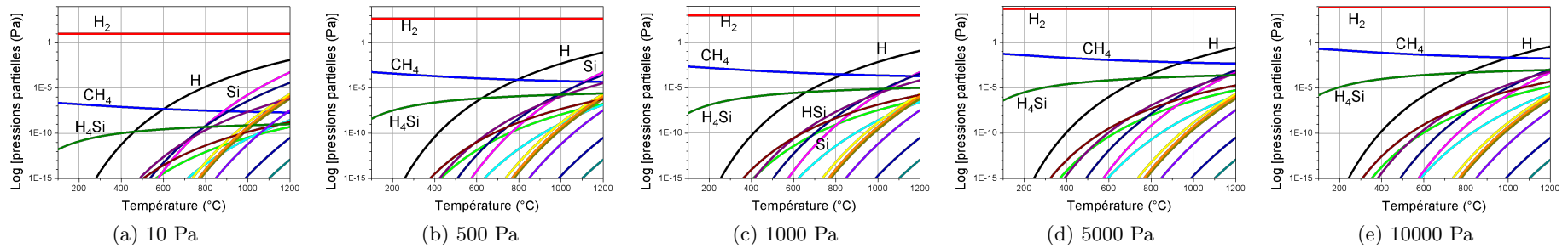
FIGURE 3.9 – Graphiques représentant les pressions partielles des 16 principaux gaz en équilibre avec les phases solides \langle\text{Si}\rangle et \langle\text{SiC}\rangle en fonction de la température, pour différentes pressions totales. Les échelles des ordonnées sont en log.
