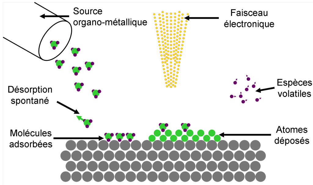
FIGURE 2.25 – Représentation schématique du dépôt assisté par faisceau électronique.
