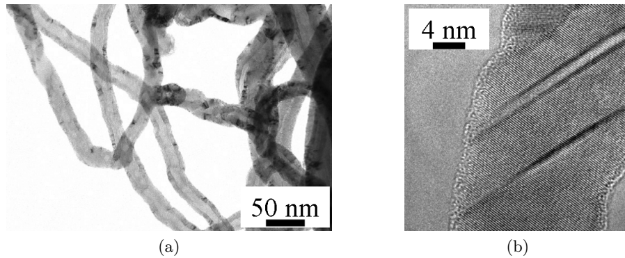
FIGURE 1.53 – (a) Image MET de nanotubes de SiC obtenus par réaction d'un gaz de SiO sur des nanotubes de carbone. (b) Image MET d'un nanofil de SiC obtenu par réaction d'un gaz de SiO sur des nanotubes de carbone pendant la même expérience. D'après [162].
