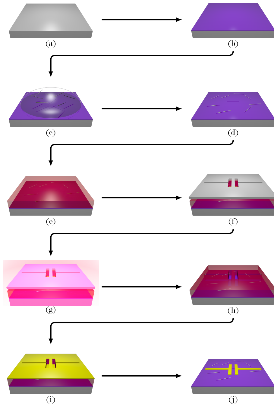
FIGURE 4.11 – Les principales étapes de fabrication d'un nano-transistor à effet de champ à canal nanostructure 1D : (a) Substrat de Si dégénéré p ++ . (b) Dépôt d'une couche de Si 3 N 4 faisant office d'oxyde de grille. (c) Dépôt d'une goutte d'isopropanol contenant des nanostructures 1D. (d) Évaporation de l'isopropanol pour déposer les nanostructures sur la surface. (e) Étalement d'une résine négative photosensible. (f) Alignement d'un masque de lithographie définissant le drain et la source. (g) Insolation par photolithographie. (h) Retrait, par un révélateur, de la résine insolée. (i) Dépôt des contacts par évaporation de Ni/Al. (j) Retrait par « lift-off » du métal déposé sur la résine.
