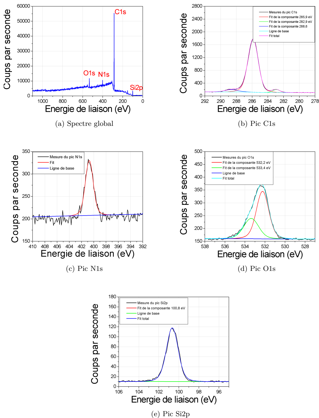
FIGURE 3.38 – Spectres XPS réalisés sur un échantillon plan de Si(100) ayant subi une carburation suivie d’une reprise d’épitaxie dans le bâti du LMI.
