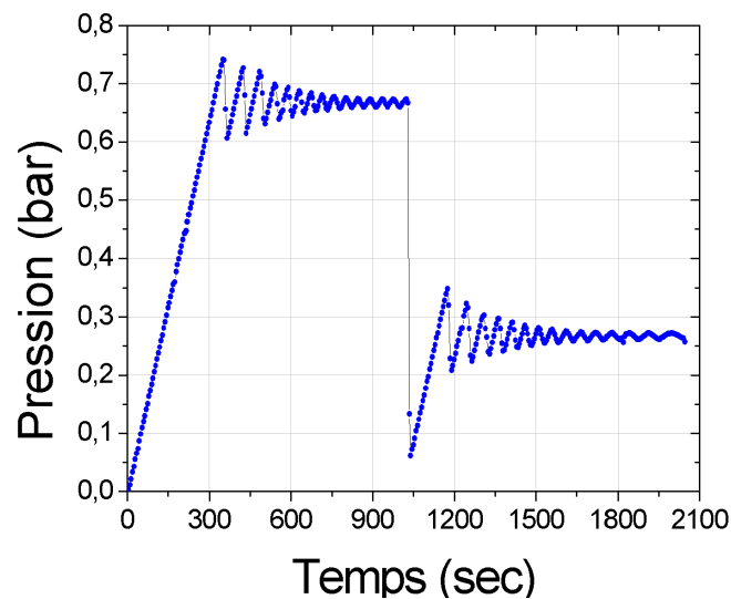
FIGURE 2.13 – Graphique représentant la valeur de la pression mesurée au cours du temps pendant un cycle de consigne 0 Pa \rightarrow 6,67 \times 10^4 Pa \rightarrow 2,67 \times 10^4 Pa.
