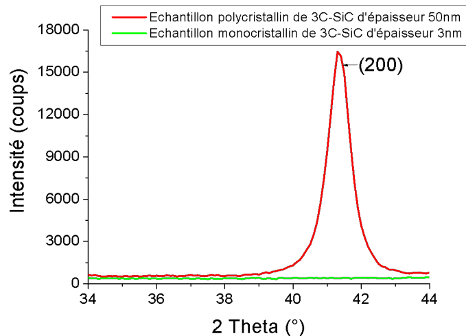
FIGURE 2.33 – Graphique où sont superposés deux diffractogrammes autour de la valeur de l’angle de diffraction des plans \{200\} du 3C–SiC : en rouge dans le cas d’une couche polycristalline de 50 nm d’épaisseur, en vert dans le cas d’une couche monocristalline de 3 nm d’épaisseur. Ces mesures ont été réalisées sur le diffractomètre du CMTC du campus.
