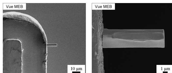
FIGURE 2.32 – (Suite) Images MEB et/ou FIB des différentes étapes de préparation d'une lame mince transversales de nano-objets.
