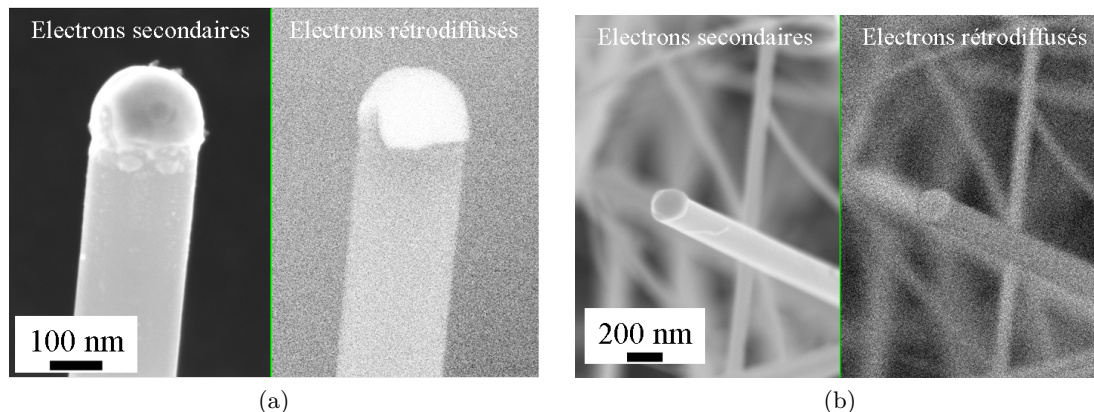
FIGURE 3.12 – (a) Image MEB —en électrons secondaires à gauche et en électrons rétrodiffusés à droite— de la tête d’un nanofil de Si obtenu par mécanisme VLS où le catalyseur d’or est visible. (b) Image MEB —en électrons secondaires à gauche et en électrons rétrodiffusés à droite— de la tête d’un nanofil de Si obtenu par mécanisme VLS où le catalyseur d’or a été éliminé par une solution de type IKI.
