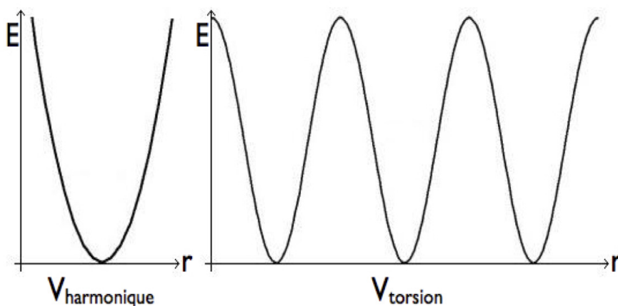
Figure 2.4 – Représentation des interactions liées
