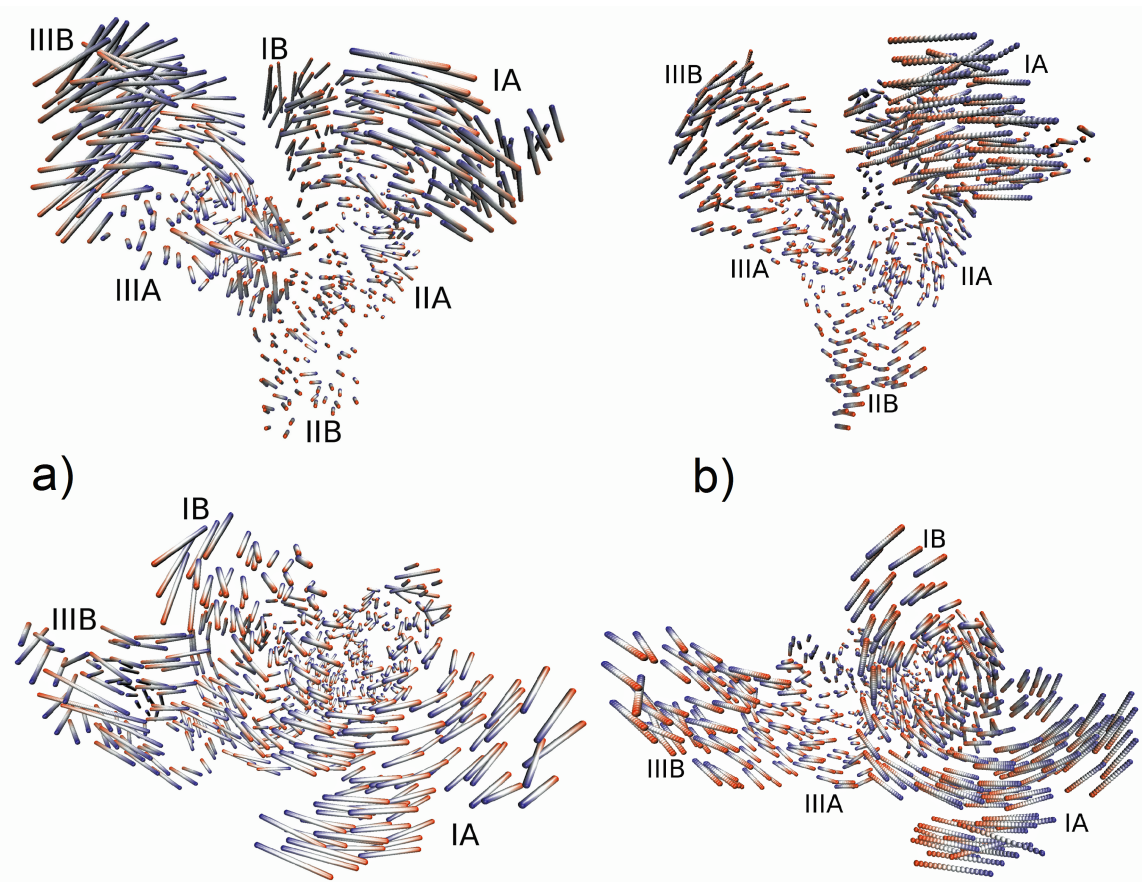
Figure 3.6 – Mouvement des atomes C_\alpha : a) entre les deux valeurs extrêmes de PC1 dérivé de traj1 (bleu pour le minimum, rouge pour le maximum) et b) au cours de la transition entre les conformations native et complexée avec le myristate (rouge pour la native, bleu pour le complexe HSA-myristate).
