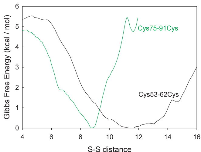
Figure 4.9 – Profils d'énergie libre de Gibbs calculés par rapport à la distance thiol-thiol pour les deux ponts réduits dans une conformation séparée.
