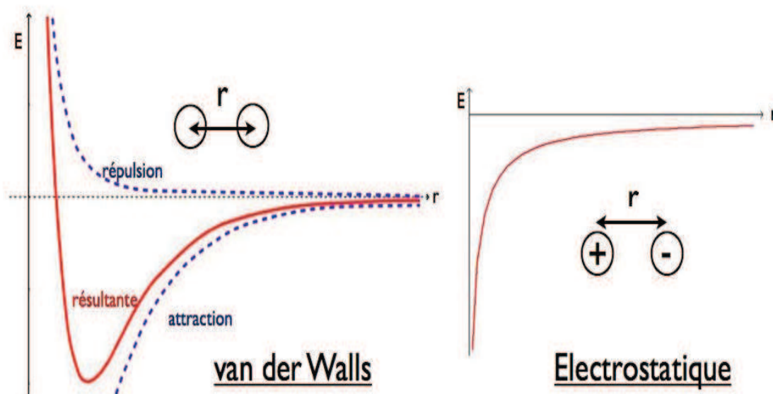
Figure 2.5 – Représentation des interactions non-liées
