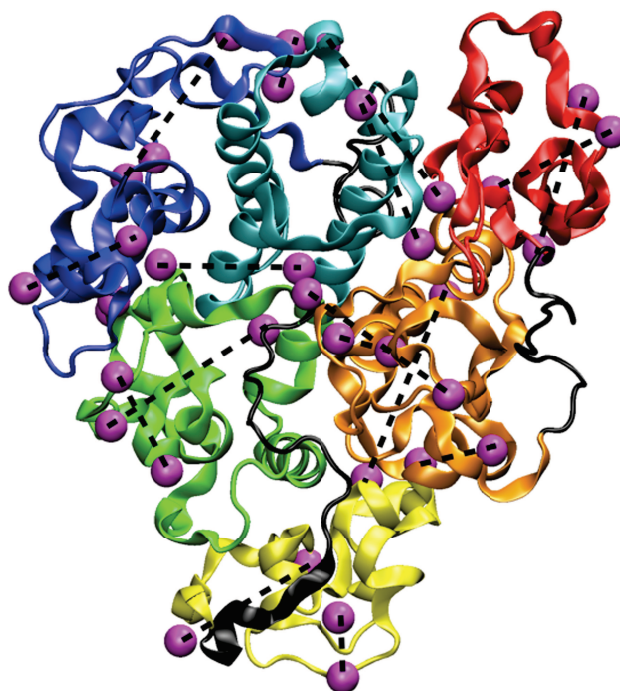
Figure 4.4 – Distorsion de la structure tertiaire de HSA (R) . La structure a été extraite de la trajectoire avec le champ de force OLPS-AA simulé à 500 K. Les atomes de soufre sont représentés par des sphères solides et sont connectés par des lignes pointillées lorsqu'ils appartenait au même pont réduit.
