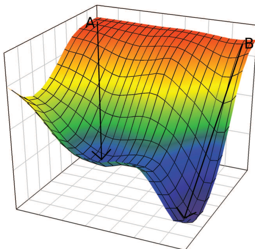
Figure 2.9 – Défaut de la méthode des gradients : le choix de la configuration initiale influe directement sur la position du minimum
