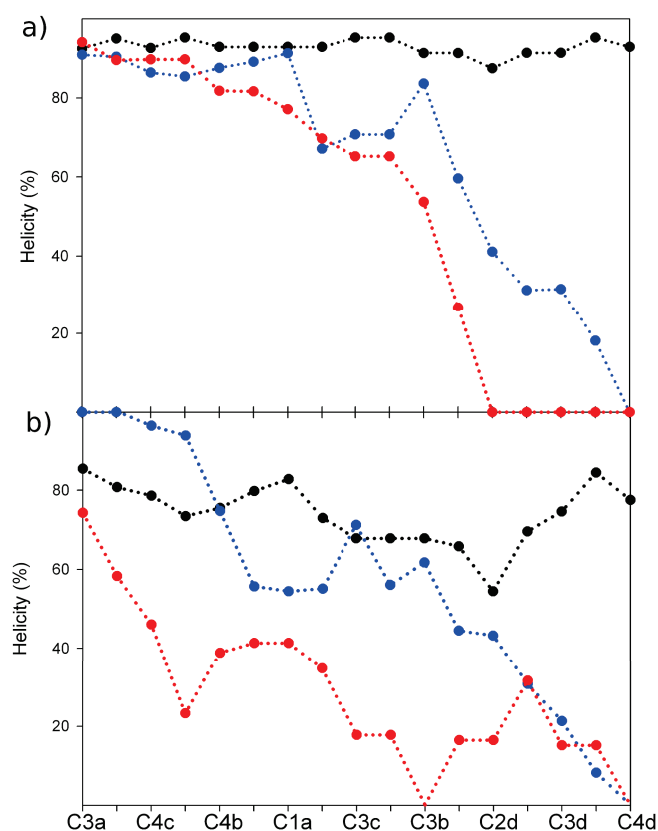
Figure 5.7 – Dépliage de trois hélices longues de type H2 (noir), H3 (bleu) et H4 (rouge) : a) dans le sous-domaine IA et b) dans le sous-domaine IIIB. Voir la Figure 1.2 pour l'emplacement des hélices.
