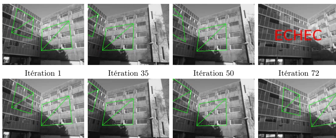
FIGURE 6 – Algorithmes de suivi dans des conditions variables. Au dessus : deux trackers mono-plans. En dessous : un tracker multiplans. L'algorithme basé sur un suivi de plan simple est perdu à l'itération 50.
