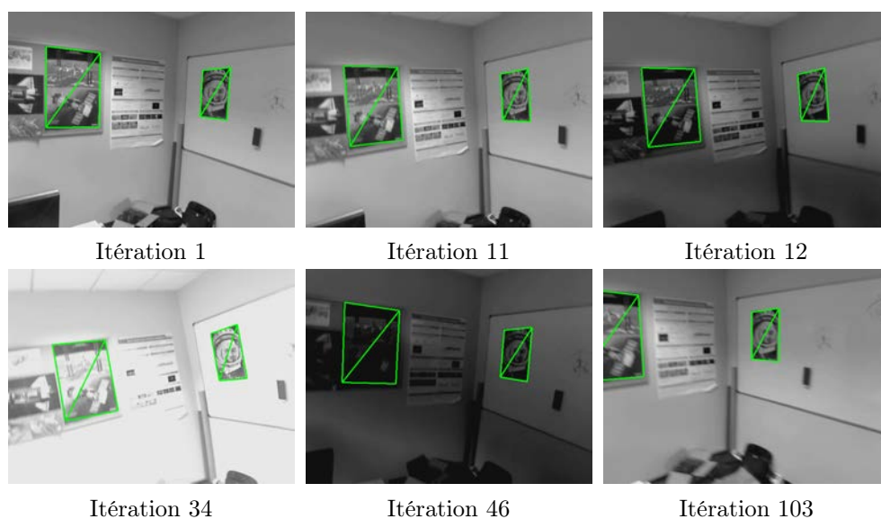
FIGURE 5 – Algorithmes de suivi dans des conditions variables. L'algorithme basé sur la SSD est perdu au premier changement brutal d'illumination à l'itération 12. L'algorithme proposé suit toujours le patch malgré les diminutions et augmentations brutales de luminosité (itérations 12, 34 et 46) ainsi que par de fortes conditions de flou (itération 103).
