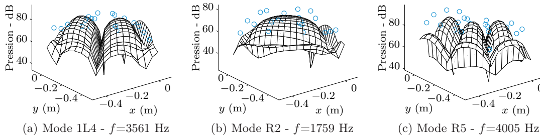
FIGURE 2.31 – Champ acoustique rayonné par la roue entre 180 et 270^\circ : modèle de plaque bafflée développée pour \mathcal{R}=0 (—) et mesures ( \circ )
