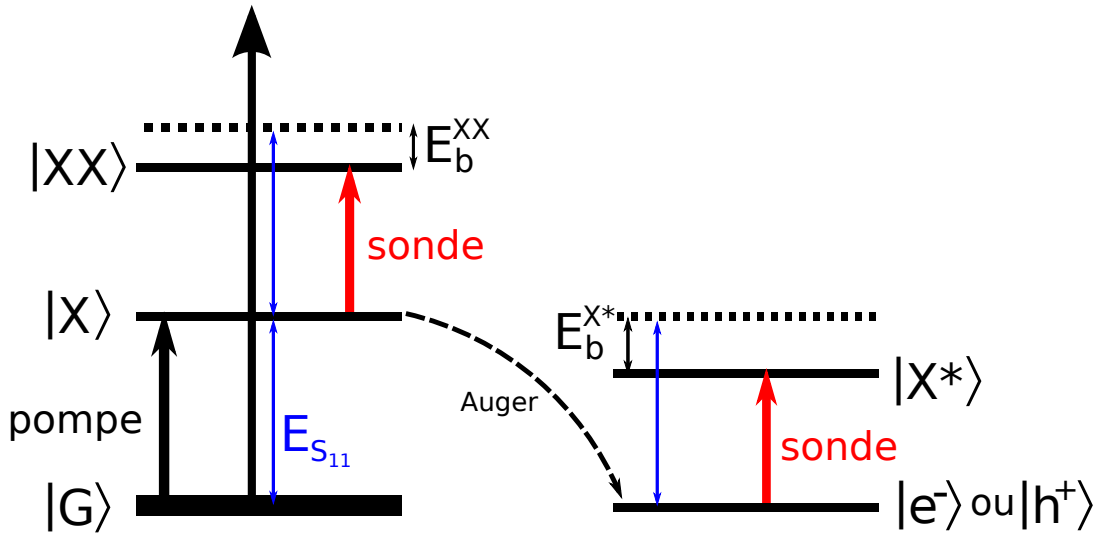
FIGURE 4.16 – Sch ema repr esentant les contributions   la photoabsorption de la formation de biexciton (XX)   partir d'un exciton (X), et de la formation d'un trion ( X^* )   partir d'une charge ( e ou h ) cr ee par dissociation d'un exciton.
