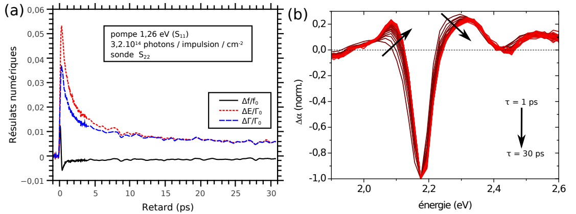
FIGURE 4.36 – (a) Dynamique de \Delta f/f_0 , \Delta E/\Gamma_0 et \Delta\Gamma/\Gamma_0 pour la transition S_{22} pour une pompe accordée sur S_{11} . (b) Spectres d'absorption transitoire normalisés correspondants, le pas entre deux spectres est de 1 ps.
