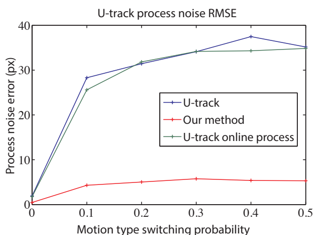
Figure 0.13: Erreurs d'estimation de la variance du bruit caractérisant le processus mesuré sur simulations en fonction de la probabilité de changement de type de transport (0 indique un déplacement purement Brownien confiné, 0.5 indique une chance sur deux de transiter vers un mouvement dirigé à chaque point de temps). Notre méthode (en rouge) est sept fois plus précise que l'estimateur u-track (en bleu). De plus, une simple estimation récursive de la variance, prenant en compte les mesures d'erreur issues du calcul à l'itération précédente, met en évidence l'intérêt de notre méthode basée sur l'algorithme u-track (en vert). L'adaptivité et l'agilité de l'algorithme de suivi sont assurées par la mise en place de plusieurs filtres.
