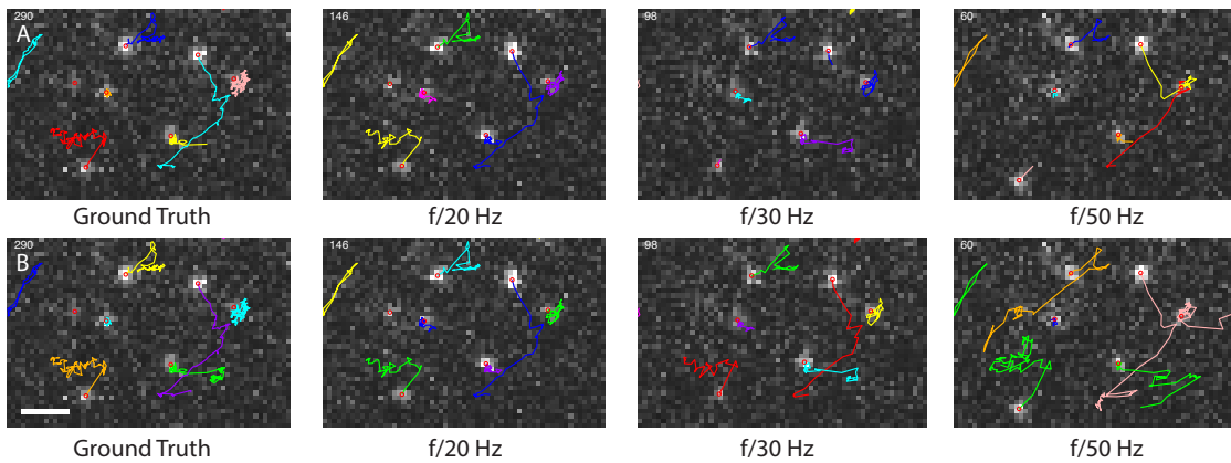
(b) u-track échoue à partir d'un facteur de décimation égal à 30 tandis que notre approche présente une seule erreur pour un facteur de décimation égal à 50 (les trajectoires les plus longues sont liées des fréquences faibles d'échantillonnage).
