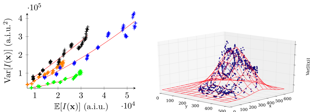
(a) Quatre gains quadratiques différents mesurés dans quatre régions différentes. Les croix d'intensité \lambda = 20000 \pm 10 a.i.u., tracées en noir, orange, bleu et vert, représentent les variances mesurées, les courbes rouges représentent la fonction (0.2) contrôlée par les paramètres estimés localement. (b) Variance locale mesurée pour une valeur d'intensité \lambda = 20000 \pm 10 a.i.u., tracée en bleu, fonction des positions spatiales. En théorie les variances mesurées devraient former un plan horizontal.
