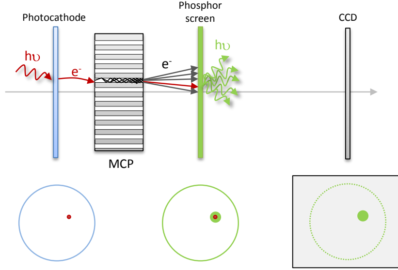
Figure 0.6: Processus de formation de l'image formation dans un CCD intensificateur de troisième génération.
