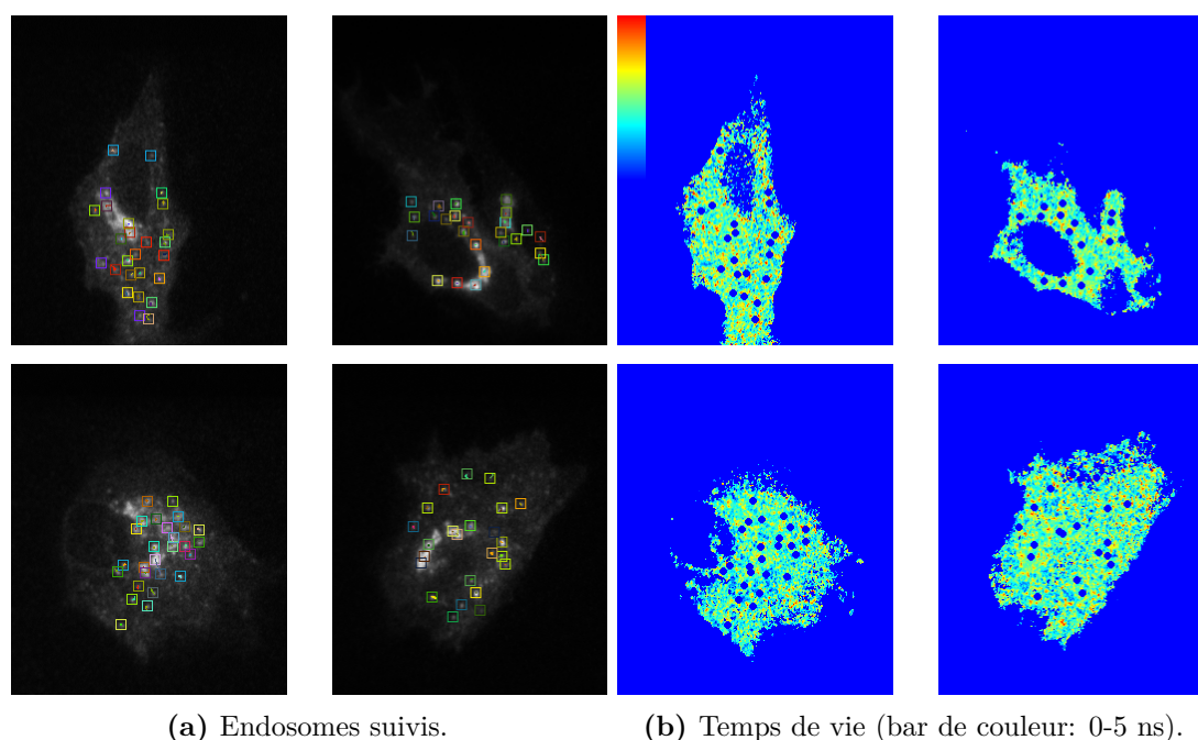
Figure 0.10: RX protéine marquée GFP sur les endosomes (gauche) et temps de vie à la membrane (droite) en l'absence d'accepteur.
