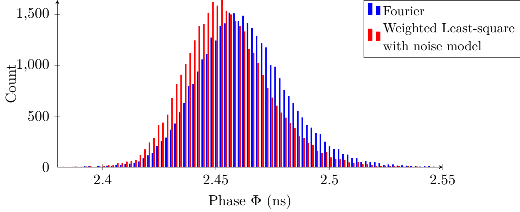
Figure 0.8: Histogrammes de phase comparant les résultats obtenus avec la méthode de Fourier et la méthode des moindres carrés pondérés par l’échelle du bruit estimée.
