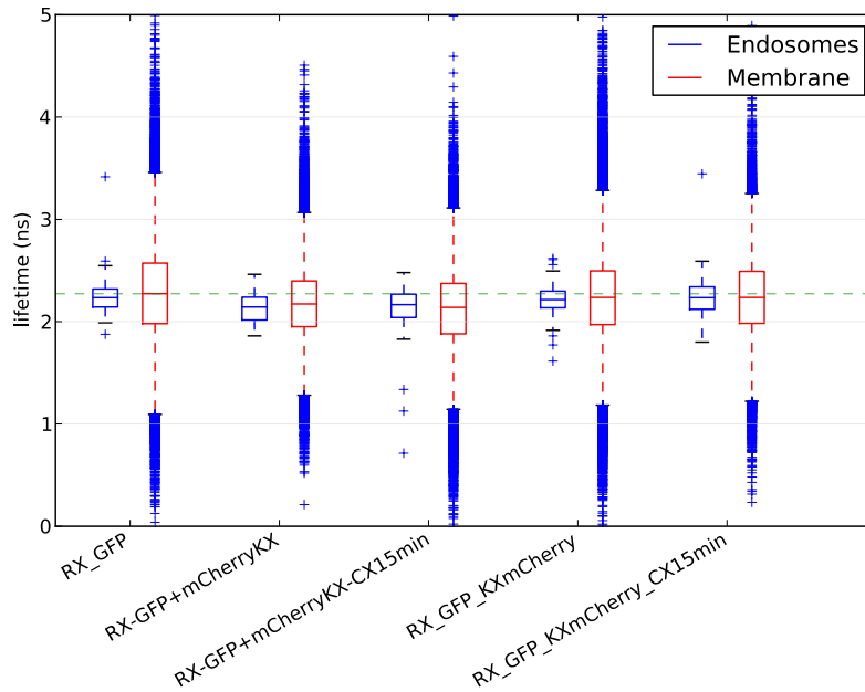
Figure 0.11: Distribution de temps de vie estimés au niveau des endosomes et à la membranes (voir détails Section 6.1 à la page 113).
