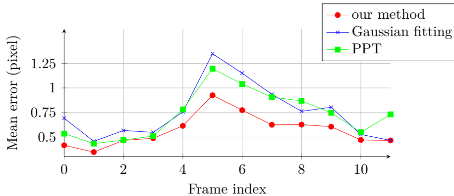
Figure 0.9: Erreurs moyennes de localisation. La méthode “Gaussian Fitting” [Anderson et al., 1992] est analogue à notre méthode, mais sans prise en compte de modèle d’intensité sinusoïdale. La méthode PPT est une méthode plus avancée combinant détection, puis calcul des trajectoires selon le principe du filtrage stochastique [Genovesio et al., 2006]. Les résultats sont obtenus sur des protéines RX marquées GFP et suivies manuellement (cellules épithéliales).
